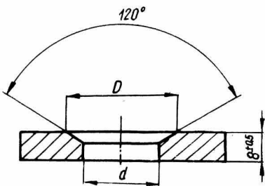
3.2. Wymiary podkładki stożkowej - wg rys. 2 i tabl.2.
