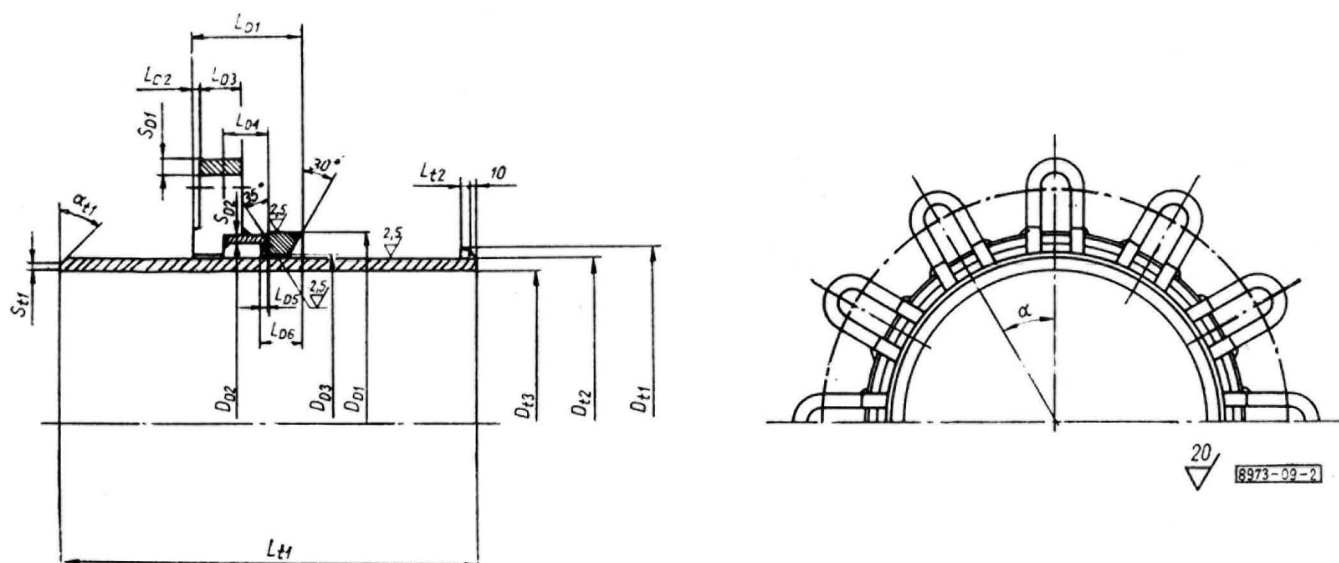
Rys. 2. Tuleja i dławik wydłużeń
