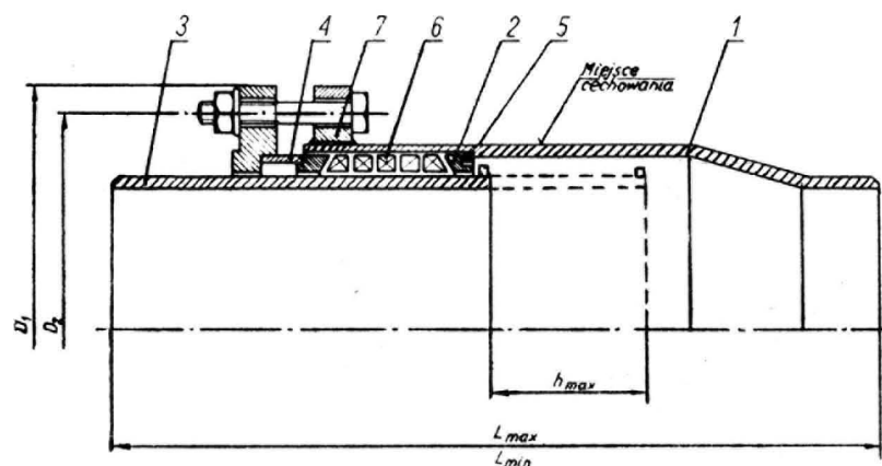
Rys. 1. Wydłużka dławicowa
