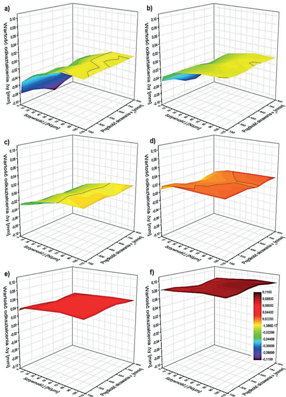
Rys. 6.11. Wartości odkształcenia w przekrojach środkowych ścianek nieutwardzonych o długości L_s=90\text{mm} wykonanych ze stopu EN AW-7075 narzędziem o sztywności j=2,0\text{ N}/\mu\text{m} ; grubości ścianek g: a) 4,0 mm, b) 2,8 mm, c) 2,0 mm, d) 1,4 mm, e) 1,0 mm, f) 0,7 mm
