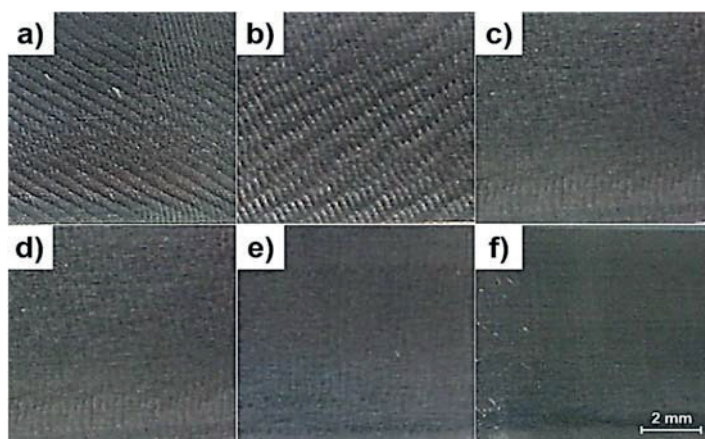
Rys. 6.29. Widok powierzchni ścianek nieutwardzonych o grubości g_s = 4 \text{ mm} , wykonanych ze stopu EN AW-7075, narzędziem o sztywności j = 72 \text{ N}/\mu\text{m} z różnymi prędkościami skrawania v_c : a) 150 m/min; b) 300 m/min; c) 450 m/min; d) 600 m/min; e) 750 m/min; f) 900 m/min
