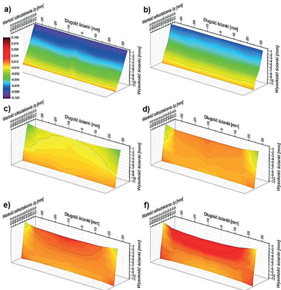
Rys. 6.22. Zarys powierzchni bocznej ścianek utwardzonych o długości L_s=90\text{mm} ; materiał EN AW-7075; prędkość skrawania v_c=600\text{m/min} ; sztywność narzędzia j=2,0\text{ N/}\mu\text{m} ; grubości ścianek g_s : a) 4,0 mm, b) 2,8 mm, c) 2,0 mm, d) 1,4 mm, e) 1,0 mm, f) 0,7 mm
