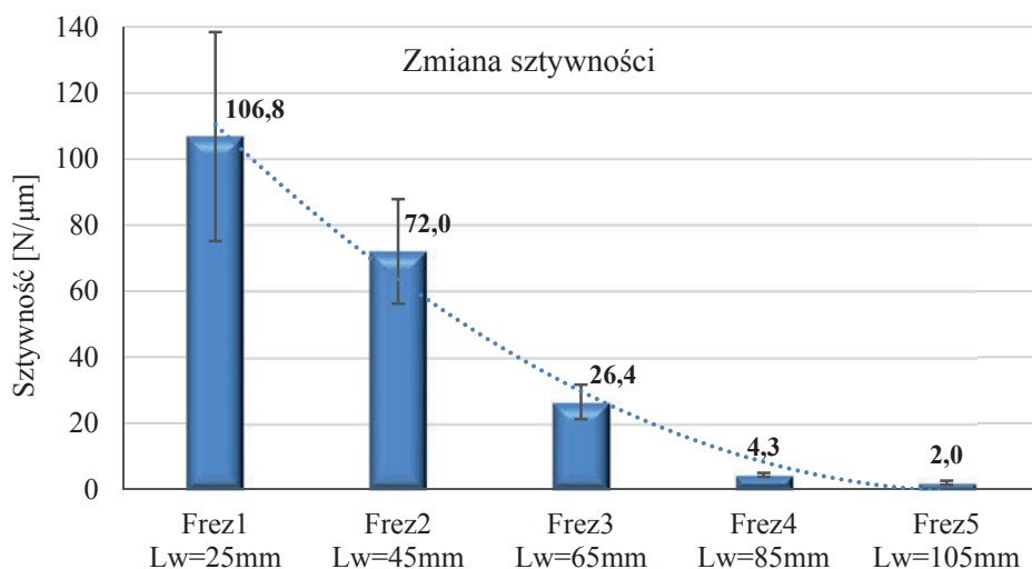
Rys. 4.2. Zmiana uśrednionej sztywności układu narzędzie–oprawka–wrzeciono w zależności od długości wysięgu narzędzia
