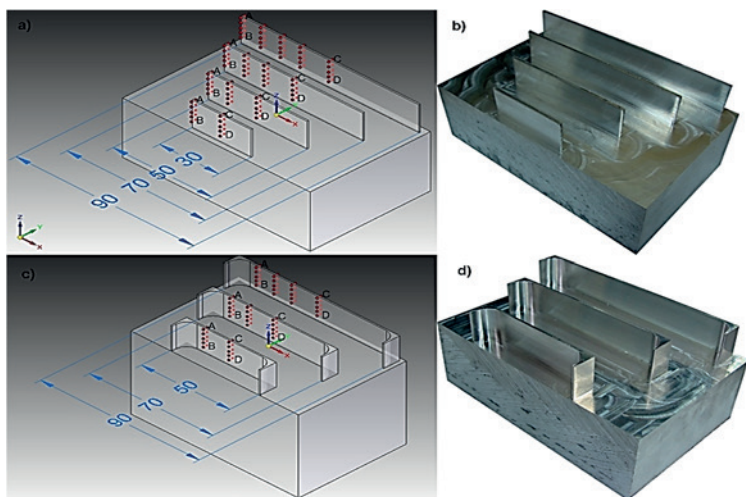
Rys. 3.2. Modele i widoki obróbianych próbek: a), b) próbki ze ściankami nieutwardzonymi; c), d) próbki ze ściankami utwardzonymi
