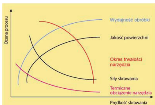
Rys. 1.9. Wpływ wzrostu prędkości skrawania na zmiany zjawisk towarzyszących procesowi obróbki [28, 71]
