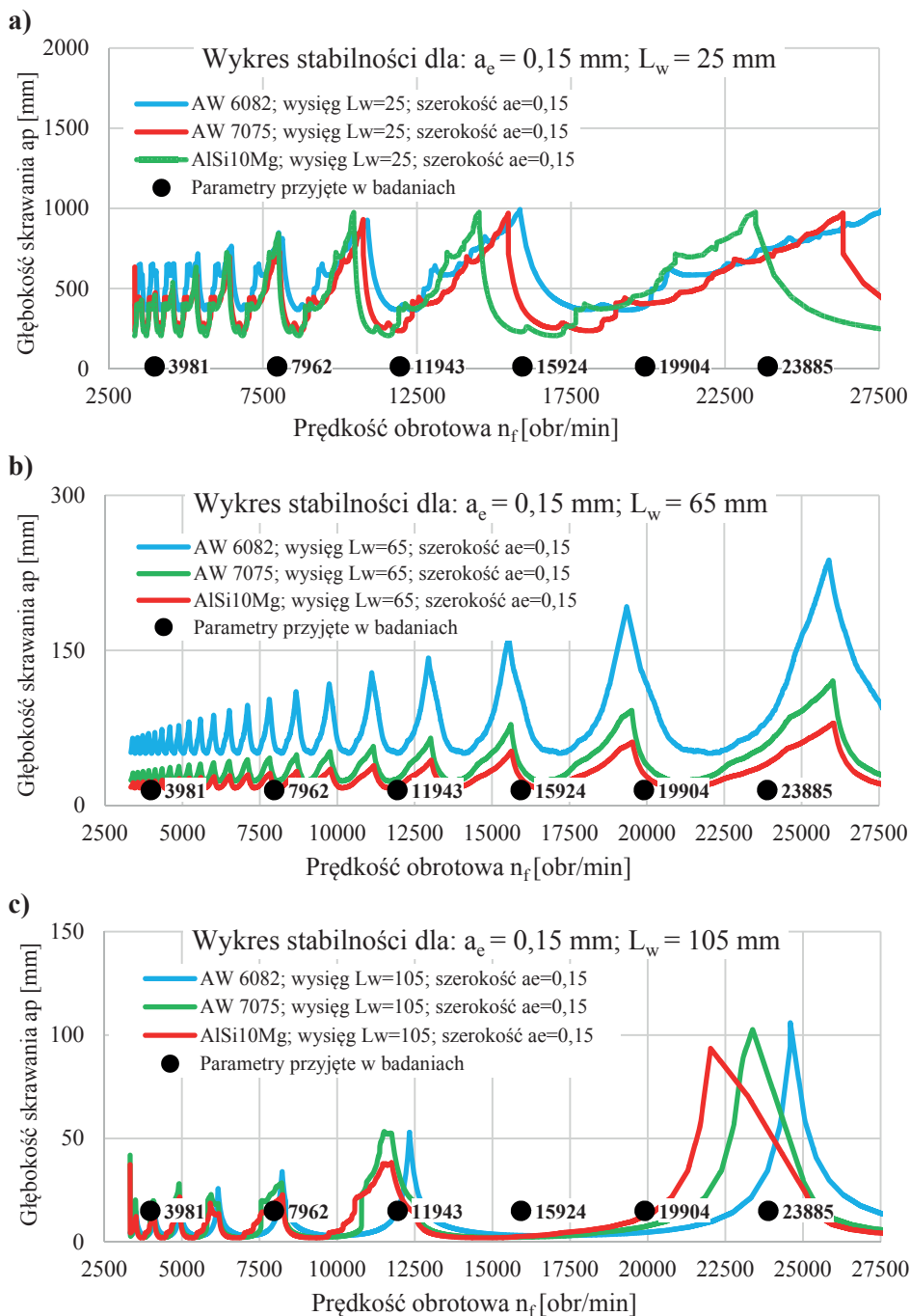
Rys. 4.4. Przykładowe wykresy stabilności dla głębokości skrawania a_p = 15 \text{ mm} i szerokości frezowania a_e = 0,15 \text{ mm} oraz różnych wysięgów narzędzia:
