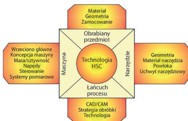
Rys. 1.7. Czynniki determinujące HSM [28]
