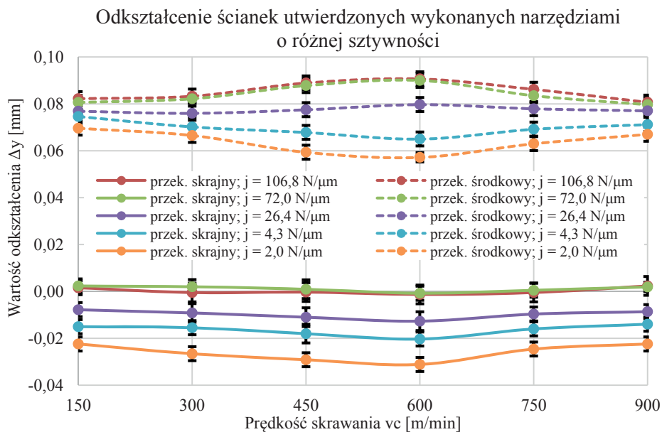
Rys. 6.16. Wartości odkształcenia w przekrojach skrajnych i środkowych ścianek utwardzonych o długości L_s=90\text{mm} i grubości g_s=0,7\text{mm} , wykonanych ze stopu EN AW-7075 z różnymi prędkościami skrawania
