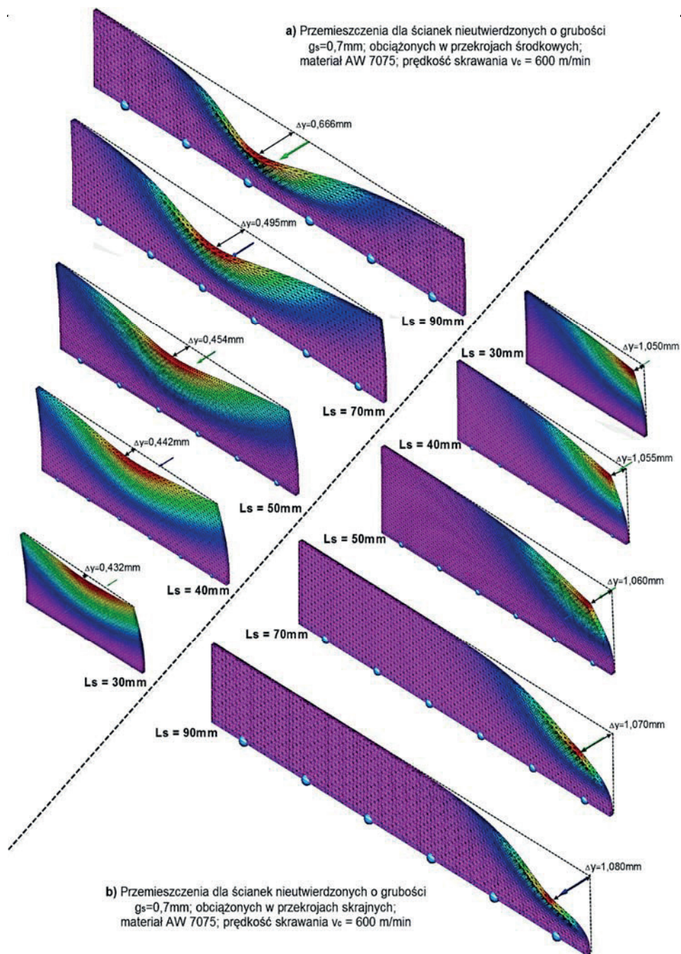
Rys. 5.6. Przemieszczenie wyliczone z zastosowaniem MES dla ścianek nieutwardzonych o różnych długościach i grubości g_s = 0,7\text{ mm} , dla stopu AW-7075 i obciążenia odpowiadającego sile skrawania przy prędkości v_c = 600\text{ m/min} , przyłożonego w przekrojach: a) środkowych, b) skrajnych
