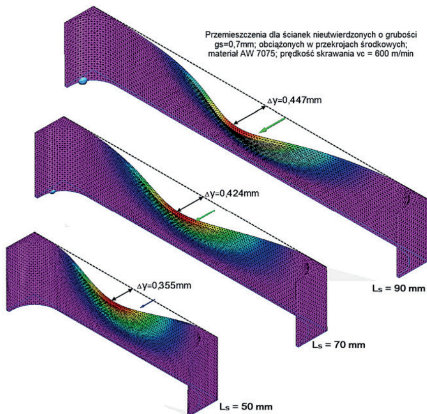
Rys. 5.7. Przemieszczenie wyliczone z zastosowaniem MES dla ścianek utwardzonych o różnych długościach i grubości g_s = 0,7 mm, dla stopu AW-7075 i obciążenia, odpowiadającego sile skrawania przy prędkości v_c = 600 m/min, przyłożonego w przekrojach środkowych
