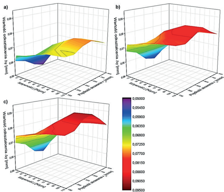
Rys. 6.27. Wartości odkształcenia w przekrojach środkowych ścianek utwardzonych o grubości g_s=0,7 mm wykonanych ze stopu EN AW-7075 narzędziem o sztywności j=2,0 N/ \mu m; długości ścianek: a) 50 mm, b) 70 mm, c) 90 mm
