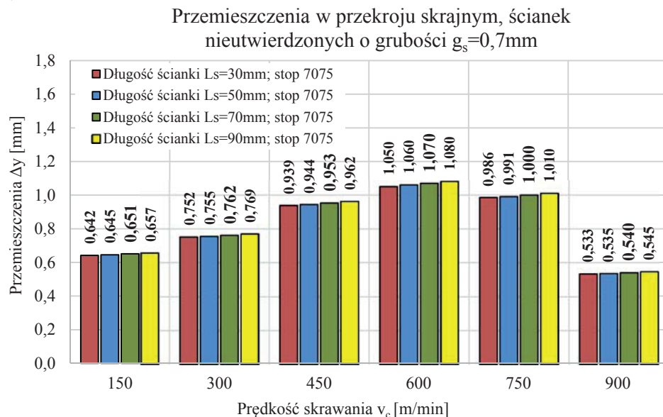
Rys. 5.11. Przemieszczenie ścianek nieutwardzonych o grubości g_s = 0,7 mm i różnych długościach L_s wykonanych ze stopu AW-7075, w przekrojach: a) środkowych, b) skrajnych
