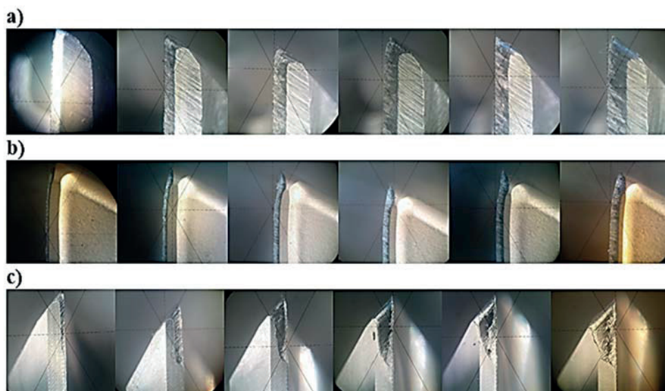
Rys. 1.16. Kolejne fazy zużycia ostrzy narzędzi: a) frez HSS, b) frez składany z płytką powlekaną \text{TiN} , c) frez węglkowy H10F [48]
