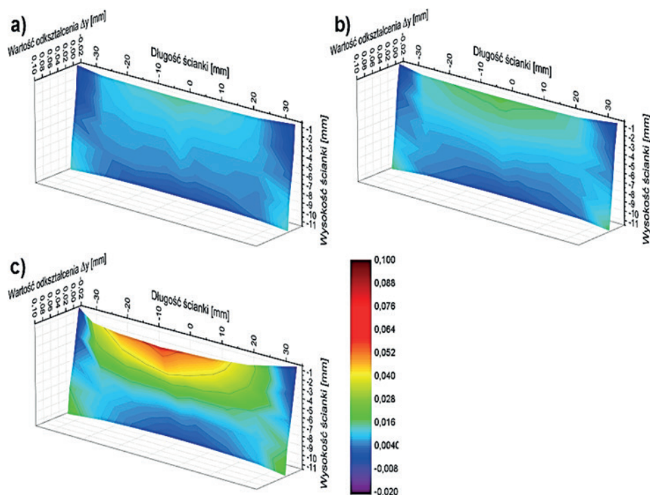
Rys. 6.19. Zarys powierzchni bocznej ścianek utwardzonych o długości L_s=90\text{mm} i grubości g_s=0,7\text{mm} ; prędkość skrawania v_c=600\text{m/min} ; sztywność narzędzia j=2,0\text{ N/}\mu\text{m} ; materiał: a) AlSi10Mg, b) EN AW-6082, c) EN AW-7075
