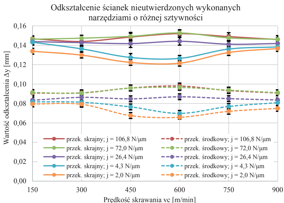
Rys. 6.2. Wartości odkształceń w przekrojach skrajnych i środkowych ścianek nieutwardzonych o długościach L_s=90 mm i grubościach g_s=0,7 mm, wykonanych ze stopu EN AW-7075 z różnymi prędkościami skrawania
