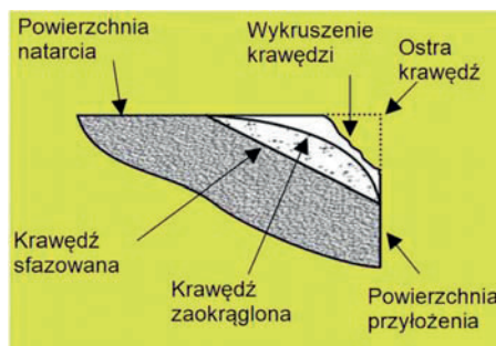
Rys. 1.10. Ukształtowanie krawędzi skrawającej narzędzia [13]
