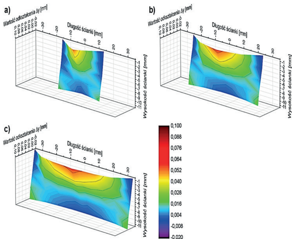
Rys. 6.25. Zarys powierzchni bocznej ścianek utwardzonych o grubości g_s=0,7\text{mm} ; materiał EN AW-7075; prędkość skrawania v_c=600\text{m/min} ; sztywność narzędzia j=2,0\text{ N}/\mu\text{m} ; długości ścianek L_s : a) 50 mm, b) 70 mm, c) 90 mm
