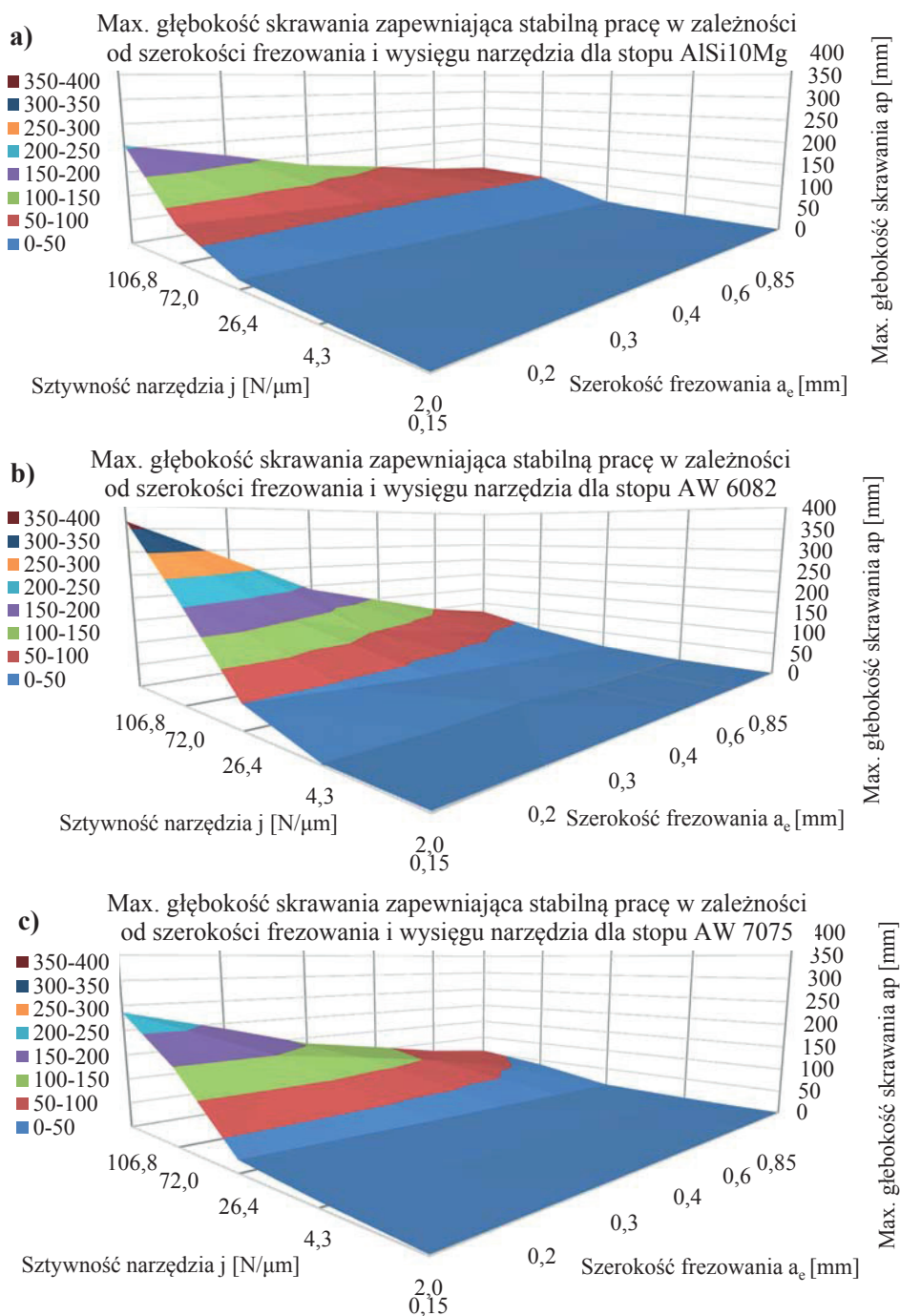
Rys. 4.5 Max. głębokość skrawania zapewniająca stabilną pracę w zależności od szerokości frezowania i wysięgu narzędzia dla stopu: a) AlSi10Mg, b) AW 6082, c) AW 7075
