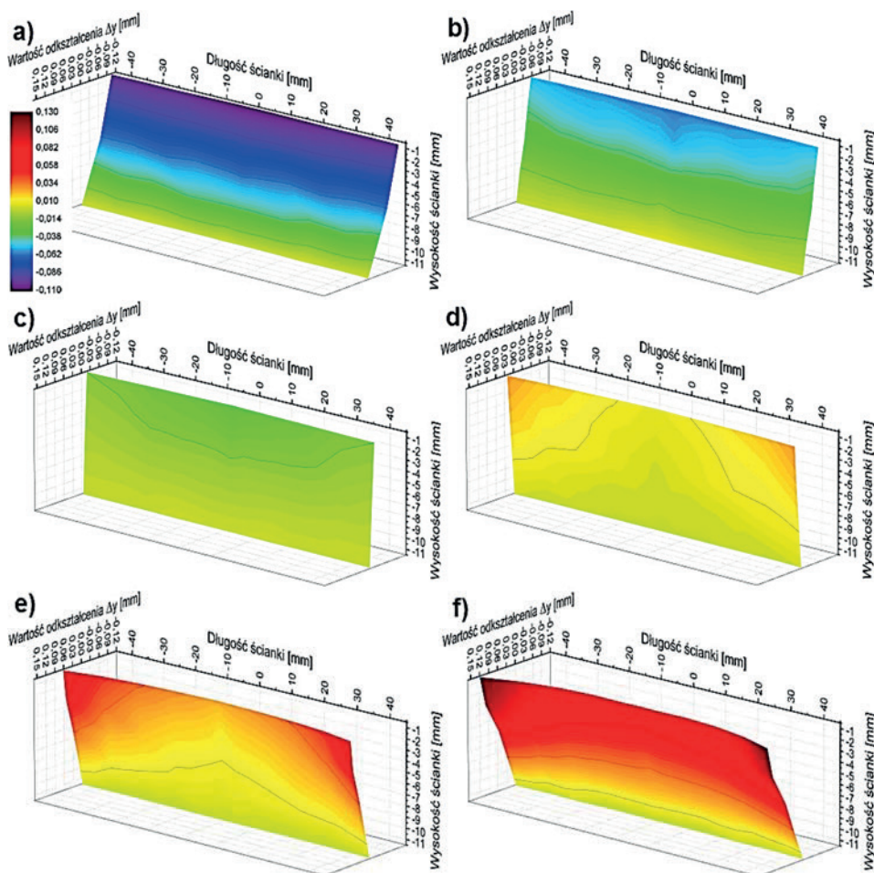
Rys. 6.9. Zarys powierzchni bocznej ścianek nieutwardzonych o długości L_s=90 mm; materiał EN AW-7075; prędkość skrawania v_c=600 m/min; sztywność narzędzia j=2,0 N/ \mu m; grubość ścianek g_s : a) 4,0 mm, b) 2,8 mm, c) 2,0 mm, d) 1,4 mm, e) 1,0 mm, f) 0,7 mm
