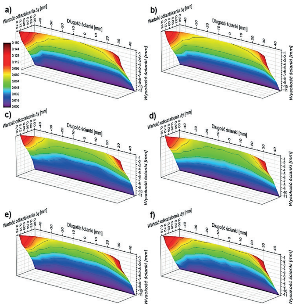
Rys. 6.1. Zarys powierzchni bocznej ścianek nieutwardzonych o długości L_s=90 mm i grubości g_s=0,7 mm; materiał EN AW-7075; sztywność narzędzia j=2,0 N/ \mu m; prędkości skrawania v_c : a) 150 m/min, b) 300 m/min, c) 450 m/min, d) 600 m/min, e) 750 m/min, f) 900 m/min
