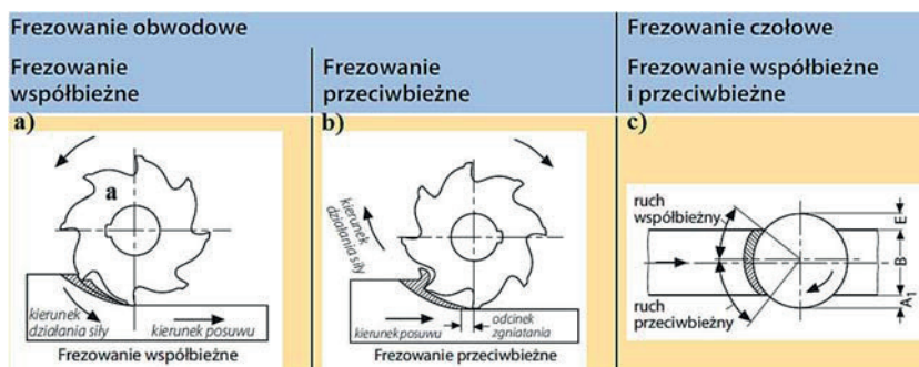
Rys. 1.2. Rodzaje frezowania [28]
