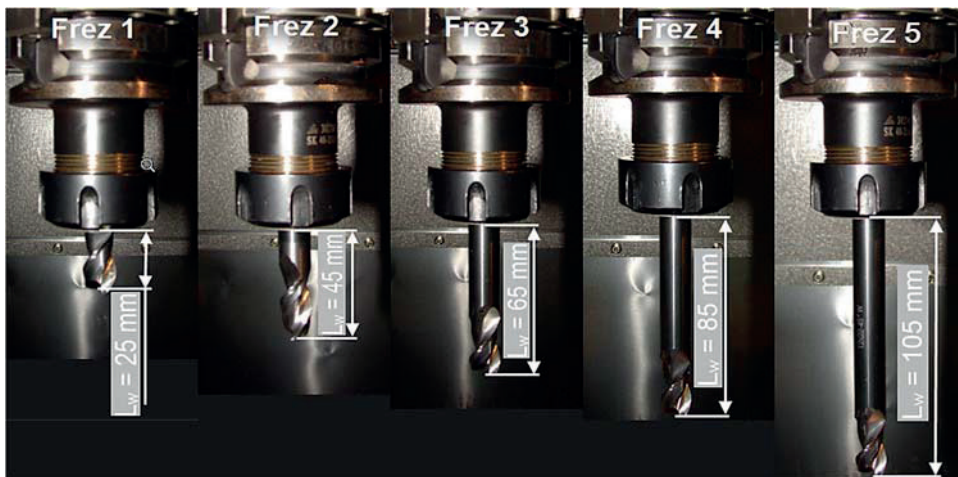
Rys. 3.4. Widoki narzędzi o różnej długości wysięgów zamocowanych we wrzecionie obrabiarki
