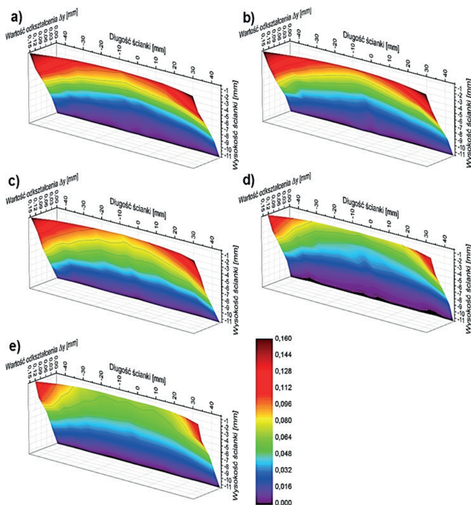
Rys. 6.3. Zarys powierzchni bocznej ścianek nieutwardzonych o długości L_s=90\text{ mm} i grubości g_s=0,7\text{ mm} ; materiał EN AW-7075; prędkość skrawania v_c=600\text{ m/min} ; sztywność narzędzi j: a) 106,8\text{ N}/\mu\text{m} , b) 72\text{ N}/\mu\text{m} , c) 26,4\text{ N}/\mu\text{m} , d) 4,3\text{ N}/\mu\text{m} , e) 2,0\text{ N}/\mu\text{m}
