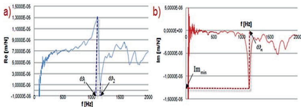
Rys. 1.24. Przykładowa odpowiedź układu narzędzie-oprawka-wrzeciono na wymuszenie a) część rzeczywista, b) część urojona [76]
