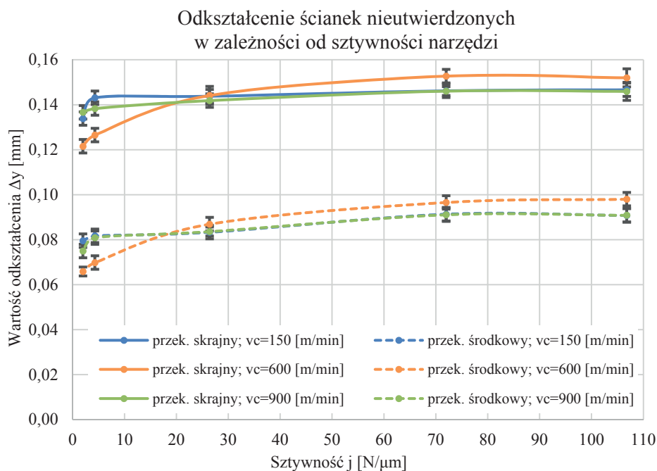
Rys. 6.5. Wartości odkształcenia w przekrojach skrajnych i środkowych ścianek nieutwierdzonych o długości L_s=90 mm i grubości g_s=0,7 mm, wykonanych ze stopu EN AW-7075 narzędziami o różnej sztywności
