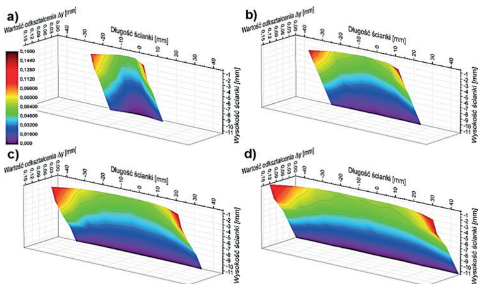
Rys. 6.12. Zarys powierzchni bocznej ścianek nieutwardzonych o grubości g_s=0,7 mm; materiał EN AW-7075; prędkość skrawania v_c=600 m/min; sztywność narzędzia j=2,0 N/ \mu m; długości ścianek L_s : a) 30 mm, b) 50 mm, c) 70 mm, d) 90 mm
