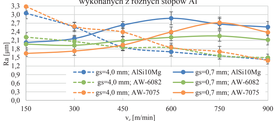
Rys. 6.31. Chropowość powierzchni ścianek nieutwardzonych o grubościach g_s=4,0 \text{ mm} i g_s=0,7 \text{ mm} , wykonanych z różnych stopów Al narzędziami o sztywnościach j : a) 106,8 \text{ N}/\mu\text{m} ; b) 2,0 \text{ N}/\mu\text{m}
