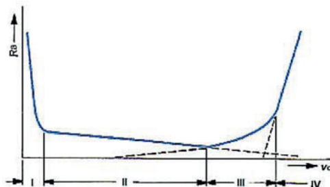
Rys. 1.14. Zależność parametru Ra od prędkości skrawania v_c [41, 69]
