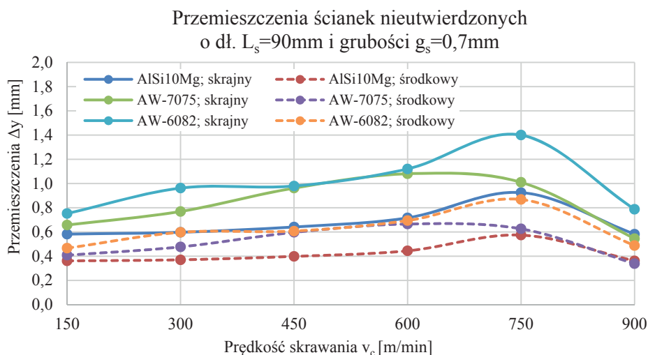
Rys. 5.10. Przemieszczenie w przekrojach środkowych i skrajnych ścianek nieutwardzonych
