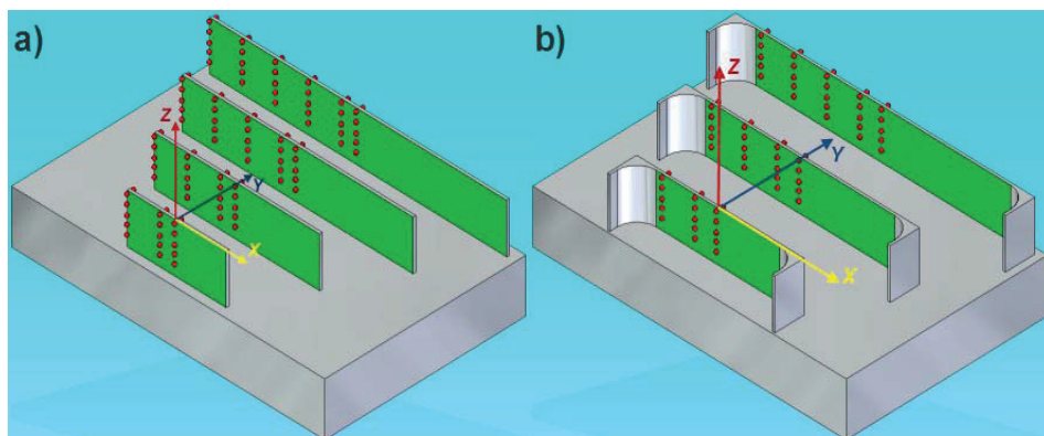
Rys. 3.13. Położenie układu współrzędnych względem, którego wykonano pomiary ścianek: a) nieutwierdzonych, b) utwierdzonych
