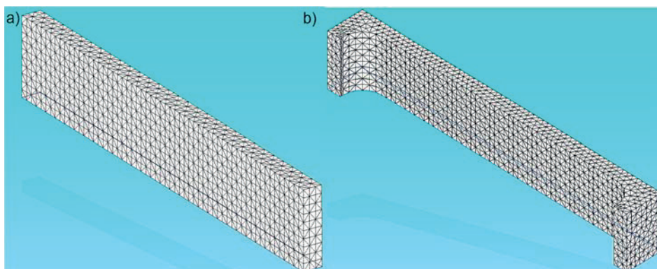
Rys. 5.5. Przykłady wygenerowanych siatek elementów skończonych dla ścianek: a) nieutwardzonych, b) utwardzonych
