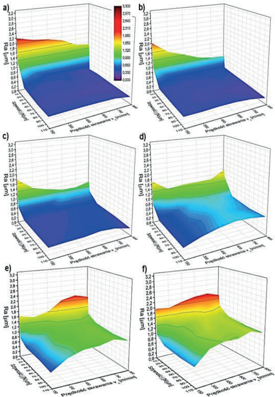
Chropowość powierzchni ścianek nientwierdzonych wykonanych ze stopu EN AW-6082; grubości ścianek: a) g=4,0\text{mm} ; b) g=2,8\text{mm} ; c) g=2,0\text{mm} ; d) g=1,4\text{mm} ; e) g=1,0\text{mm} ; f) g=0,7\text{mm}
