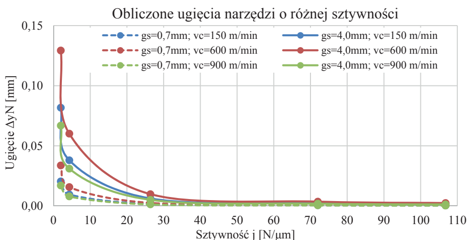
Rys. 6.4. Wartości ugięcia narzędzi o różnej sztywności dla wybranych grubości ścianek g_s i prędkości skrawania v_c
