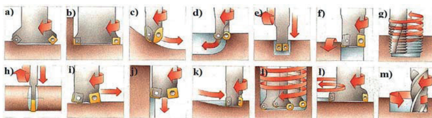
Rys. 1.3. Typy operacji frezarskich [90]
