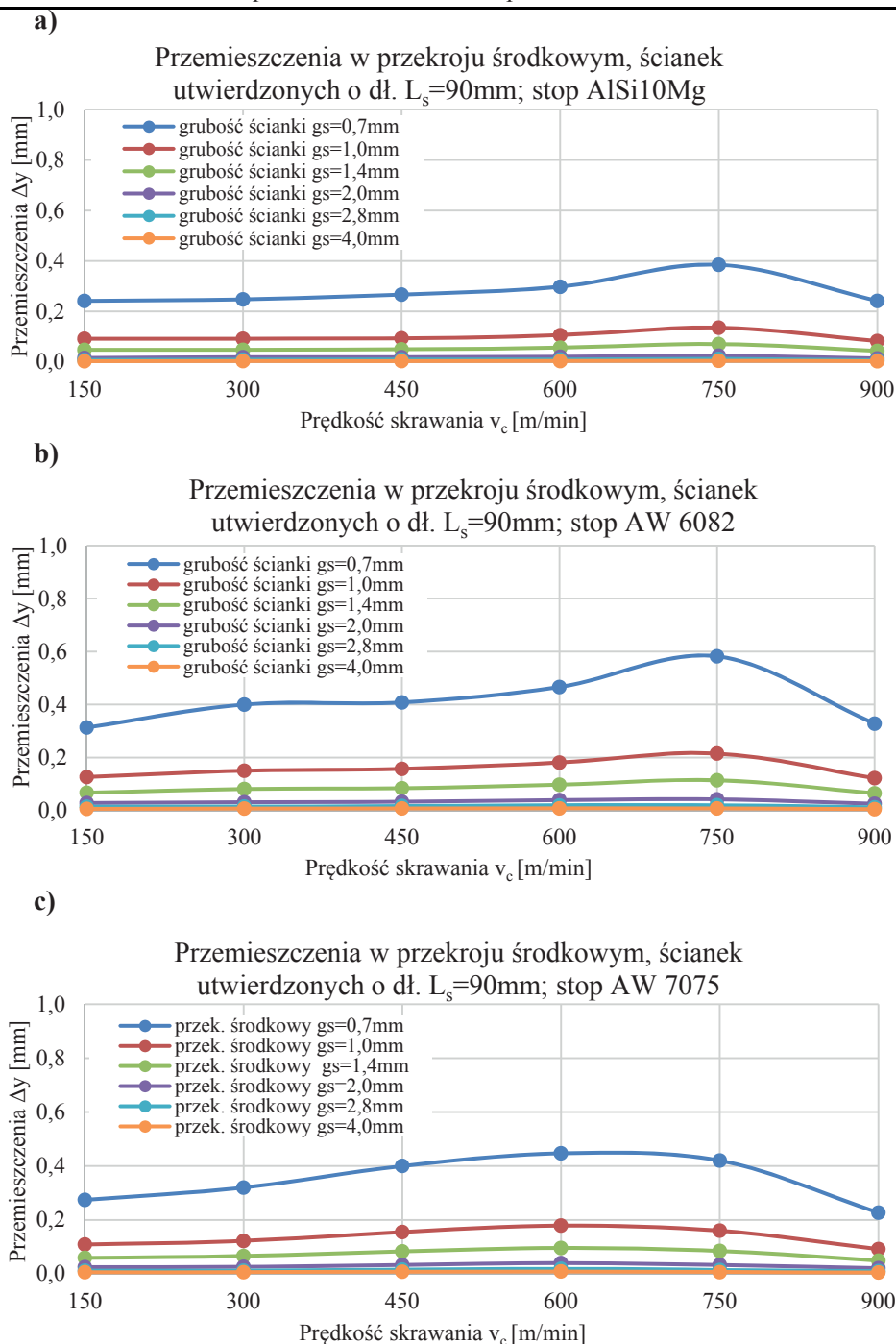
Rys. 5.12. Przemieszczenie w przekrojach środkowych ścianek utwardzonych o różnych długościach i grubości dla stopów: a) AlSi10Mg, b) AW-6082, c) AW-7075
