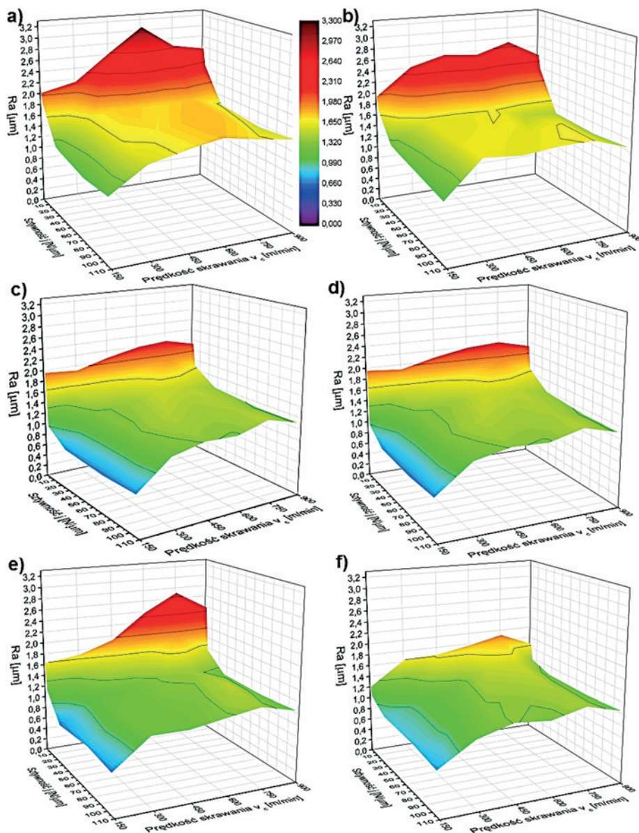
Rys. 6.34. Chropowość powierzchni ścianek nieutwardzonych i utwardzonych o grubości g_s=0,7 mm, wykonanych z różnych stopów Al: a) AlSi10Mg, nieutw.; b) AlSi10Mg, utw.; c) AW-6082, nieutw.; d) AW-6082, utw.; e) AW-7075, nieutw.; f) AW-7075, utw.
