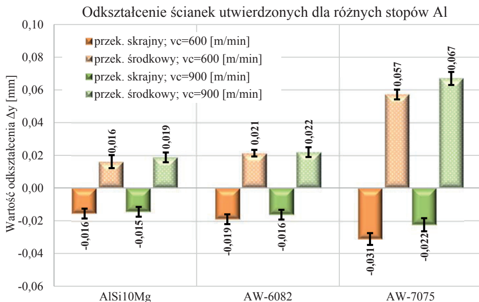
Rys. 6.20. Wartości odkształcenia w przekrojach skrajnych i środkowych ścianek utwardzonych o długości L_s=90 mm i grubości g_s=0,7 mm, wykonanych z różnych stopów Al narzędziem o sztywności j=2,0 N/ \mu m
