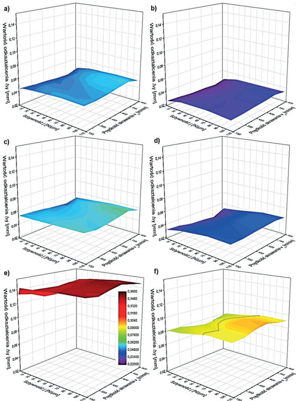
Rys. 6.8. Wartości odkształcenia w przekrojach skrajnych i środkowych ścianek nieutwardzonych o długości L_s=90\text{mm} i grubości g_s=0,7\text{mm} wykonanych z różnych stopów Al : a) przekrój skrajny stop AlSi10Mg; b) przekrój środkowy stop AlSi10Mg; c) przekrój skrajny stop EN AW-6082; d) przekrój środkowy stop EN AW-6082; e) przekrój skrajny stop EN AW-7075; f) przekrój środkowy stop EN AW-7075
