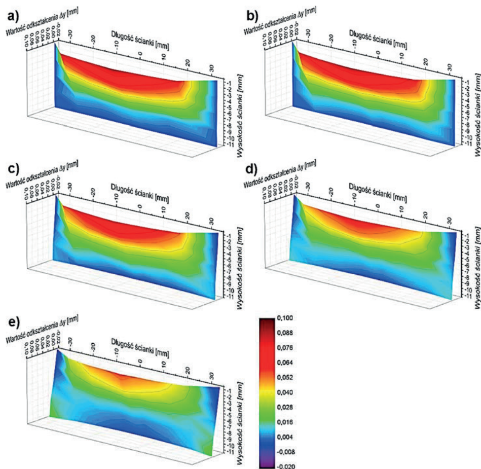
Rys. 6.17. Zarys powierzchni bocznej ścianek utwierdzonych o długości L_s=90\text{mm} i grubości g_s=0,7\text{mm} ; materiał EN AW-7075; prędkość skrawania v_c=600\text{m/min} ; sztywność narzędzi j : a) 106,8 \text{ N}/\mu\text{m} , b) 72 \text{ N}/\mu\text{m} , c) 26,4 \text{ N}/\mu\text{m} , d) 4,3 \text{ N}/\mu\text{m} , e) 2,0 \text{ N}/\mu\text{m}
