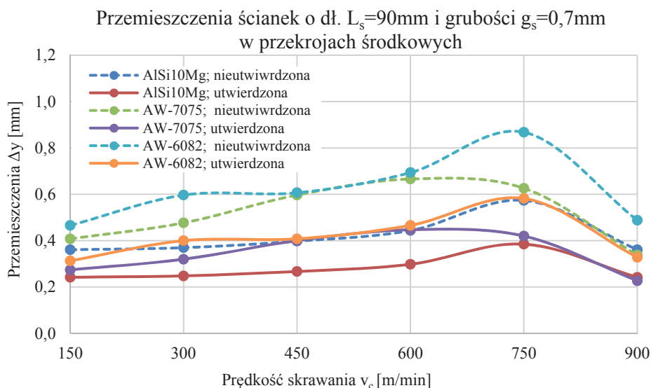
Rys. 5.15. Przemieszczenie w przekrojach środkowych ścianek nieutwardzonych i utwardzonych o długości L_s = 90 mm i grubości g_s = 0,7 mm
