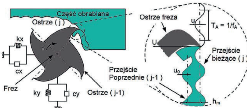
Rys. 1.21. Schemat powstawania drgań karbujących [13]
