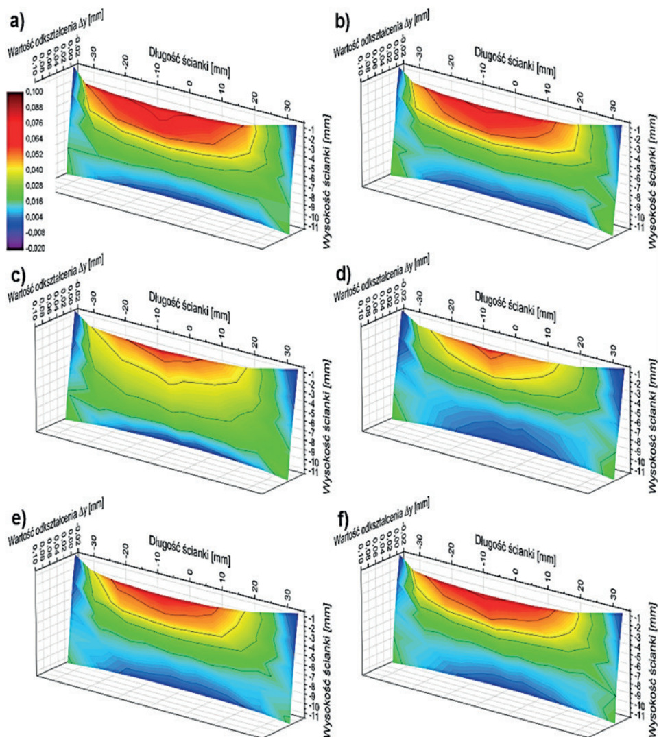
Rys. 6.15. Zarys powierzchni bocznej ścianek utwardzonych o długości L_s=90\text{mm} i grubości g_s=0,7\text{mm} ; materiał EN AW-7075; sztywność narzędzia j=2,0\text{ N}/\mu\text{m} ; prędkości skrawania v_c : a) 150 m/min, b) 300 m/min, c) 450 m/min, d) 600 m/min, e) 750 m/min, f) 900 m/min
