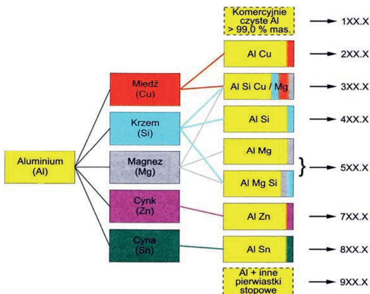
Rys. 1.19. Podział odlewniczych stopów aluminium [69]
