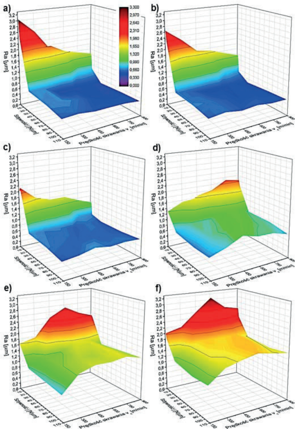
Chropowość powierzchni ścianek nieutwardzonych wykonanych ze stopu \text{AlSi10Mg} ; grubości ścianek: a) g=4.0\text{mm} ; b) g=2.8\text{mm} ; c) g=2.0\text{mm} ; d) g=1.4\text{mm} ; e) g=1.0\text{mm} ; f) g=0.7\text{mm}
