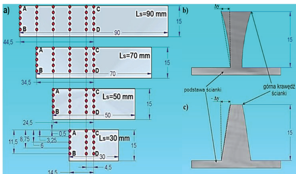
Rys. 3.12. Pomiary dokładności ścianek: a) rozmieszczenie punktów pomiarowych, b) kształt ścianki – odchyłka dodatnia, c) kształt ścianki – odchyłka ujemna
