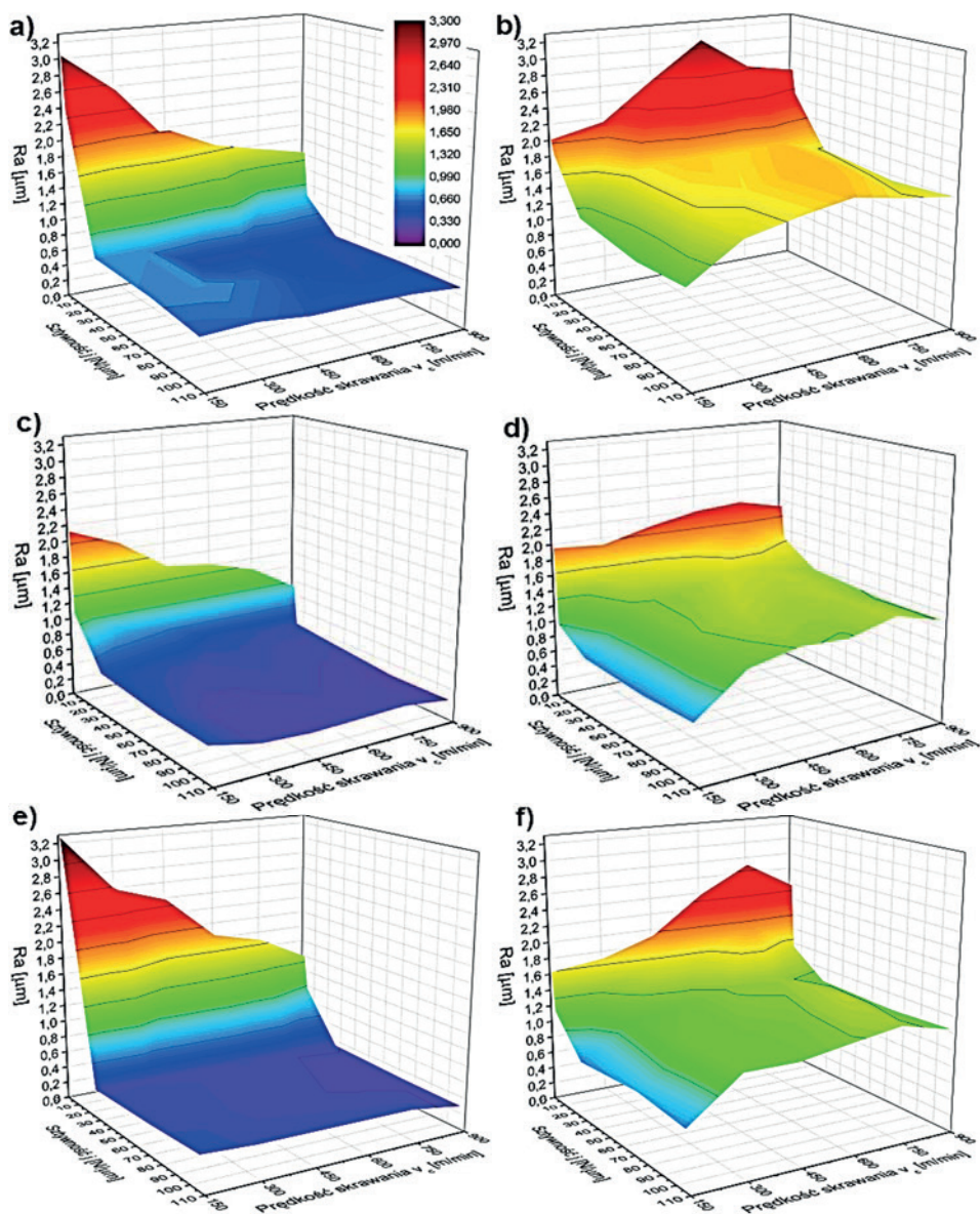
Rys. 6.32. Chropowość powierzchni ścianek nieutwardzonych wykonanych z różnych stopów Al: a) AlSi10Mg, g_s=4,0\text{mm} ; b) AlSi10Mg, g_s=0,7\text{mm} ; c) AW-6082, g_s=4,0\text{mm} ; d) AW-6082, g_s=0,7\text{mm} ; e) AW-7075, g_s=4,0\text{mm} ; f) AW-7075, g_s=0,7\text{mm}
