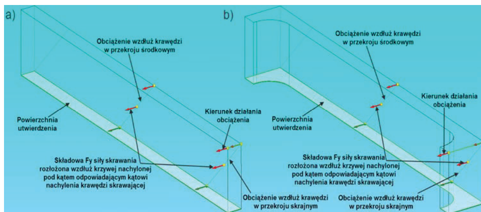
Rys. 5.4. Modele obciążenia oraz utwierdzenia przyjęte w analizie MES: a) nieutwardzonych, b) utwardzonych
