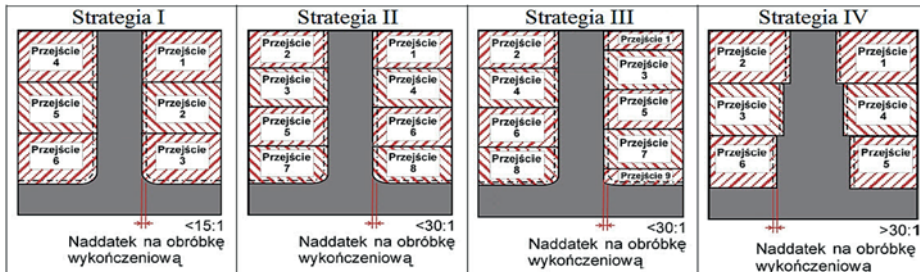
Rys. 1.26. Strategie obróbki cienkich ścianek [90, 103]
