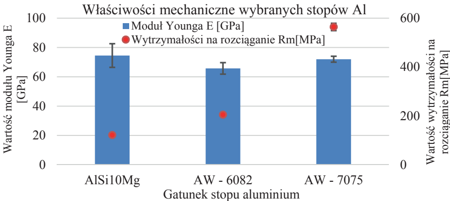
Rys. 5.3. Moduł Younga oraz wytrzymałość na rozciąganie wybranych stopów aluminium
