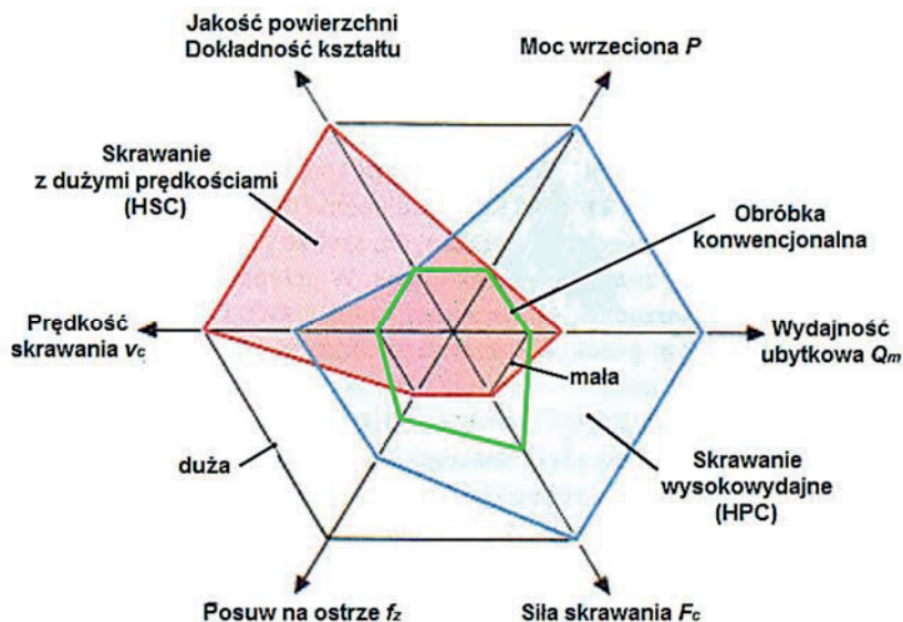
Rys. 1.11. Porównanie obróbki konwencjonalnej z obróbkami HSC i HPC [16, 67, 69]
