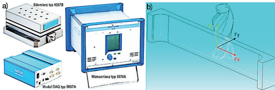
Rys. 3.9. Pomiar sił skrawania: a) zestaw do pomiaru sił z siłomierzem 9257B, b) rozkład siły skrawania na mierzone składowe F_x , F_y , F_z [43]
