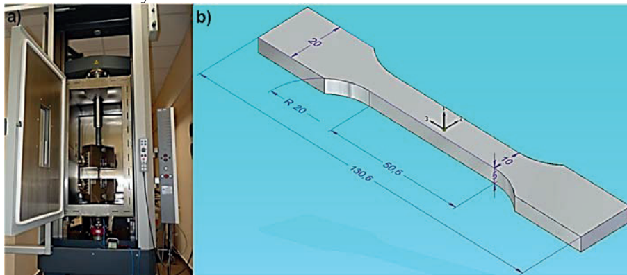
Rys. 3.8. Statyczna próba rozciągania: a) maszyna wytrzymałościowa Zwick/Roell Z150, b) kształt i wymiary próbek wg. PN-EN 10002-1:2004 [64]
