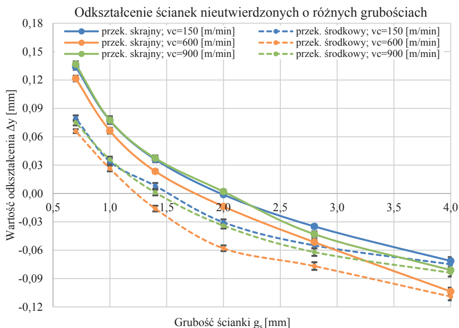
Rys. 6.10. Wartości odkształcenia w przekrojach skrajnych i środkowych ścianek nieutwardzonych o różnych grubościach i długości L_s=90 mm, wykonanych ze stopu EN AW-7075 narzędziem o sztywności j=2,0 N/ \mu m
