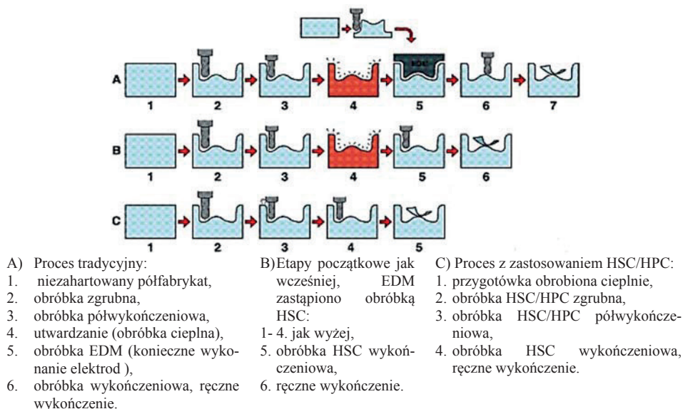
Rys. 1.4. Usprawnienie procesu produkcyjnego - redukcja czasu produkcji w procesie C) w stosunku do procesu A) na poziomie 30 - 50% [74, 87]
