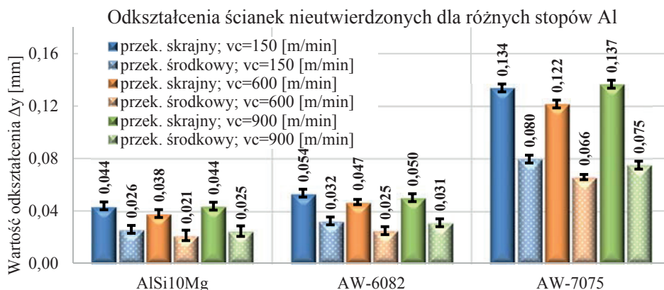
Rys. 6.7. Wartości odkształcenia w przekrojach skrajnych i środkowych ścianek nieutwardzonych długości L_s=90 mm i grubości g_s=0,7 mm, wykonanych z różnych stopów Al narzędziem o sztywności j=2,0 N/ \mu m
