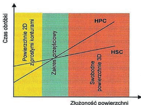
Rys. 1.13. Wybór obróbki HSC lub HPC w zależności od stopnia złożoności [68]
