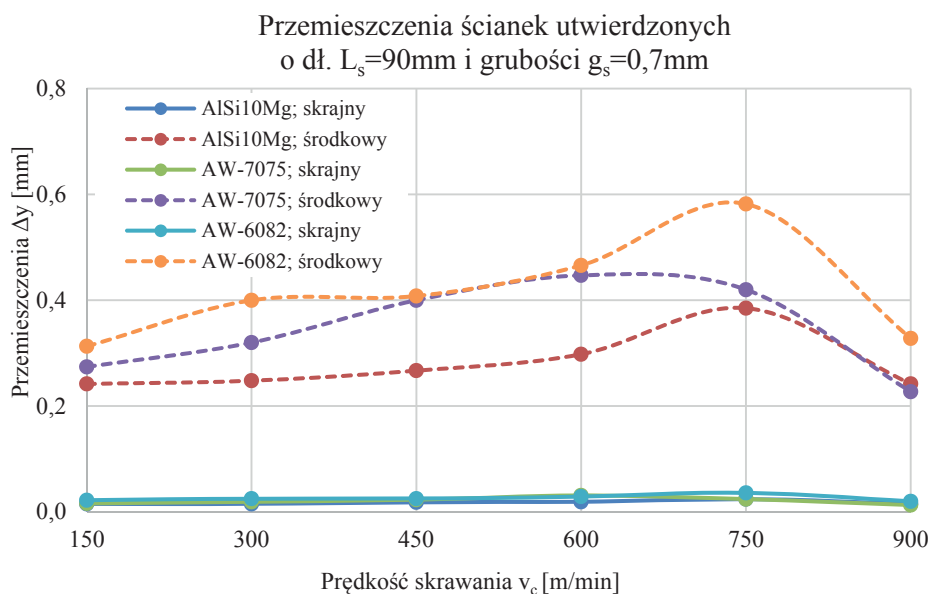
Rys. 5.13. Przemieszczenie w przekrojach środkowych i skrajnych ścianek utwardzonych
