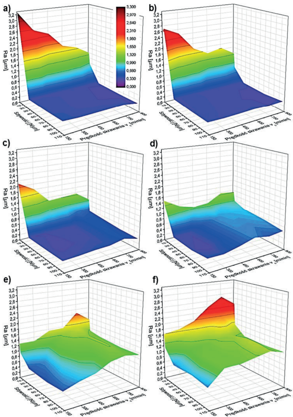
Rys. 6.30. Chropowość powierzchni ścianek nieutwardzonych wykonanych ze stopu EN AW-7075; grubości ścianek g_s : a) 4,0mm; b) 2,8mm; c) 2,0mm; d) 1,4mm; e) 1,0mm; f) 0,7mm
