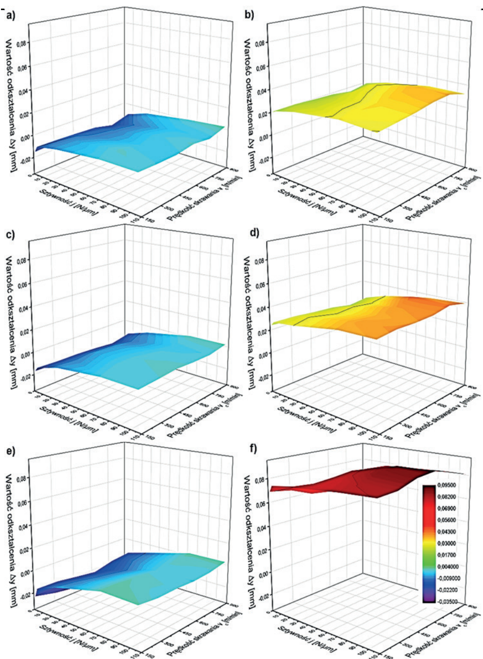
Rys. 6.21. Wartości odkształcenia w przekrojach skrajnych i środkowych ścianek utwardzonych o długości L_s=90\text{mm} i grubości g_s=0,7\text{mm} wykonanych z różnych stopów Al:
