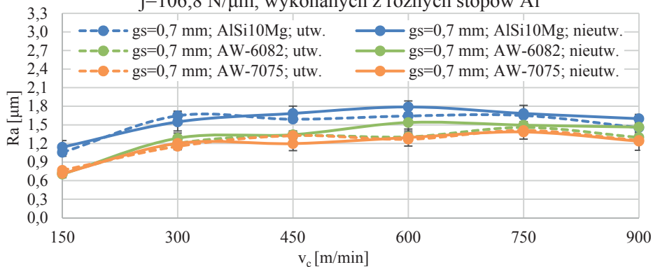
b) Chropowatość powierzchni ścianek utwardzonych i nieutwardzonych obrobionych narzędziem o sztywności j=2,0 N/ \mu m, wykonanych z różnych stopów Al
