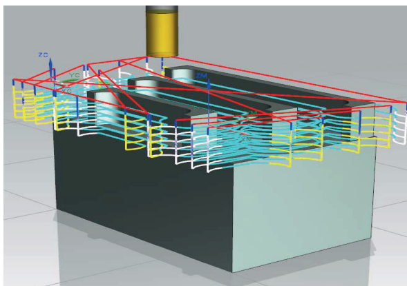
Rys. 3.5. Przykład ścieżek obróbkowych wygenerowanych w NX 8.0
