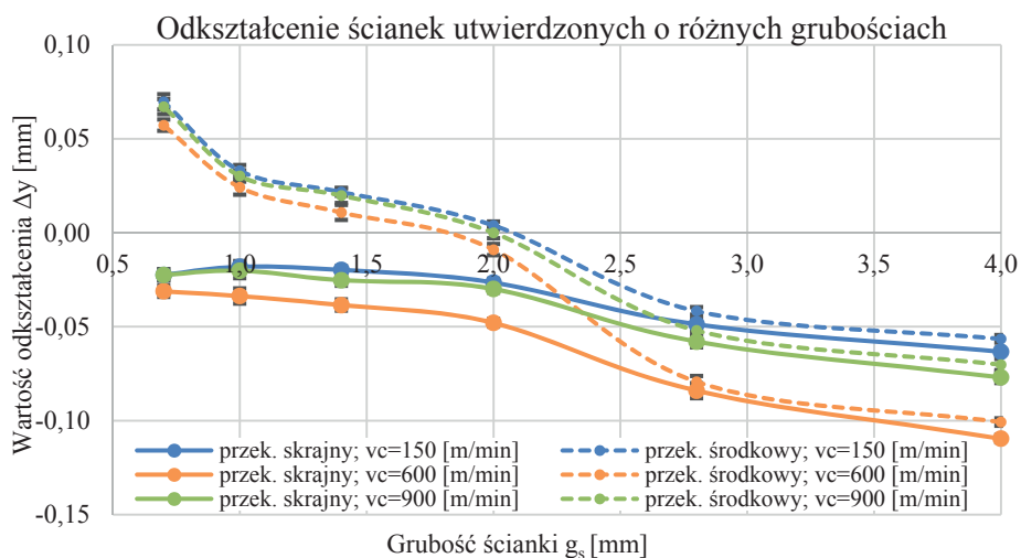
Rys. 6.23. Wartości odkształcenia w przekrojach skrajnych i środkowych ścianek utwardzonych o różnych grubościach i długości L_s=90 mm, wykonanych ze stopu EN AW-7075 narzędziem o sztywności j=2,0 N/ \mu m
