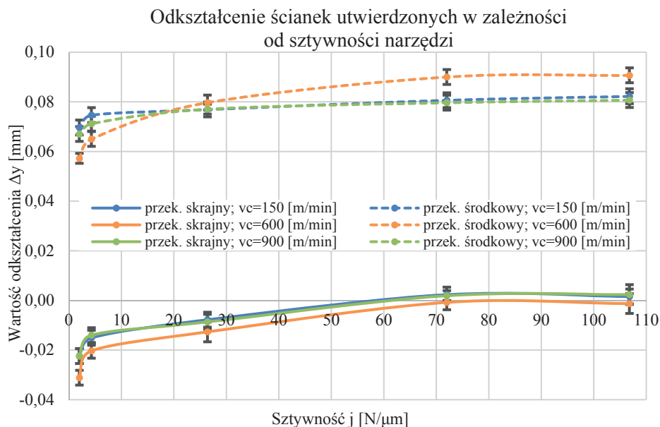
Rys. 6.18. Wartości odkształcenia w przekrojach skrajnych i środkowych ścianek utwardzonych o długości L_s = 90 \text{ mm} i grubości g_s = 0,7 \text{ mm} , wykonanych ze stopu EN AW-7075 narzędziami o różnej sztywności
