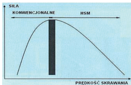
Rys. 1.5. Przebieg sił skrawania w funkcji prędkości [1, 2]
