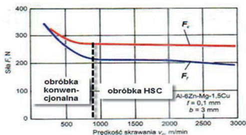
Rys. 1.6. Zależność składowych siły skrawania od prędkości skrawania przy toczeniu stopu Al6ZnMg1,5Cu [69]
