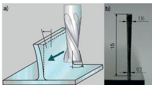
Rys. 1.25. Zjawiska towarzyszące obróbce elementów cienkościennych a) odkształcenie ścianki i narzędzia [10], b) przykładowy zarys ścianki po obróbce
