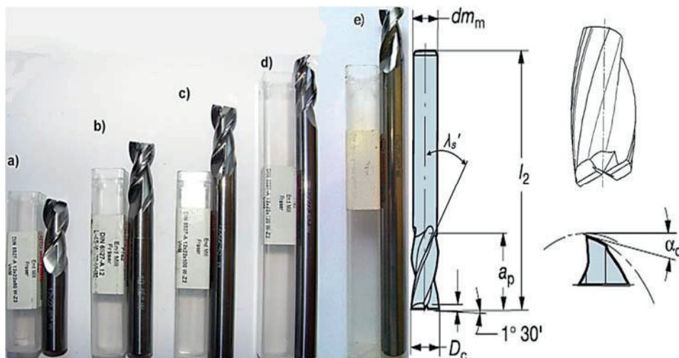
Rys. 3.3. Widoki i geometria frezów zastosowanych do badań; frezy o długościach: a) 60 mm, b) 80mm, c) 100 mm, d) 120 mm, e) 140mm
