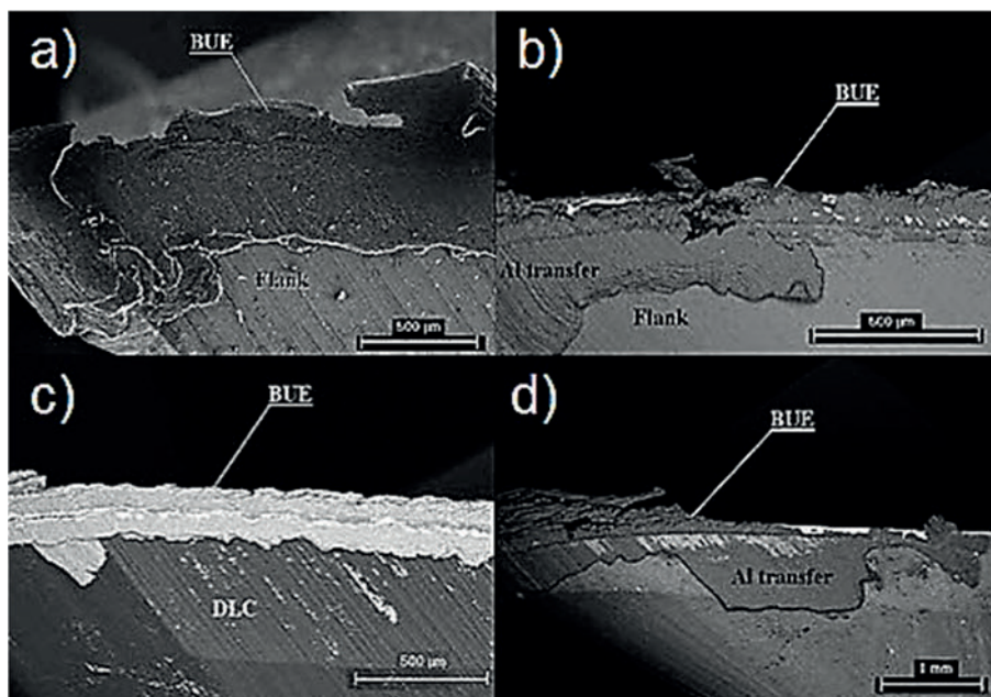
Rys. 1.15. Powstawanie narostu na krawędzi skrawającej: a) ostrze bez powłoki, b) powłoka TiAlCrYN, c) powłoka diamentowa DLC, d) powłoka TiAlN/VN [36]
