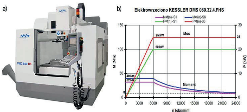
Rys. 3.6. Centrum frezarskie VMC 800HS: a) widok ogólny, b) charakterystyka elektrowrzeciona [8]
