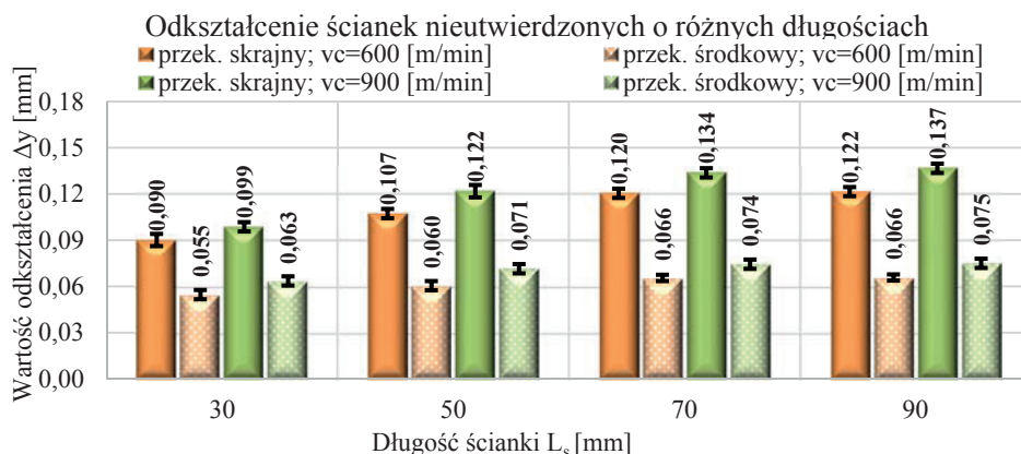
Rys. 6.13. Wartości odkształcenia w przekrojach skrajnych i środkowych ścianek nieutwierdzonych o różnych długościach i grubości g_s = 0,7 mm, wykonanych ze stopu EN AW-7075 narzędziem o sztywności 2,0 N/mm
