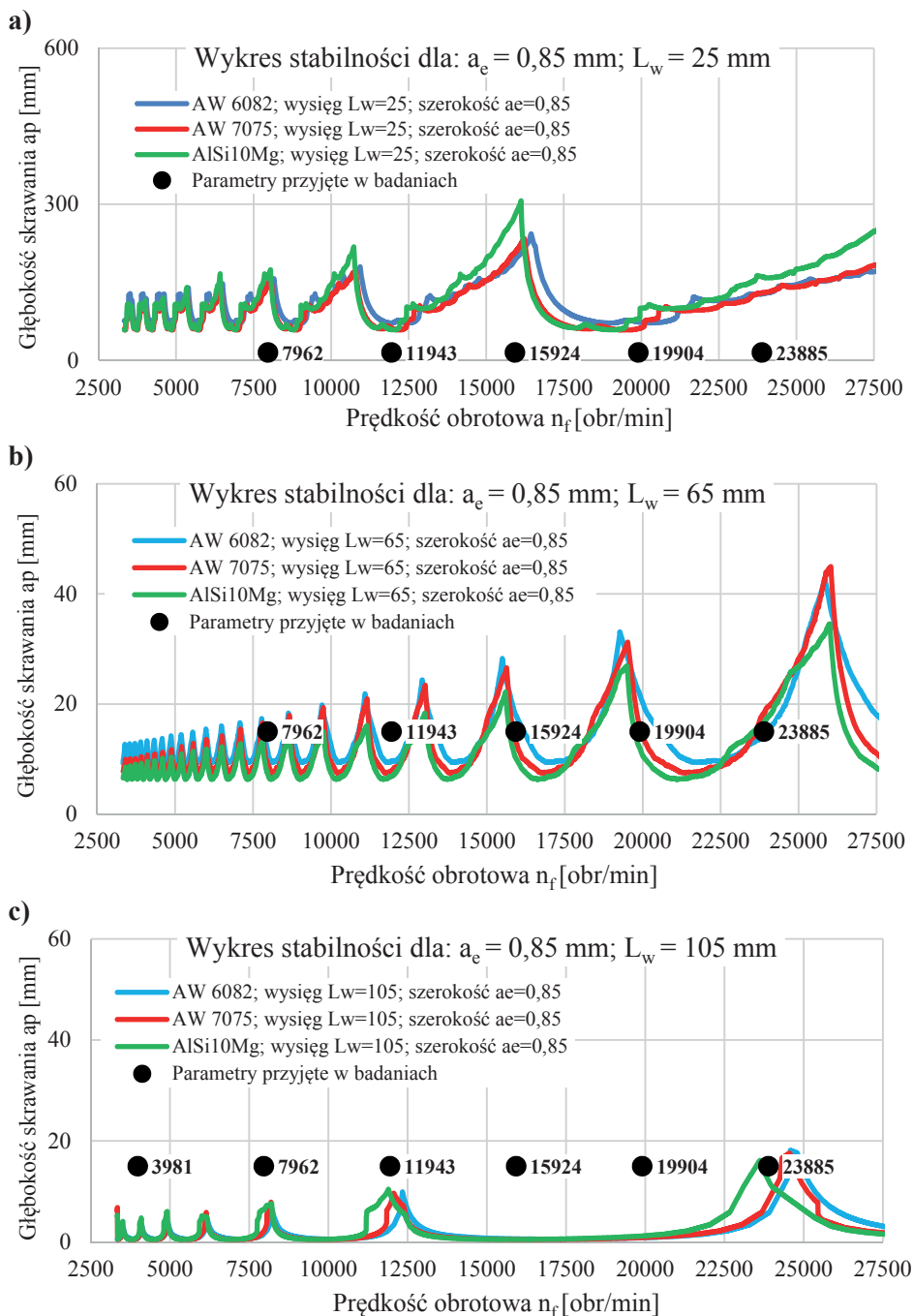
Rys. 4.3. Przykładowe wykresy stabilności dla głębokości skrawania a_p = 15 \text{ mm} i szerokości frezowania a_e = 0,85 \text{ mm} oraz różnych wysięgów narzędzia:
