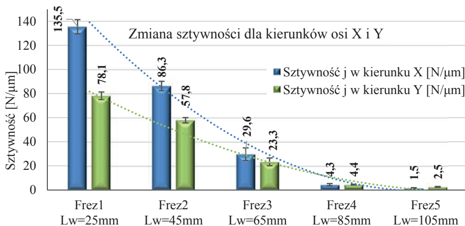
Rys. 4.1. Zmiana sztywności „modalnej” układu narzędzie–oprawka–wrzeciono w zależności od długości wysięgu narzędzia dla dwu kierunków pomiaru: X i Y
