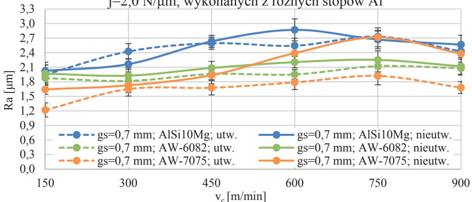
Rys. 6.33. Chropowatość powierzchni ścianek utwardzonych i nieutwardzonych o grubości g_s=0,7 mm, wykonanych z różnych stopów Al narzędziami o sztywności j : a) 106,8 N/ \mu m; b) 2,0 N/ \mu m
