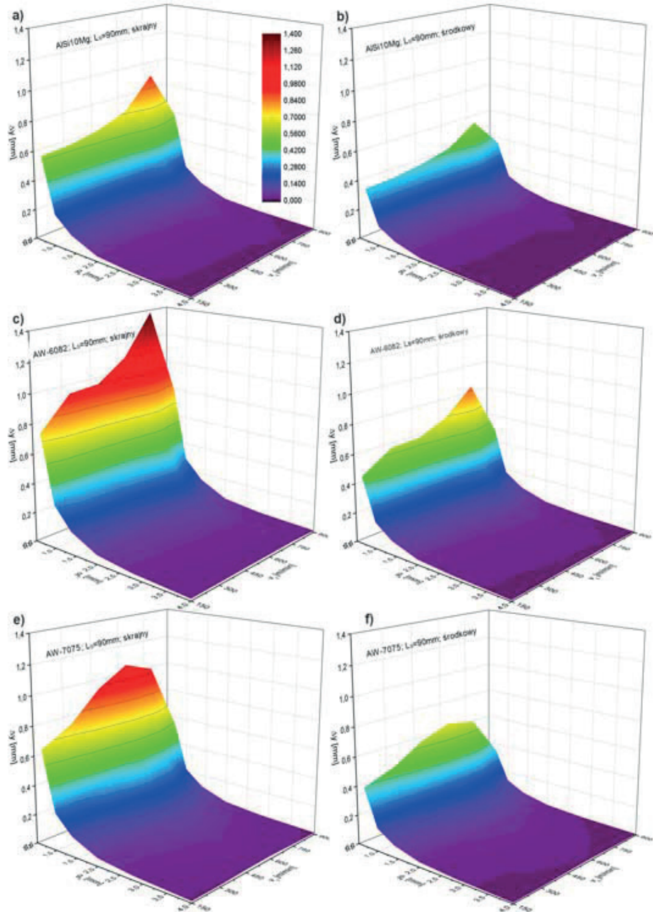
Przesunięcia ścianek nienastępnionych o długości L_s = 90\text{ mm} i grubości g_s = 0,7\text{ mm} dla: a) stop AlSi10Mg, przekrój skrajny; b) stop AlSi10Mg, przekrój środkowy; c) stop AW-6082, przekrój skrajny; d) stop AW-6082, przekrój środkowy; e) stop AW-7075, przekrój skrajny; f) stop AW-7075, przekrój środkowy (obliczenia MES)
