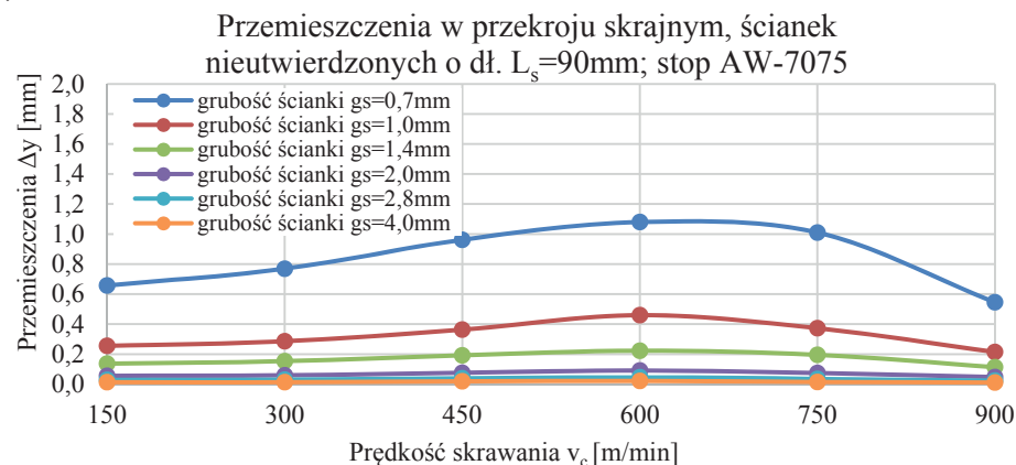
Rys. 5.9. Przemieszczenie w przekrojach skrajnych ścianek nieutwardzonych o różnych długościach i grubościach dla stopów: a) AlSi10Mg, b) AW-6082, c) AW-7075
