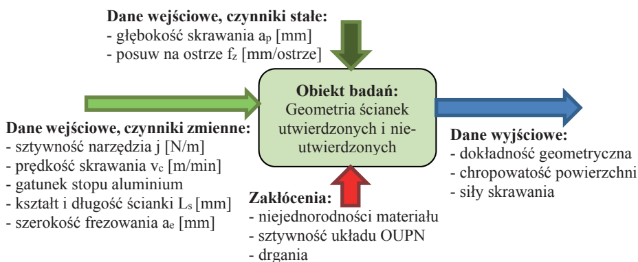
Rys. 3.1. Model obiektu badań
