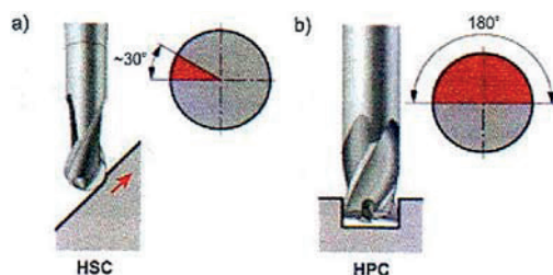
Rys. 1.12. Warunki styku ostrzy narzędzi z przedmiotem obrabianym [67, 69]
