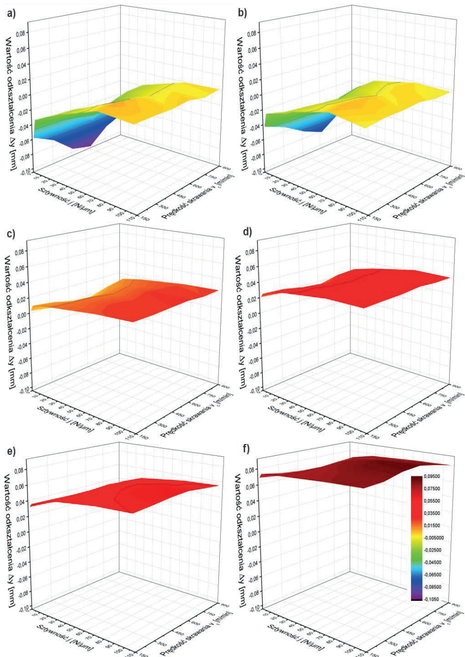
Rys. 6.24. Wartości odkształcenia w przekrojach środkowych ścianek utwardzonych o długości L_s=90\text{mm} wykonanych ze stopu EN AW-7075 narzędziem o sztywności j=2,0\text{ N}/\mu\text{m} ; grubości ścianek: a) 4,0 mm, b) 2,8 mm, c) 2,0 mm, d) 1,4 mm, e) 1,0 mm, f) 0,7 mm
