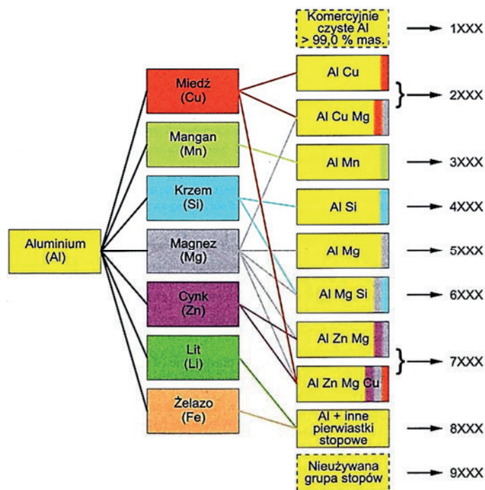
Rys. 1.18. Podział stopów aluminium do obróbki plastycznej [60, 69]
