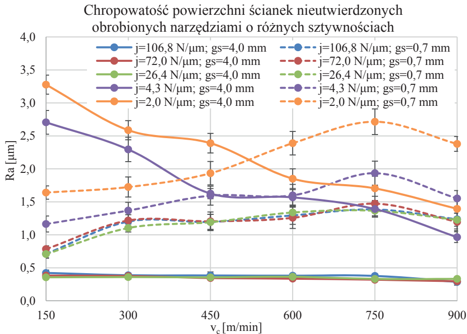
Rys. 6.28. Chropowatość powierzchni ścianek nieutwardzonych o grubości g_s=4,0 mm i g_s=0,7 mm, wykonanych ze stopu EN AW-7075 narzędziami o różnej sztywności
