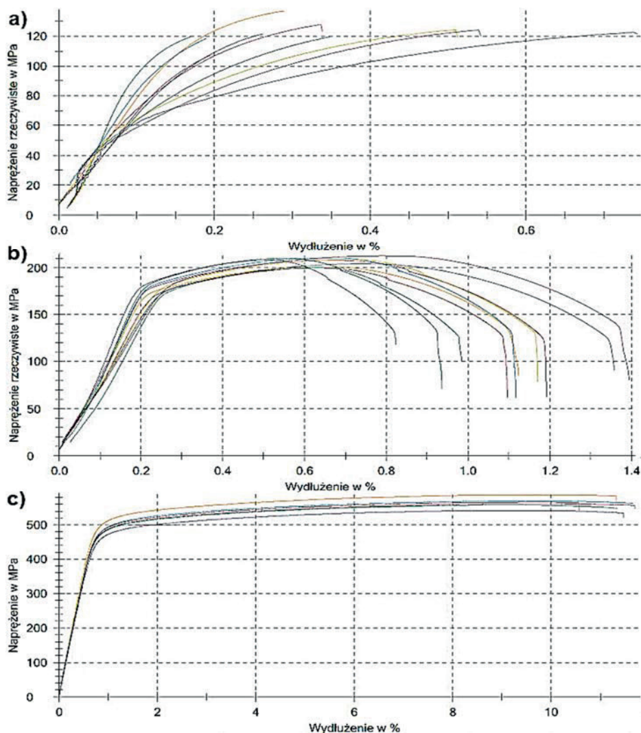
Rys. 5.2. Wyniki badań wytrzymałościowych wg PN EN 10002-1[64] dla stopów: a) AlSi10Mg, b) AW 6082, c) AW 7075
