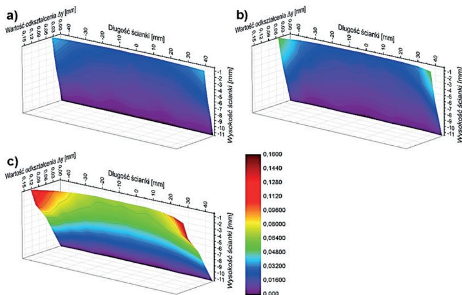
Rys. 6.6. Zarys powierzchni bocznej ścianek nieutwardzonych o długości L_s=90\text{mm} i grubości g_s=0,7\text{mm} ; prędkość skrawania v_c=600\text{m/min} ; sztywność narzędzia j=2,0\text{ N}/\mu\text{m} ; materiał: a) AlSi10Mg , b) EN AW-6082 , c) EN AW-7075
