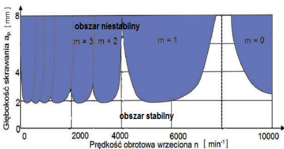
Rys. 1.22. Przykładowy wykres stabilności – krzywa workowa [13, 85]
