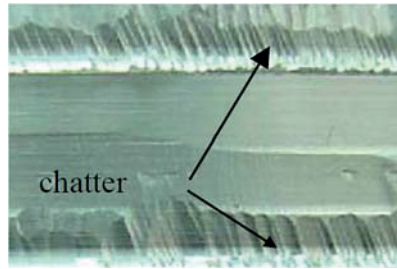
Rys. 1.20. Efekt niestabilnej pracy narzędzia - karbowanie (chatter) [12]
