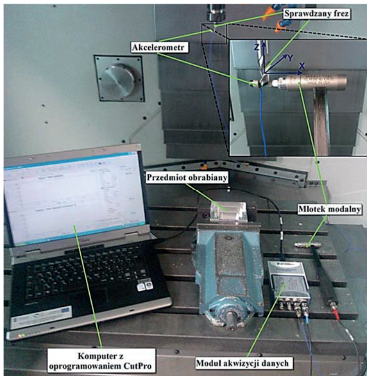
Rys. 3.7. Zestaw do analizy modalnej
