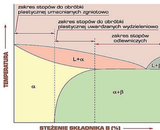
Rys. 1.17. Fragment wykresu równowagi stopów Al do obróbki plastycznej, umacnianych przez zgniot i utwardzanych wydzieleniowo oraz stopów odlewniczych [20]
