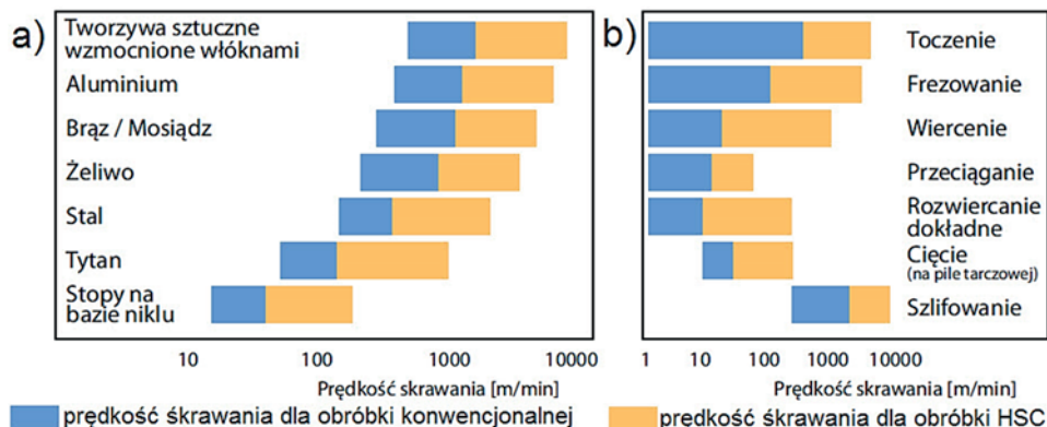
Rys. 1.8. Porównanie zakresów prędkości skrawania v_c dla obróbki konwencjonalnej i HSC, w zależności od: a) rodzaju materiału obrabianego, b) sposobu skrawania [16, 28]
