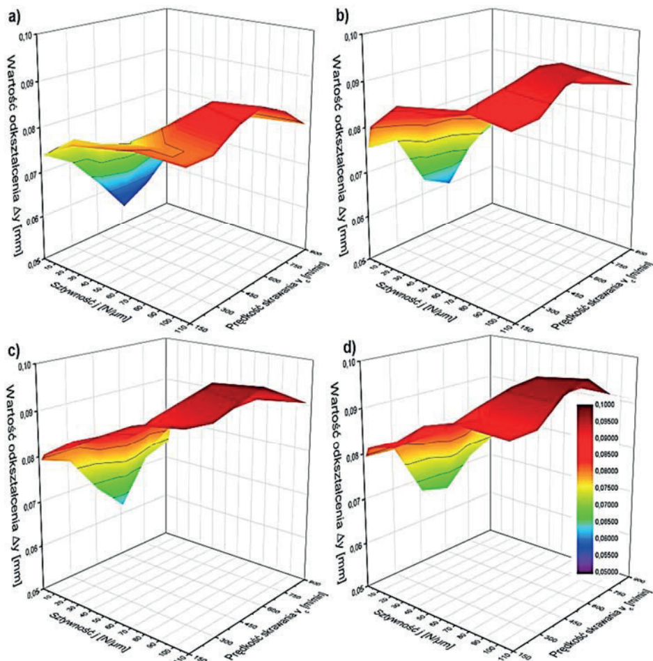
Rys. 6.14. Wartości odkształcenia w przekrojach środkowych ścianek nieutwardzonych o grubości g_s=0,7\text{ mm} wykonanych ze stopu EN AW-7075 narzędziem o sztywności j=2,0\text{ N}/\mu\text{m} ; długość ścianek: a) 30 mm, b) 50 mm, c) 70 mm, d) 90 mm
