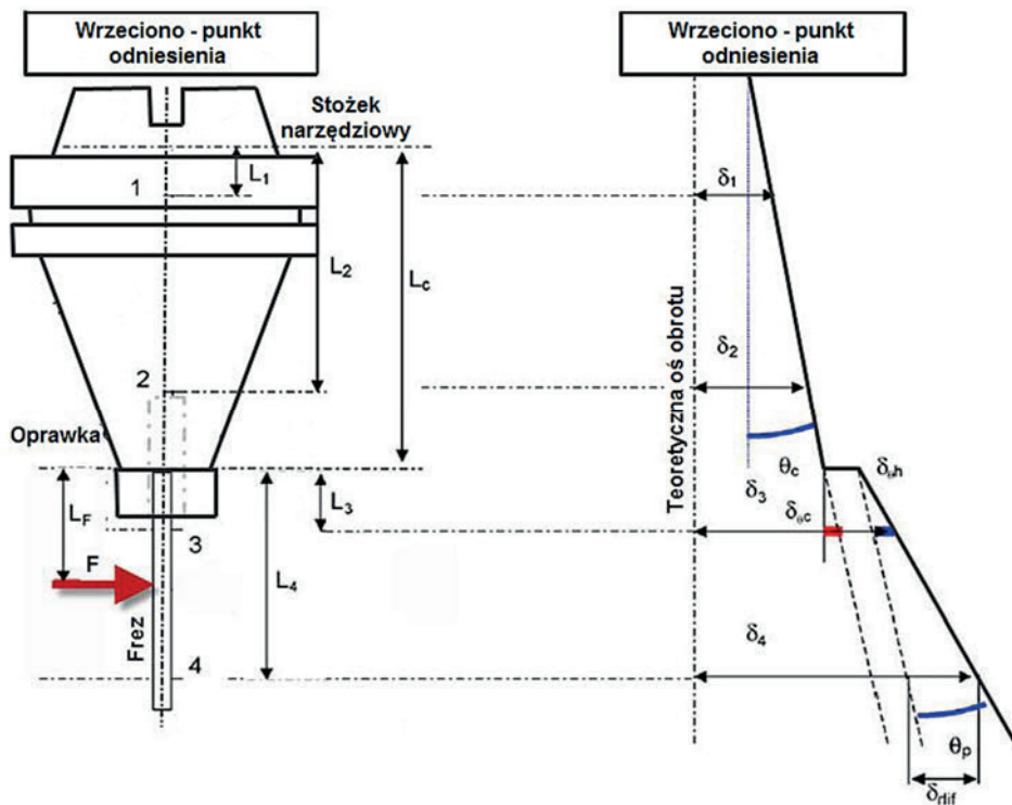
Rys. 1.23. Odształcenia układu narzędzie-oprawka-wrzeciono [86]
