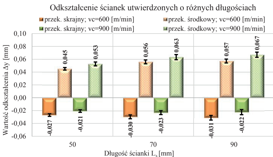
Rys. 6.26. Wartości odkształcenia w przekrojach skrajnych i środkowych ścianek utwardzonych o różnej długości i grubości g_s=0,7 mm, wykonanych ze stopu EN AW-7075 narzędziem o sztywności j=2,0 N/ \mu m
