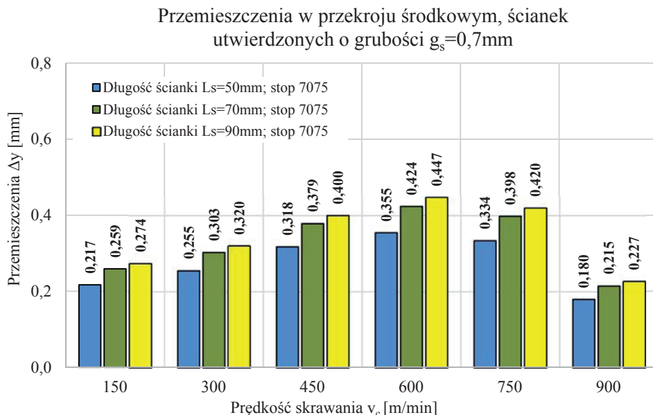
Rys. 5.14. Przemieszczenie ścianek utwardzonych o grubości g_s = 0,7\text{ mm} i różnych długościach L_s wykonanych ze stopu AW-7075, w przekrojach środkowych
