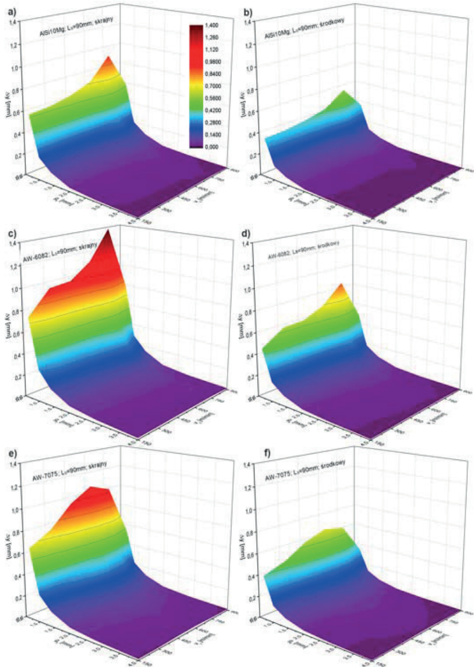
Premieszczenia ścianek nientwierdzonych o długości L_s = 90 mm i grubości g_s = 0,7 mm dla: a) stop AlSi10Mg, przekrój skrajny; b) stop AlSi10Mg, przekrój środkowy; c) stop AW-6082, przekrój skrajny; d) stop AW-6082, przekrój środkowy; e) stop AW-7075, przekrój skrajny; f) stop AW-7075, przekrój środkowy (obliczenia MES)
