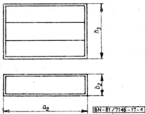
Rys. 4. Gablota nadstawna i wisząca
