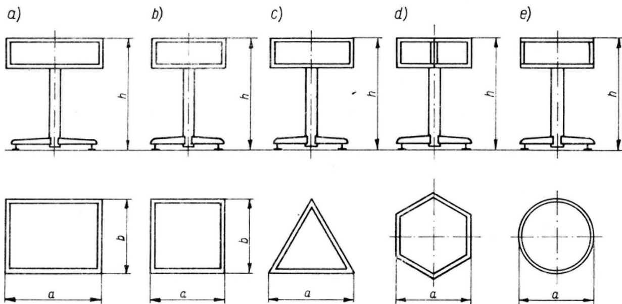
Rys. 2. Gablota stojakowa — przykłady kształtów
