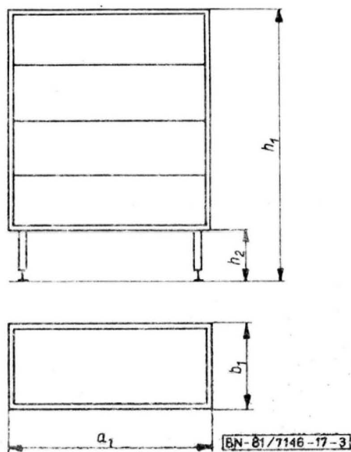
Rys. 3. Gablota wolno stojąca szafka
