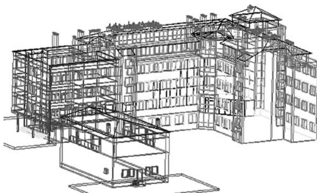
Rys. 3. Widok budynku WIŚ, ogląd koncepcyjny z lotu ptaka oraz ogląd szkieletowy od strony wsch., wykonał A. Urzędowski
