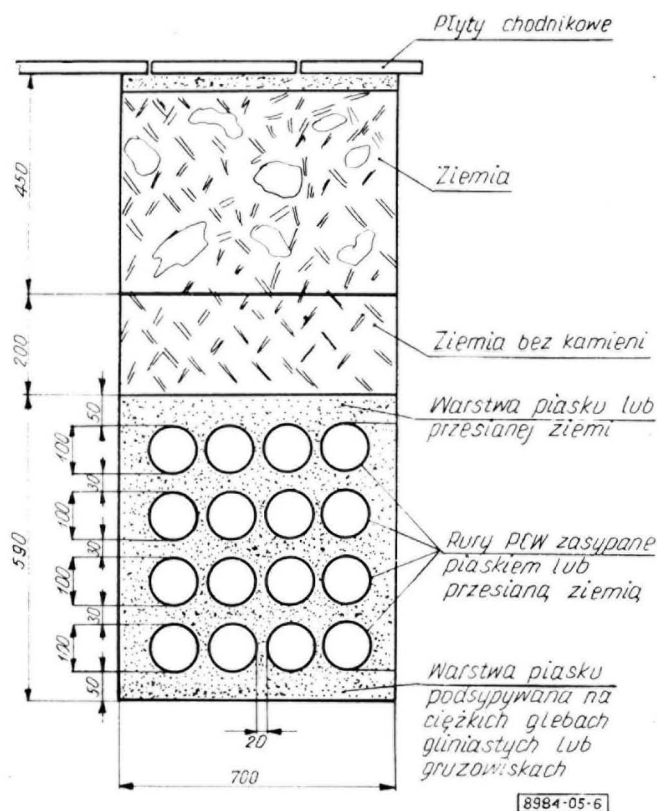
Rys. 6. Przekrój kanalizacji kablowej z rur PCW
