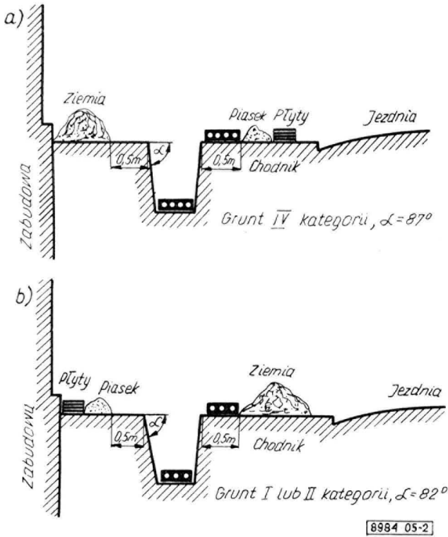
Rys. 2. Rozmieszczenie ziemi z wykopu, bloków i materiałów nawierzchni. Rysunek przykładowy
