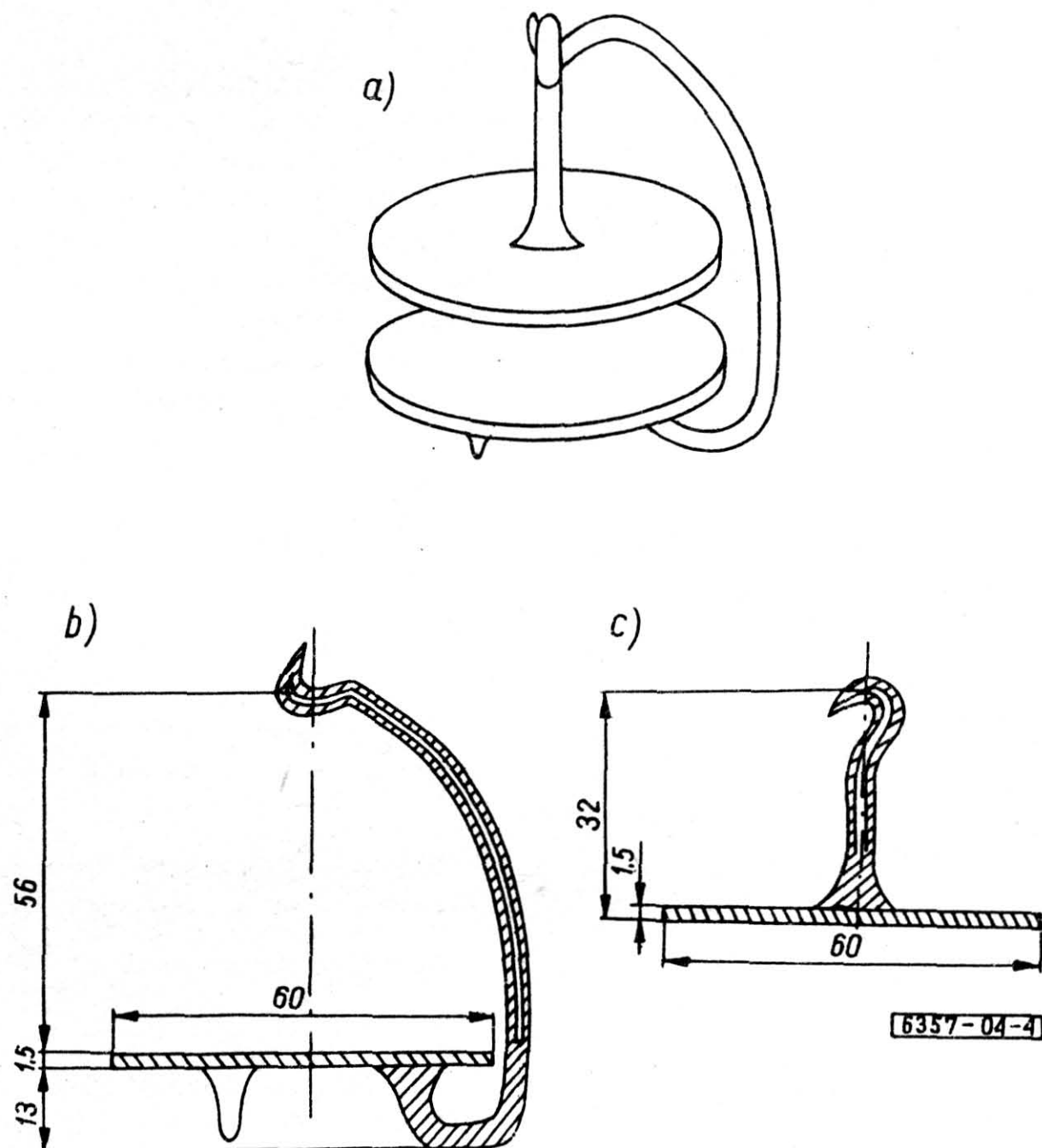
Rys. 4. Szkic do oznaczania suchej pozostałości
