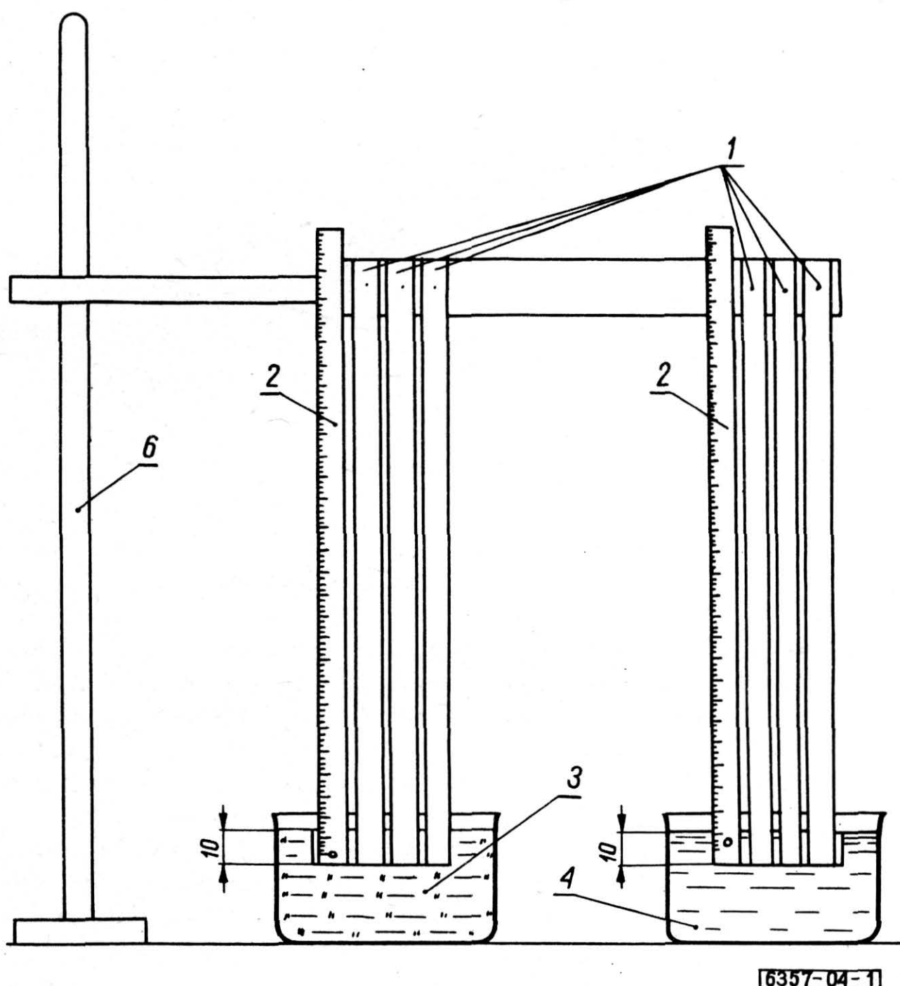
Rys. 1. Zestaw do oznaczania wsiakliwości
