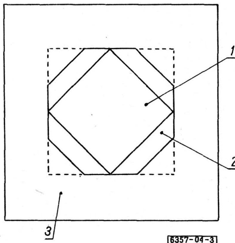
Rys. 3. Szkic do oznaczania czasu zdolności lepiącej 1 - kwadrat z kartonu o boku 40 mm, 2 - kwadrat z papieru o boku 56 mm, 3 - szablon z folii o grubości 0,1 mm i otworze w kształcie ośmiokąta równobocznego o boku 24 mm.
