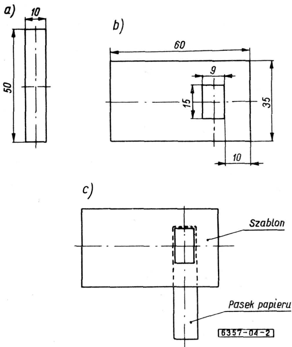
Rys. 2. Szkic do oznaczania czasu chwytania: a) pasek papieru, b) szablon z folii aluminiowej o grubości 0,1 mm, c) pasek papieru przykryty szablonem przygotowany do naniesienia kleju.
