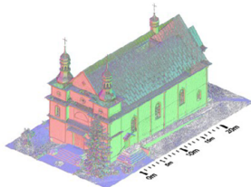
CHMURA PUNKTÓW OBIEKTU - NAROŻE PÓŁNOCNE
