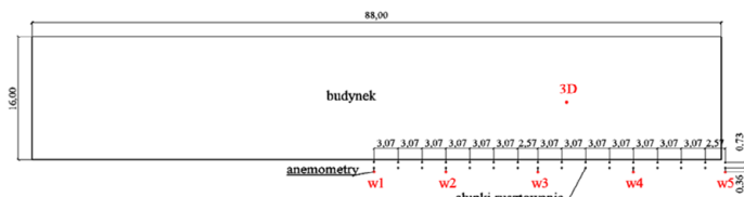
schemat rozmieszczenia anemometrów w stosunku do budynku (widok z góry, wymiary w [m])
