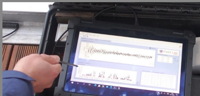
Badania dynamiczne kładki nad rzeką Bystrzycą w Lublinie Fot. Aleksandra Jaworska
