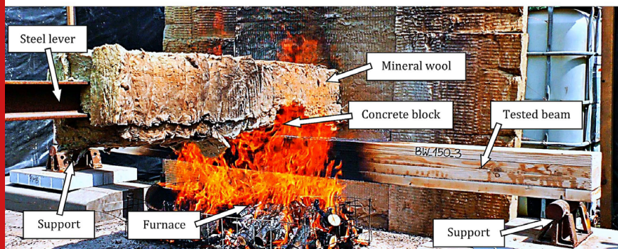
Badanie belek kompozytowych z drewna klejonego wzmacnianego taśmami CFRP
