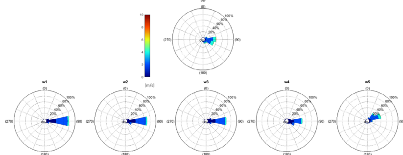
Różne wiatrów z pomiaru na rusztowaniu
