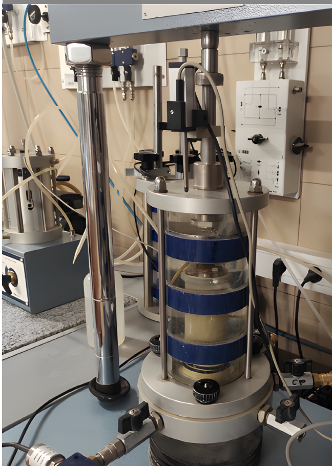
Badania laboratoryjne gruntów (ściskanie trójosiowe oraz edometryczne) Źródło: archiwum KIMBiG
