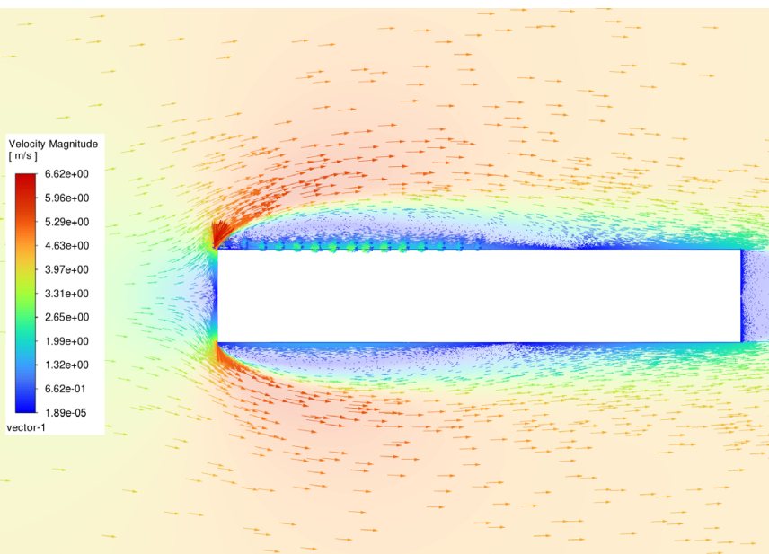
Ilustracja opływu wiatru wokół budynku z rusztowaniem
