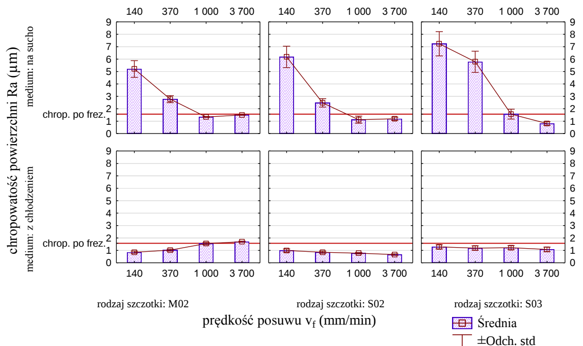
Rys. 4.51. Wpływ prędkości ruchu posuwowego w procesie szczotkowania stopu aluminium 7075-T651 na chropowatość powierzchni (obróbka poprzedzająca – frezowanie wykończeniowe)
