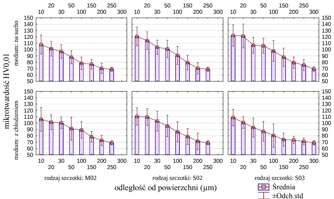
Rys. 4.62. Rozkład mikrotwardości w funkcji odległości od powierzchni po szczotkowaniu stopu magnezu AZ91HP
