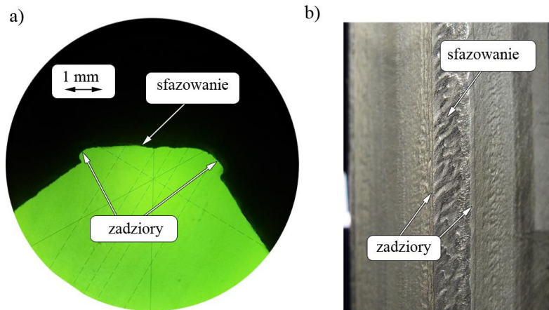
Rys. 4.29. Widok sfazowania z zadziorami w postaci wypłytki (stop AlSi10Mg, v_f = 140 mm/min, medium: na sucho): a) widok repliki, b) widok rzeczywisty
