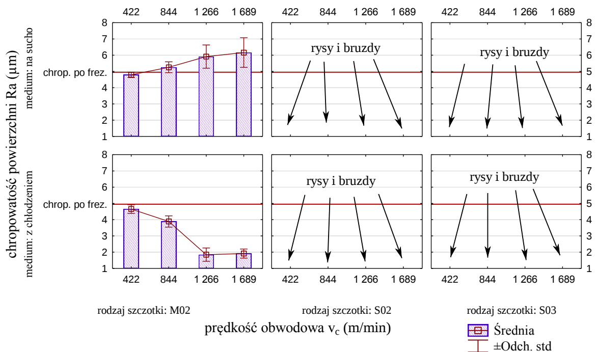
Rys. 4.32. Wpływ prędkości obwodowej w procesie szczotkowania stopu magnezu AZ31 na chropowatość powierzchni (obróbka poprzedzająca - frezowanie kształtujące)
