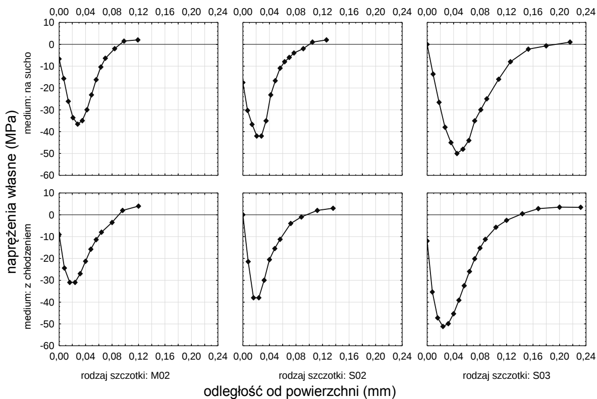
Rys. 4.67. Rozkład naprężeń własnych w funkcji odległości od powierzchni po szczotkowaniu stopu magnezu AZ31
