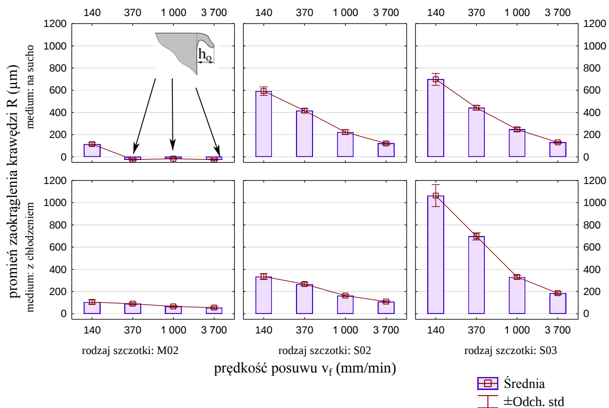
Rys. 4.26. Wpływ prędkości posuwu na promień zaokrąglenia krawędzi – materiał AZ91HP
