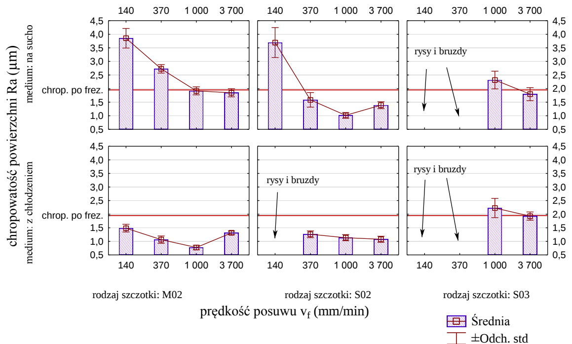
Rys. 4.49. Wpływ prędkości ruchu posuwowego w procesie szczotkowania stopu magnezu AZ31 na chropowatość powierzchni (obróbka poprzedzająca – frezowanie wykończeniowe)
