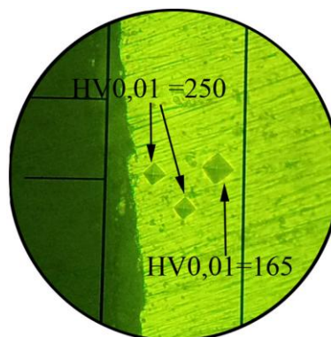
Rys. 4.63. Zgląd metalograficzny po obróbce szczotkowaniem stopu aluminium 7075-T651 (szczotka S03; medium: na sucho)
