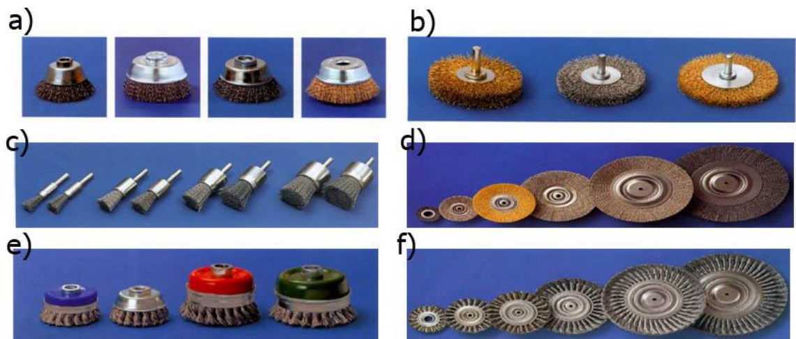
Rys. 2.16. Rodzaje szczotek: a) czołowa garnkowa, b) walcowa trzpieniowa, c) czołowa pędzlowa, d) walcowa beztrzpieniowa, e) czołowa garnkowa z drutem splecionym, f) walcowa z drutem splecionym [123]
