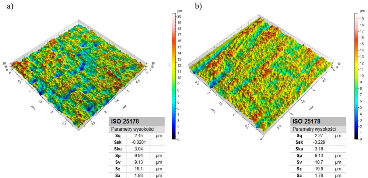
Rys. 4.44. Widok topografii powierzchni po obróbce szczotkowaniem narzędziem S02 stopu magnezu AZ31 ( v_c = 1266 m/min, v_f = 370 mm/min): a) obróbka na sucho, b) obróbka z chłodzeniem
