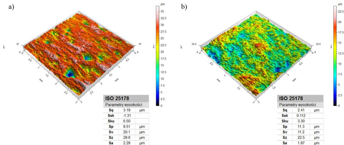
Rys. 4.54. Widok topografii powierzchni po obróbce szczotkowaniem narzędziem S02 stopu aluminium AlSi10Mg ( v_c = 1266 m/min, v_f = 370 mm/min): a) obróbka na sucho, b) obróbka z chłodzeniem
