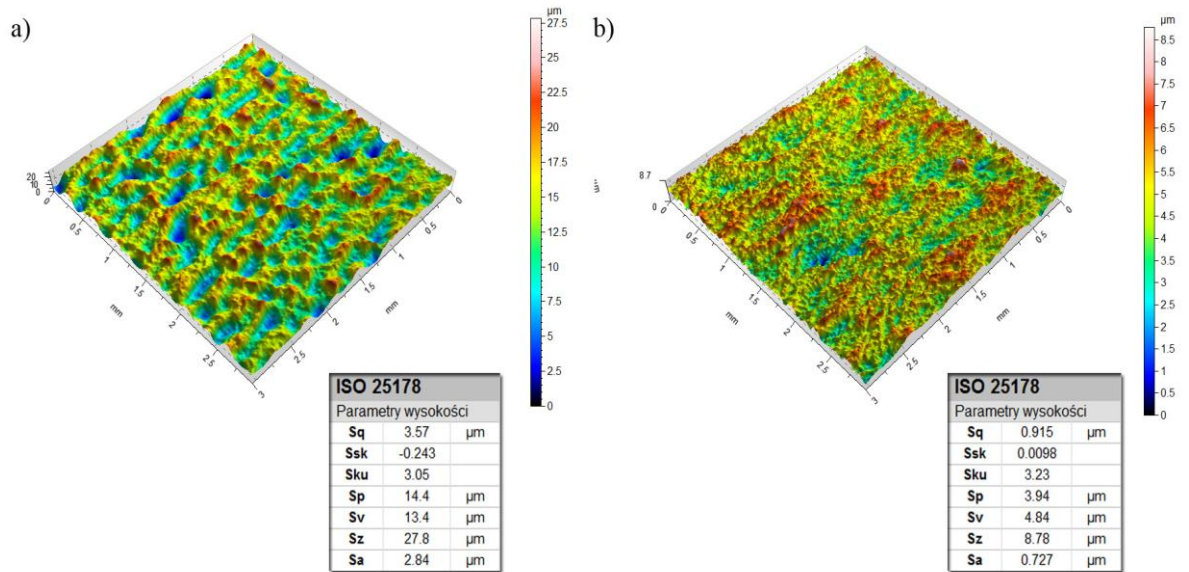
Rys. 4.46. Widok topografii powierzchni po obróbce szczotkowaniem narzędziem M02 stopu magnezu AZ91HP ( v_c = 1689 m/min, v_f = 370 mm/min): a) obróbka na sucho, b) obróbka z chłodzeniem
