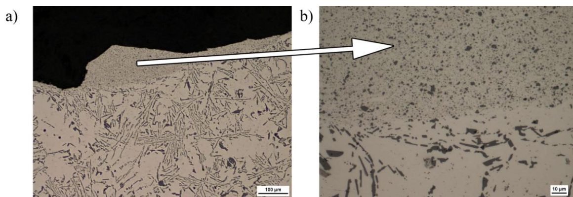
Rys. 4.65. Mikrostruktura stopu AlSi10Mg po obróbce szczotkowaniem (szczotka S03, medium: na sucho)
