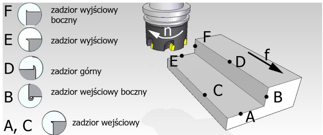
Rys. 2.9. Typy zadziorów powstających podczas frezowania współbieżnego
