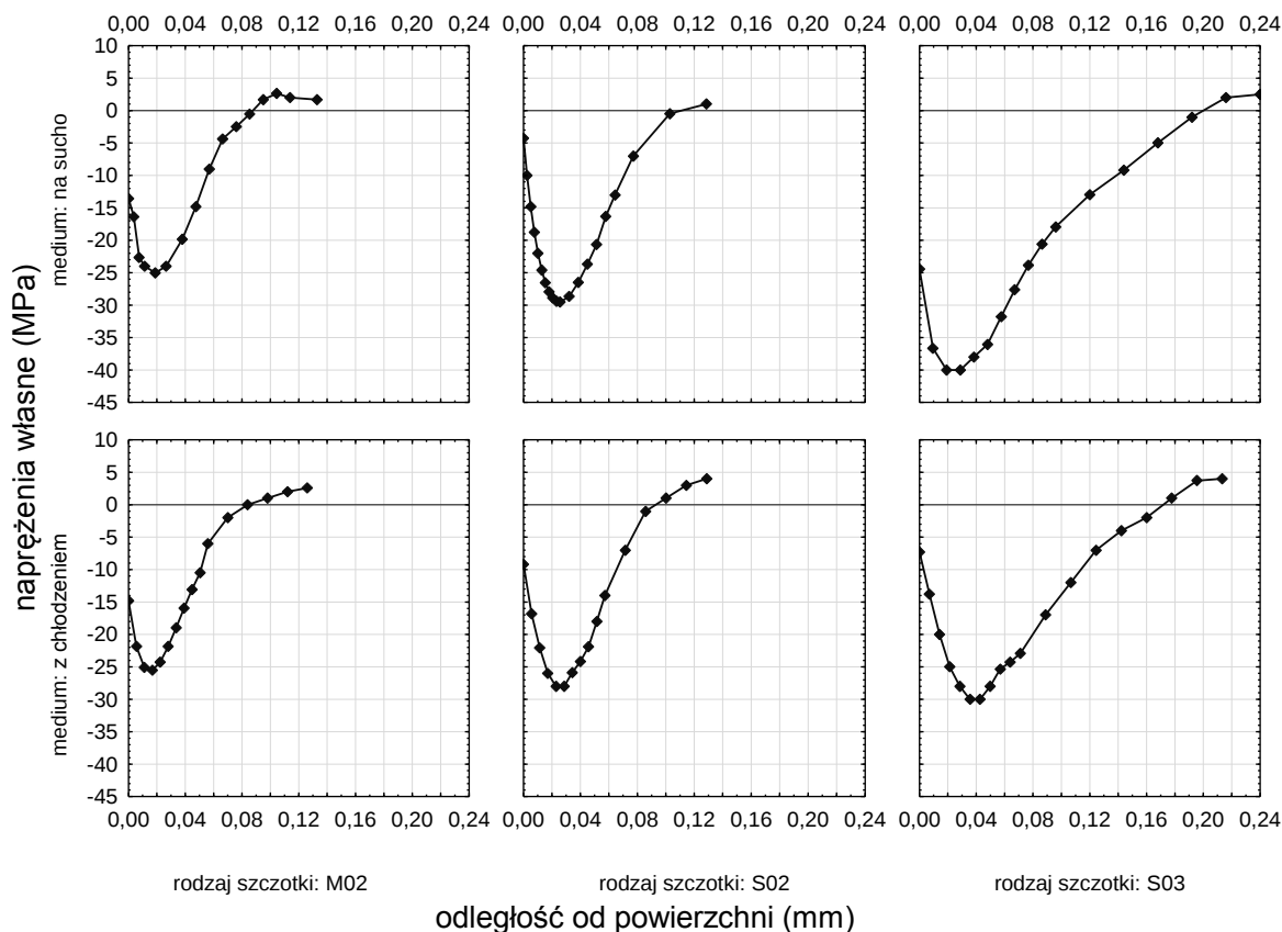
Rys. 4.70. Rozkład naprężeń własnych w funkcji odległości od powierzchni po szczotkowaniu stopu aluminium AlSi10Mg
