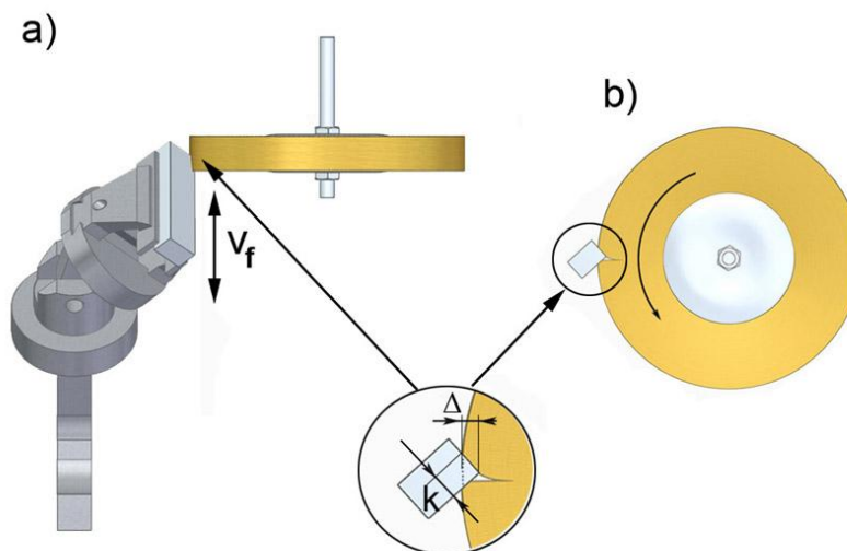
Rys. 4.55. Schemat obróbki szczotkowaniem: a) widok z boku, b) widok z góry
