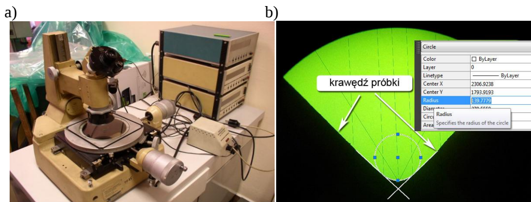
Rys. 4.18. Stanowisko do wyznaczania promienia zaokrąglenia krawędzi: a) mikroskop, b) widok repliki
