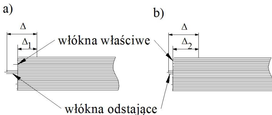
Rys. 4.8. Wpływ długości włókien odstających na średnicę dynamiczną szczotki D_d
