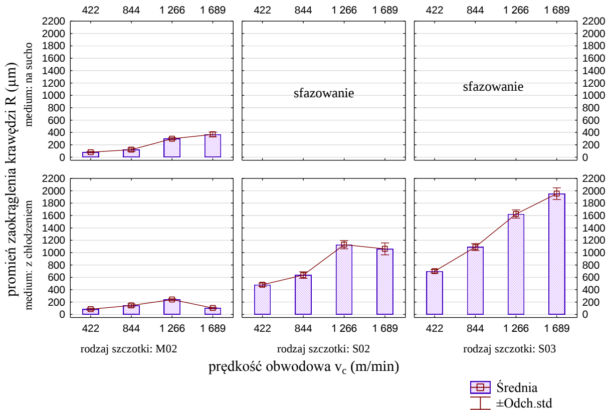
Rys. 4.23. Wpływ prędkości obwodowej na promień zaokrąglenia krawędzi – materiał AlSi10Mg
