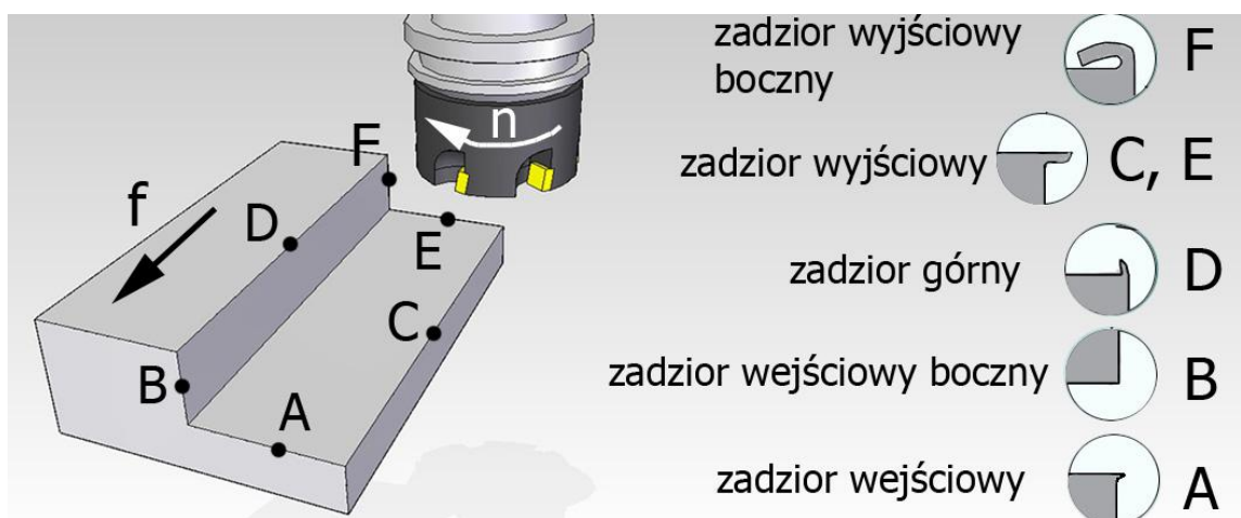
Rys. 2.10. Typy zadziorów powstających podczas frezowania przeciwbieżnego
