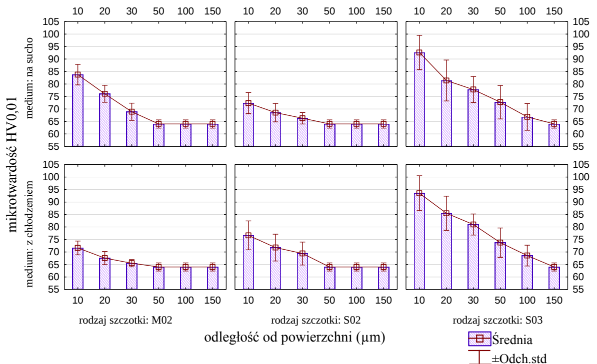
Rys. 4.59. Rozkład mikrotwardości w funkcji odległości od powierzchni po szczotkowaniu stopu magnezu AZ31
