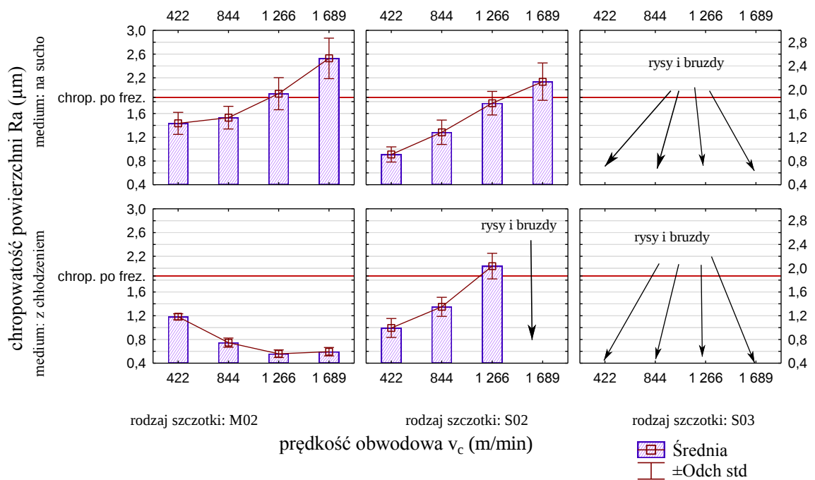
Rys. 4.45. Wpływ prędkości obwodowej w procesie szczotkowania stopu magnezu AZ91HP na chropowatość powierzchni (obróbka poprzedzająca – frezowanie wykończeniowe)
