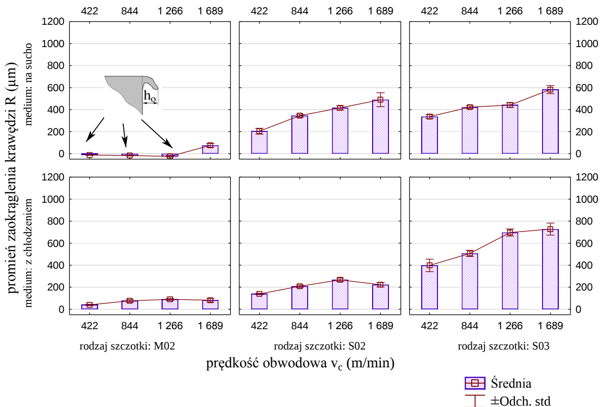
Rys. 4.20. Wpływ prędkości obwodowej na promień zaokrąglenia krawędzi – materiał AZ91HP
