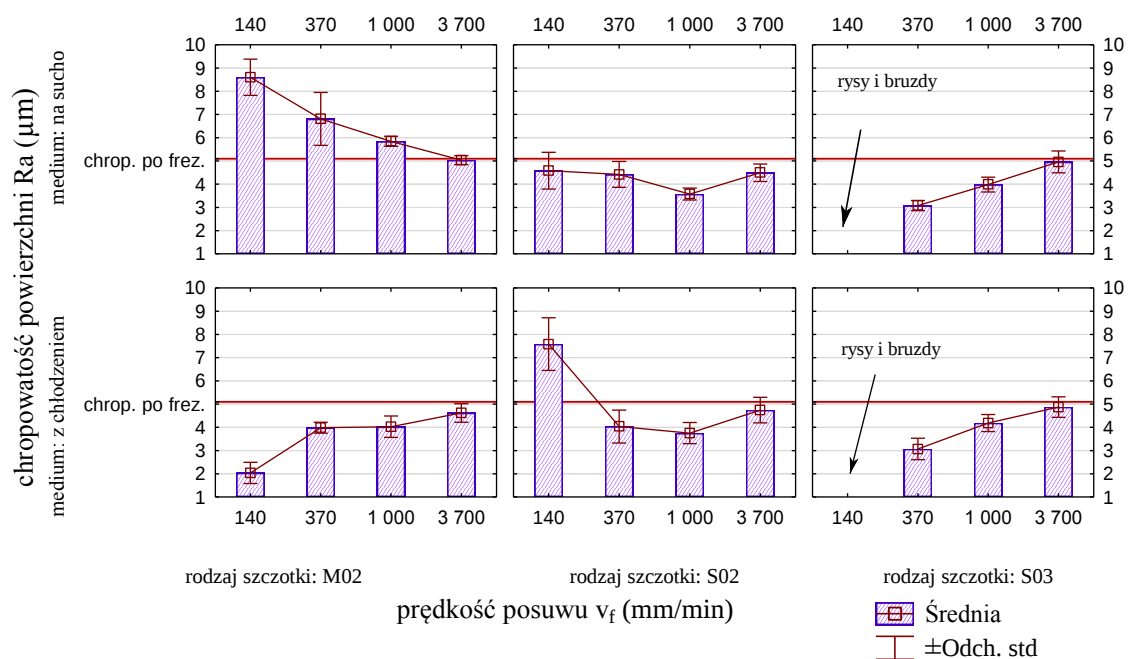
Rys. 4.39. Wpływ prędkości ruchu posuwowego w procesie szczotkowania stopu magnezu AZ91HP na chropowość powierzchni (obróbka poprzedzająca – frezowanie kształtujące)
