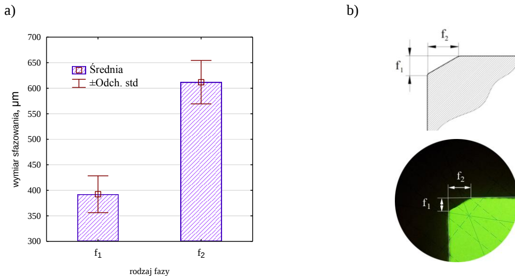
Rys. 4.28. Stan krawędzi – sfazowanie (stop 7075-T651, v_f = 140 mm/min, medium: na sucho): a) wymiary, b) schemat i widok rzeczywisty
