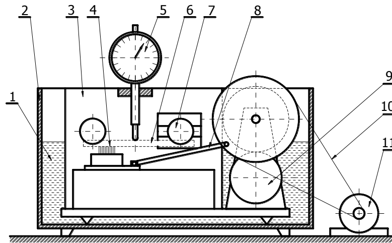
Rys. 4.66. Schemat stanowiska do trawienia próbek płaskich
