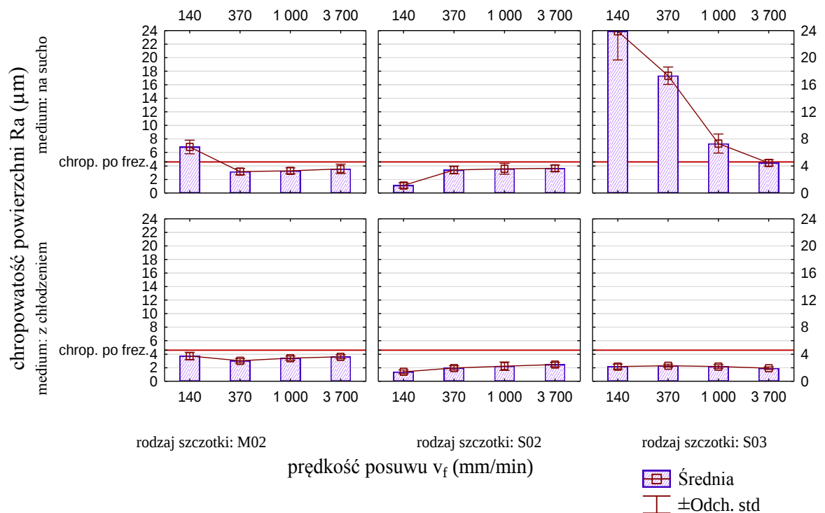
Rys. 4.41. Wpływ prędkości ruchu posuwowego w procesie szczotkowania stopu aluminium AlSi10Mg na chropowatość powierzchni (obróbka poprzedzająca – frezowanie kształtujące)
