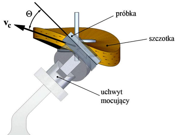
Rys. 4.22. Efekt ugięcia włókien podczas obróbki
