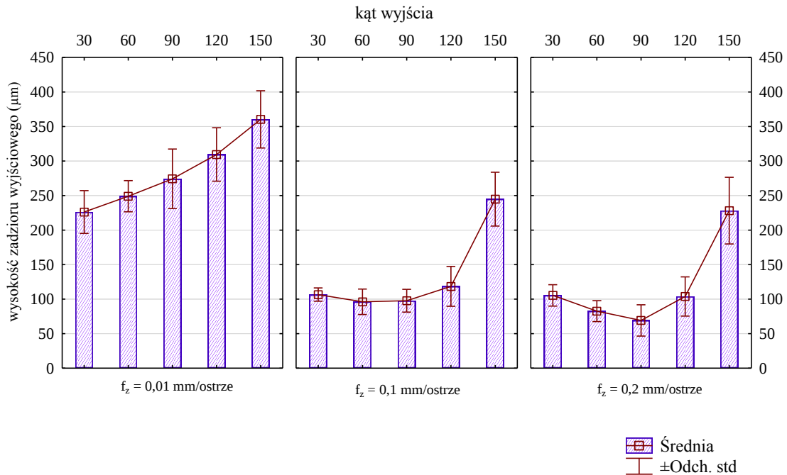
Rys. 4.14. Wpływ posuwu na ostrze skrawania i kąta wyjścia na wysokość zadzioru wyjściowego – materiał AZ91HP
