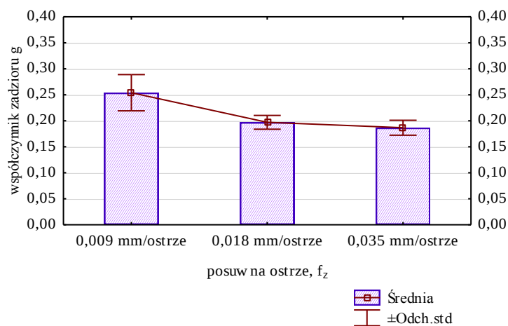
Rys. 4.16. Wpływ posuwu na ostrze na współczynnik zadzioru – stop magnezu AZ91HP
