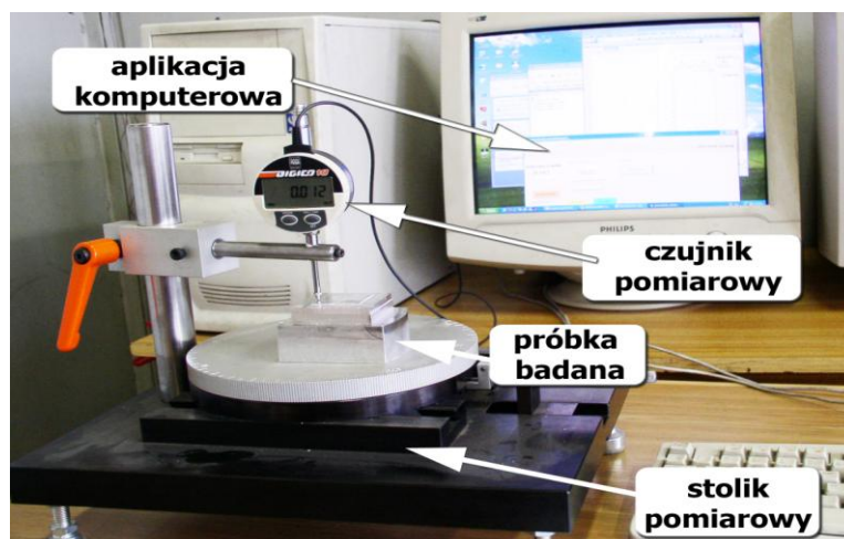
Rys. 4.10. Widok stanowiska do badania wysokości zadziorów
