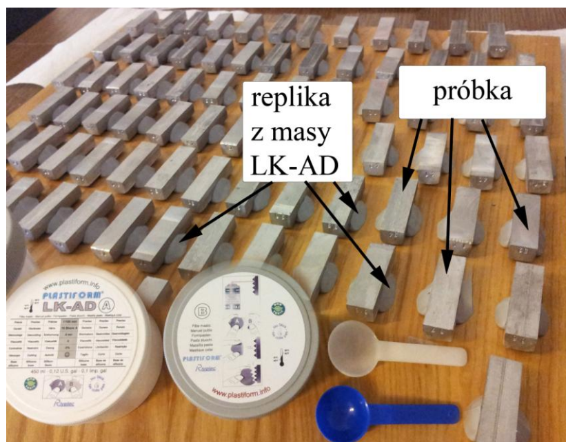
Rys. 4.17. Sposób przygotowania replik
