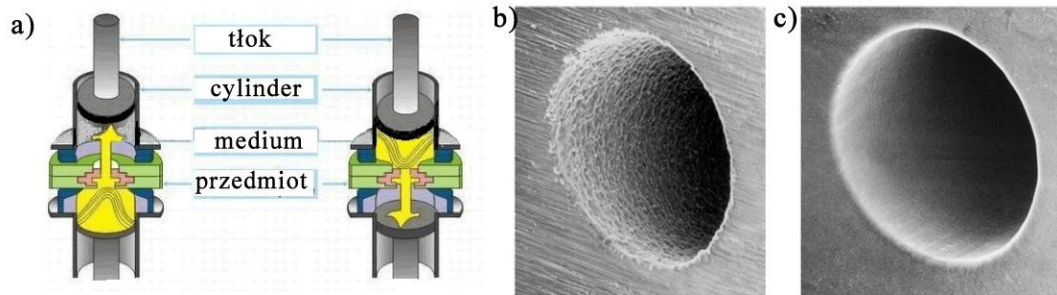
Rys. 2.12. Obróbka przetłoczno - ścierna: a) schemat obróbki dwukierunkowej, b) otwór przed obróbką, c) otwór po obróbce [28]
