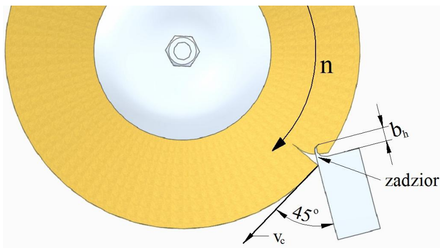
Rys. 4.5. Schemat realizacji pierwszego przejścia szczotkującego
