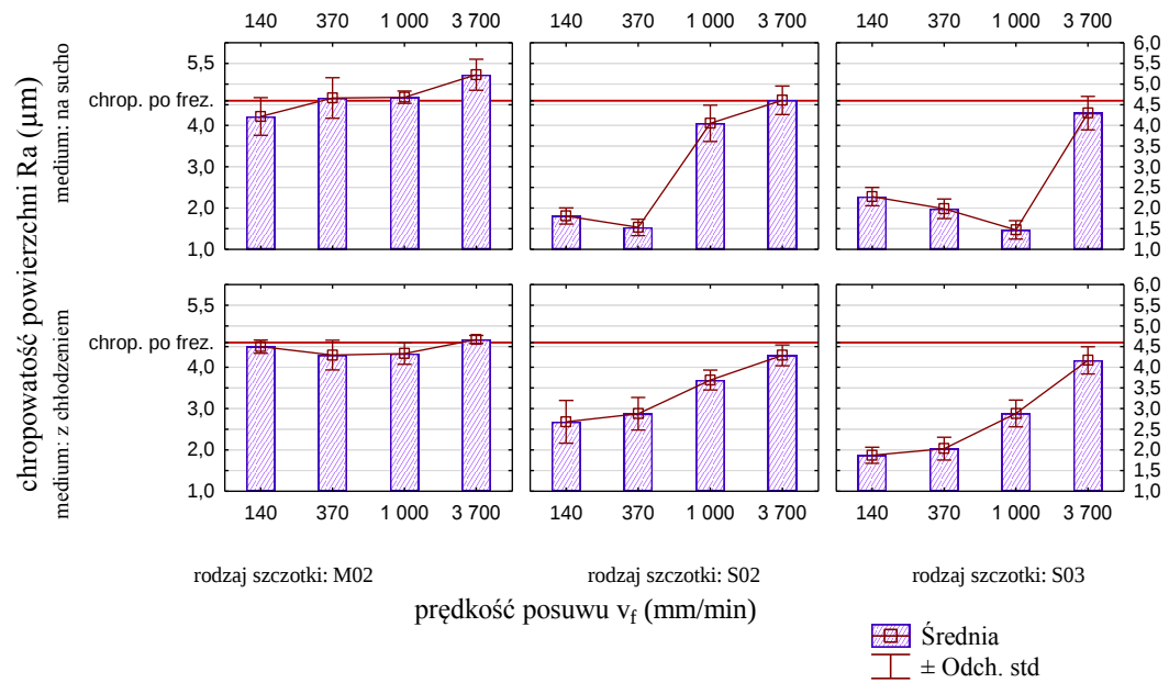
Rys. 4.40. Wpływ prędkości ruchu posuwowego w procesie szczotkowania stopu aluminium 7075-T651 na chropowość powierzchni (obróbka poprzedzająca – frezowanie kształtujące)
