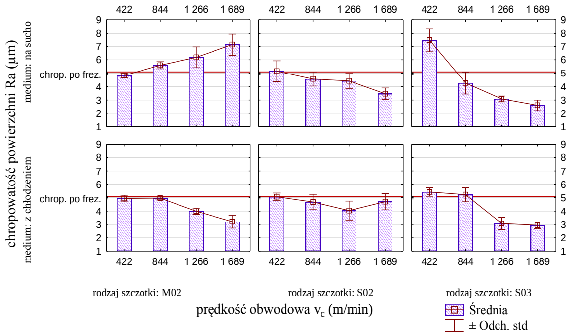
Rys. 4.35. Wpływ prędkości obwodowej w procesie szczotkowania stopu magnezu AZ91HP na chropowość powierzchni (obróbka poprzedzająca – frezowanie kształtujące)
