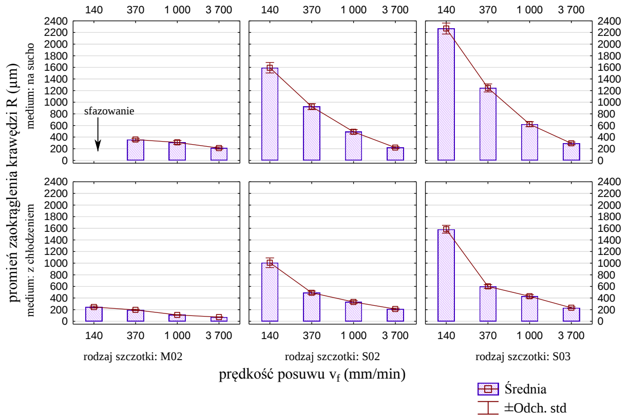
Rys. 4.27. Wpływ prędkości posuwu na promień zaokrąglenia krawędzi – materiał 7075-T651
