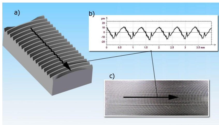
Rys. 4.31. Kierunek pomiaru chropowatości: a) schemat próbki, b) przykładowy profil, c) rzeczywisty widok próbki po frezowaniu [68]
