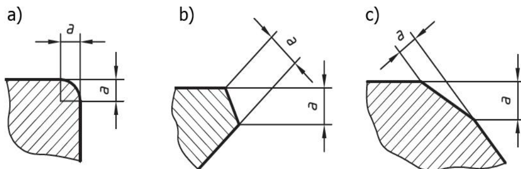
Rys. 2.2. Schemat wymiarowania podcięcia po procesie usuwania zadzioru na krawędzi powstałej przez przecięcie powierzchni przedmiotu pod kątem: a) prostym, b) ostrym, c) rozwartym [118]
