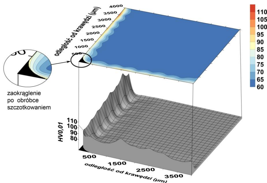
Rys. 4.61. Mapa rozkładu mikrotwardości w obrębie krawędzi po procesie szczotkowania narzędziem S03 w przypadku obróbki na sucho ( v_c = 1266 m/min, v_f = 370 mm/min) – stop magnezu AZ91HP
