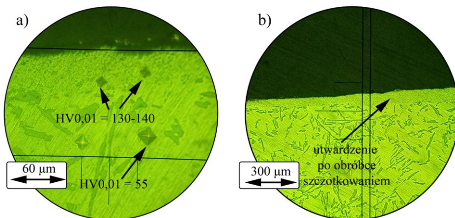
Rys. 4.64. Widok zglądu metalograficznego po obróbce szczotkowaniem stopu AlSi10Mg: a) przykładowe odciski wglębnikiem Vickersa, b) utwardzenie po obróbce szczotkowaniem
