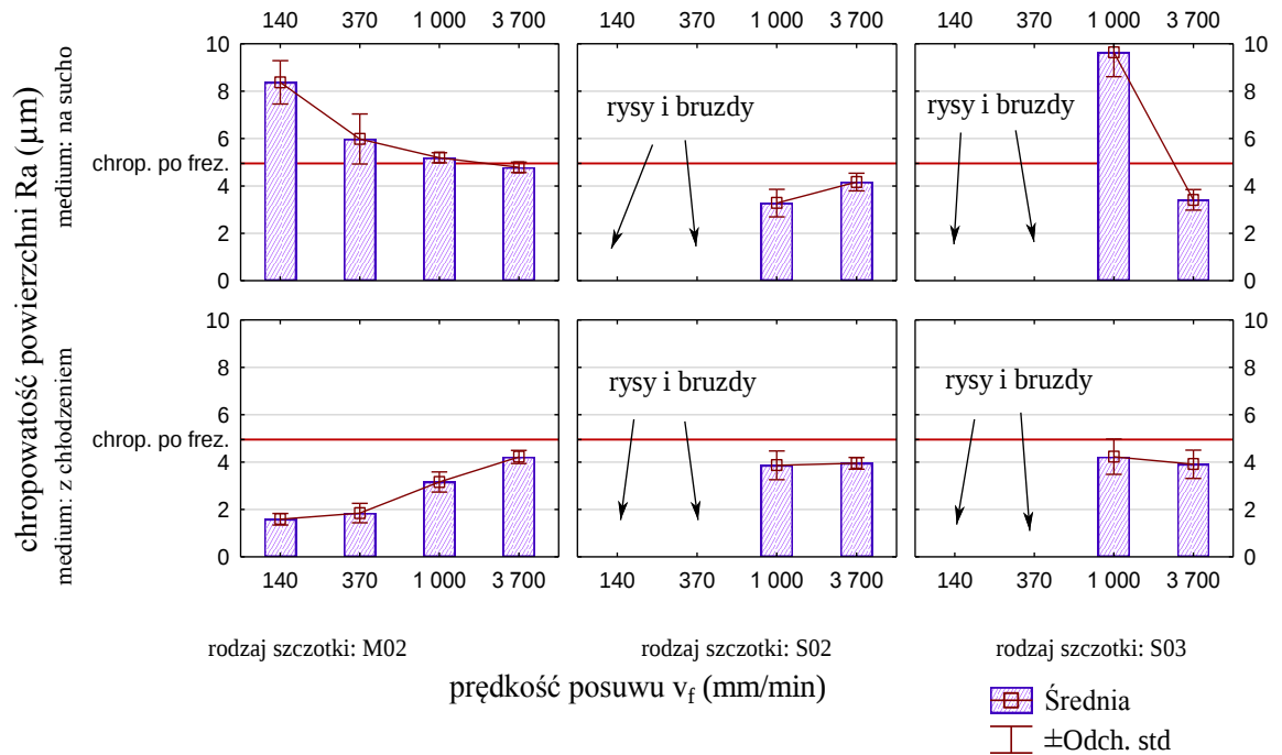
Rys. 4.38. Wpływ prędkości ruchu posuwowego w procesie szczotkowania stopu magnezu AZ31 na chropowość powierzchni (obróbka poprzedzająca – frezowanie kształtujące)
