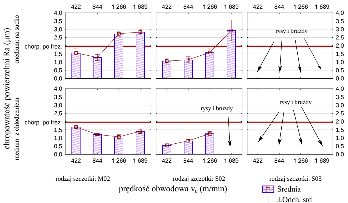
Rys. 4.43. Wpływ prędkości obwodowej w procesie szczotkowania stopu magnezu AZ31 na chropowatość powierzchni (obróbka poprzedzająca – frezowanie wykończeniowe)
