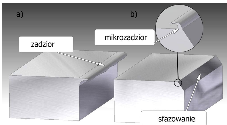
Rys. 2.14. Mikrozadziory po obróbce sztywnymi narzędziami: a) typowy zadziory, b) krawędź sfazowana z "mikrozadziorem" [opracowanie własne]
