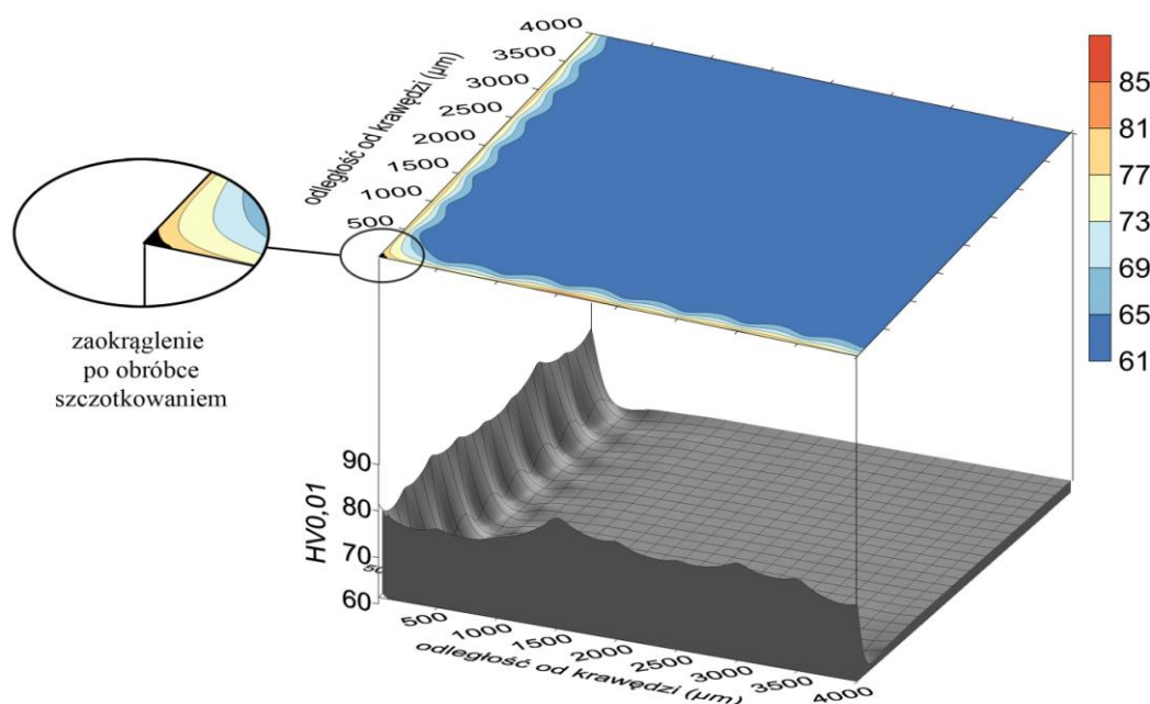
Rys. 4.57. Mapa rozkładu mikrotwardości w obrębie krawędzi po procesie szczotkowania narzędziem M02 w przypadku obróbki na sucho ( v_c = 1266 m/min, v_f = 370 mm/min) – stop magnezu AZ31
