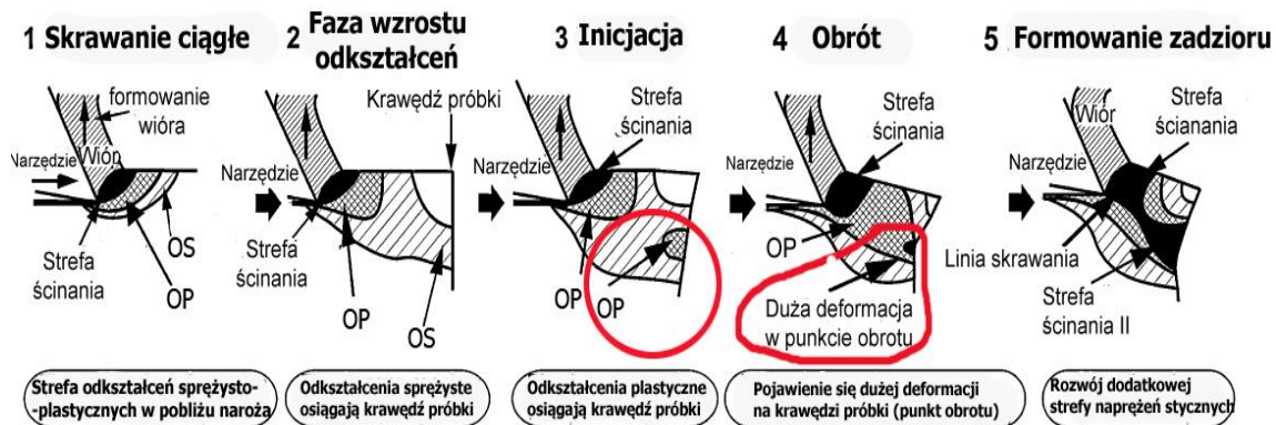
Rys. 2.4. Zjawiska zachodzące przed procesem formowania się zadzioru [40]
