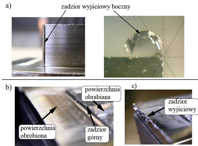
Rys. 4.9. Rodzaje zadziorów analizowanych podczas eksperymentu (badania własne)
