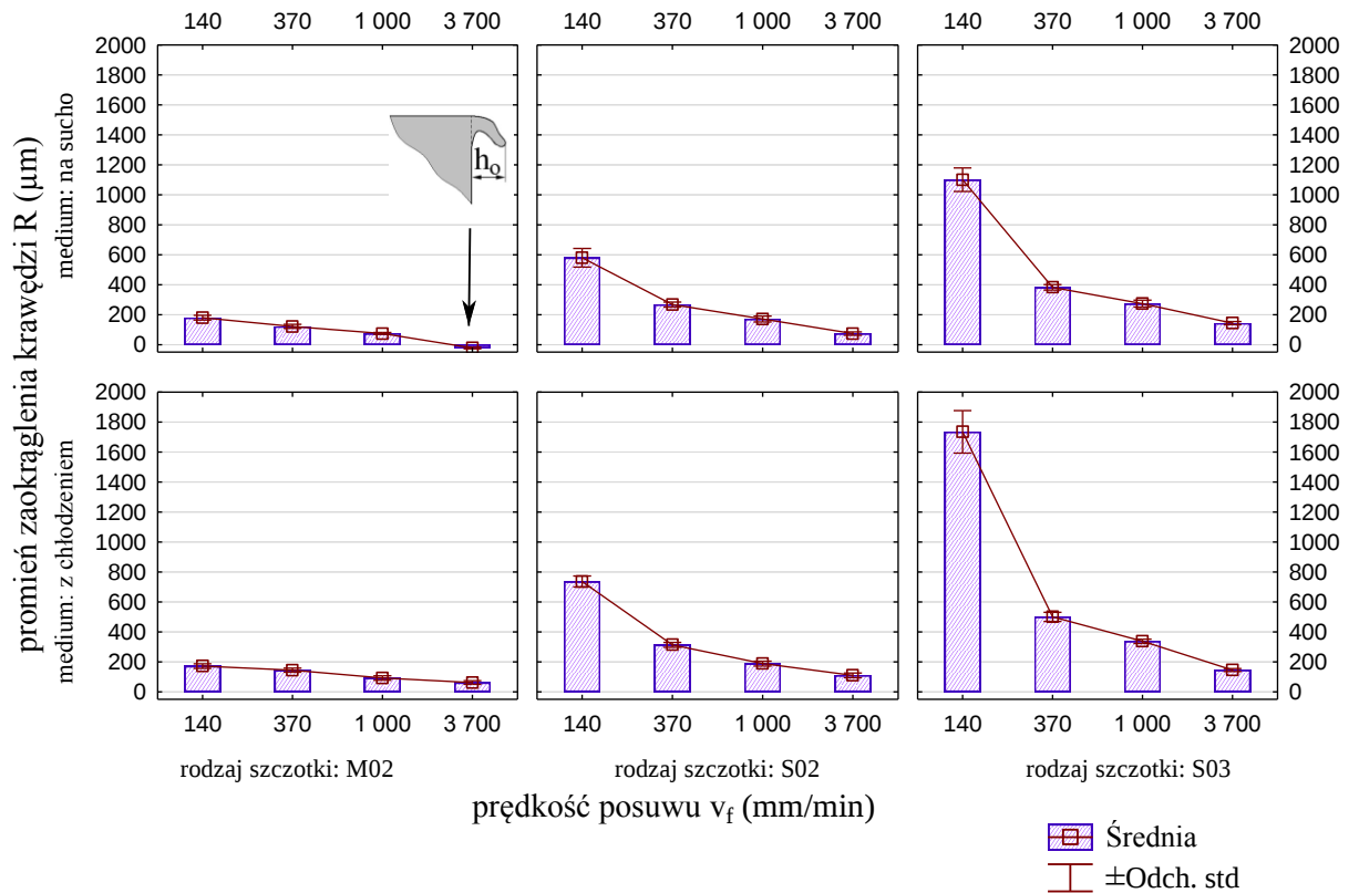
Rys. 4.24. Wpływ prędkości posuwu na promień zaokrąglenia krawędzi – materiał AZ31
