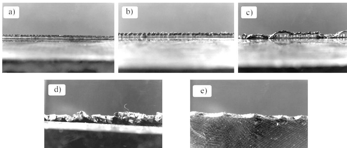
Rys. 2.7. Typy zadziorów wg [60]
