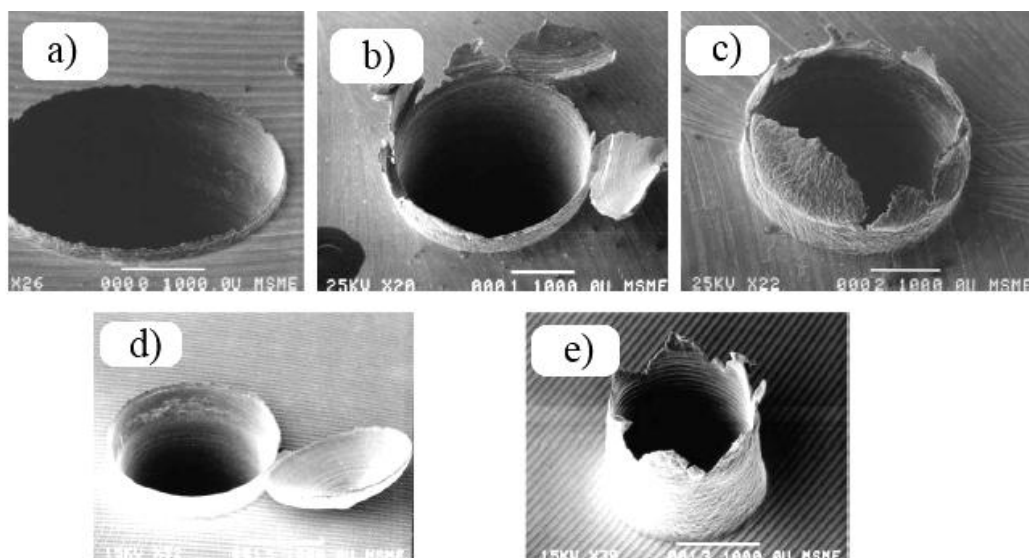
Rys. 2.8. Rodzaje zadziorów występujących podczas wiercenia: a, d) jednolity, b) przejściowy, c, e) koronowy [47]
