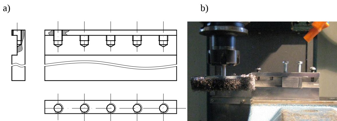
Rys. 4.2. Uchwyt do szczotkowania walcowego: a) schemat, b) widok rzeczywisty
