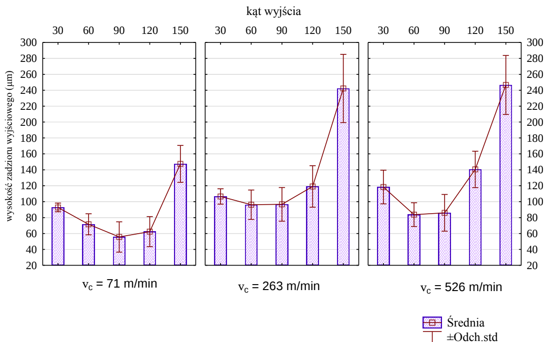
Rys. 4.13. Wpływ prędkości skrawania i kąta wyjścia na wysokość zadzioru wyjściowego - materiał AZ91HP
