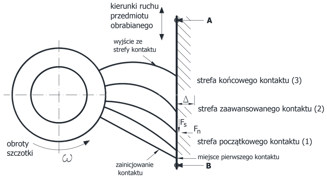
Rys. 2.17. Ugięcie pojedynczego włókna w fazie początkowej, przejściowej i wyjścia ze strefy kontaktu [96]
