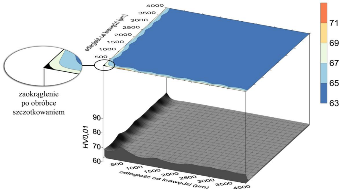
Rys. 4.58. Mapa rozkładu mikrotwardości w obrębie krawędzi po procesie szczotkowania narzędziem M02 w przypadku obróbki z chłodzeniem ( v_c = 1266 \text{ m/min} , v_f = 370 \text{ mm/min} ) – stop magnezu AZ31
