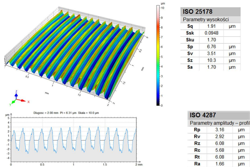
Rys. 4.42. Powierzchniowa mapa po obróbce frezowaniem – stop aluminium 7075-T651
