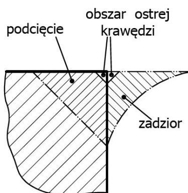
Rys. 2.1. Stany krawędzi zewnętrznej [118]
