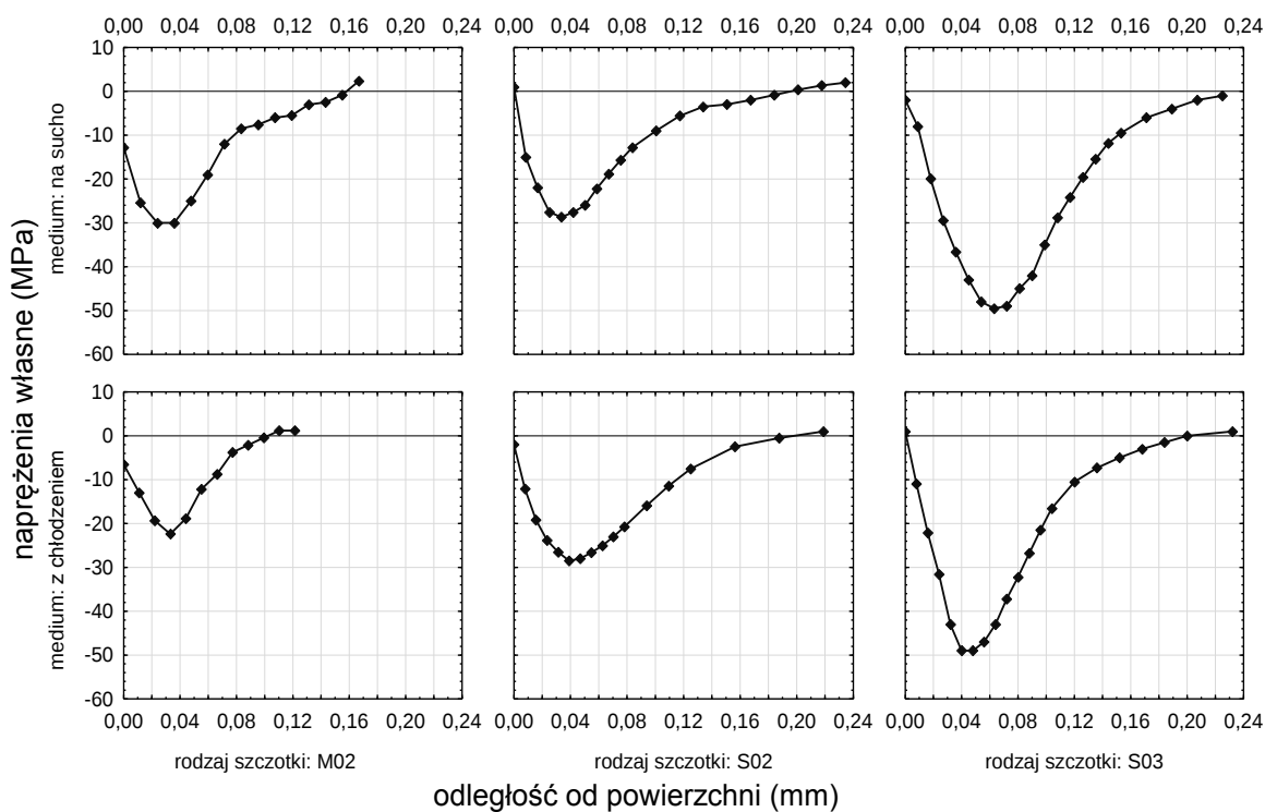
Rys. 4.68. Rozkład naprężeń własnych w funkcji odległości od powierzchni po szczotkowaniu stopu magnezu AZ91HP
