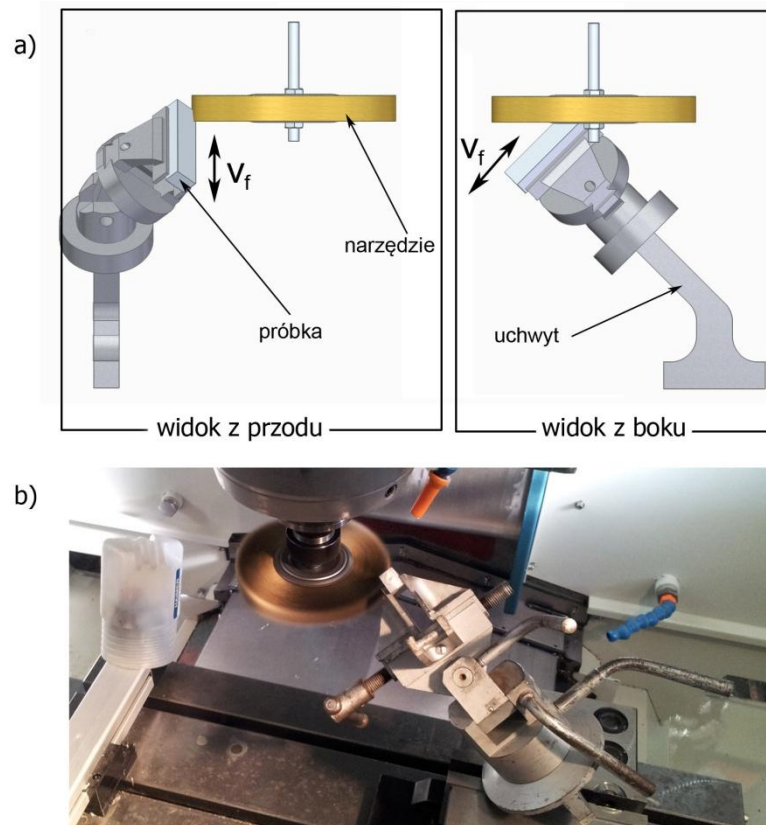
Rys. 4.3. Uchwyt do szczotkowania krawędzi: a) schemat stanowiska, b) widok rzeczywisty
