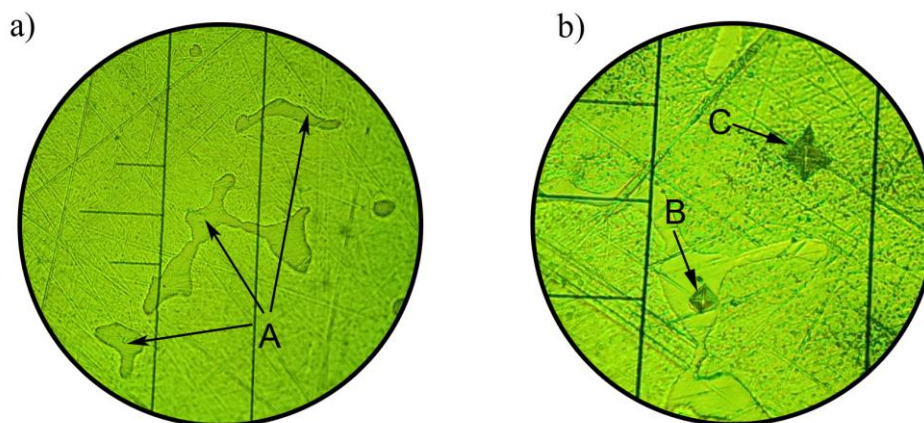
Rys. 4.60. Zgład metalograficzny stopu magnezu AZ91HP: a) faza Mg_{17}Al_{12} , b) odciski wglębnika Vickersa
