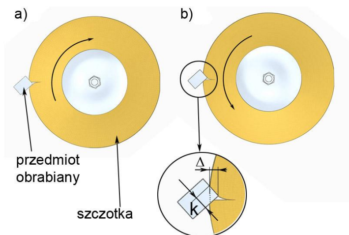
Rys. 4.4. Dwukierunkowa realizacja procesu usuwania zadziorów: a) pierwsze przejście – obroty prawe, b) drugie przejście – obroty lewe
