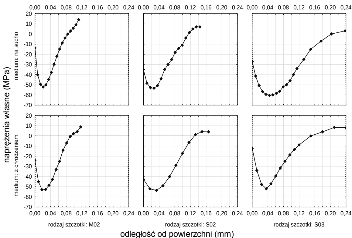
Rys. 4.69. Rozkład naprężeń własnych w funkcji odległości od powierzchni po szczotkowaniu stopu aluminium
