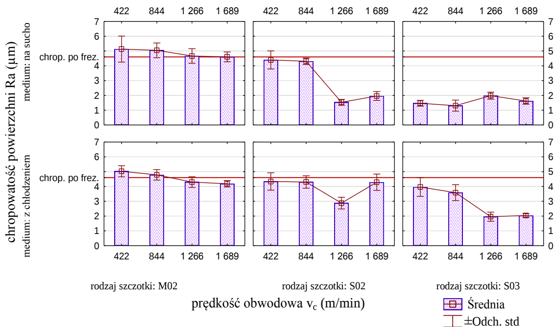
Rys. 4.36. Wpływ prędkości obwodowej w procesie szczotkowania stopu aluminium 7075-T651 na chropowość powierzchni (obróbka poprzedzająca – frezowanie kształtujące)
