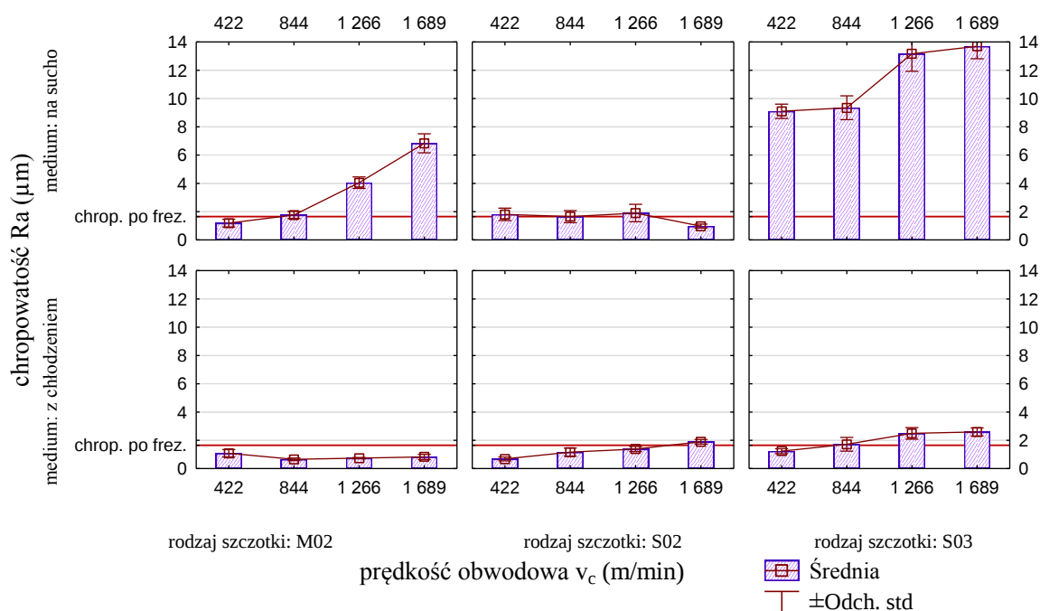
Rys. 4.48. Wpływ prędkości obwodowej w procesie szczotkowania stopu aluminium AlSi10Mg na chropowatość powierzchni (obróbka poprzedzająca – frezowanie wykończeniowe)
