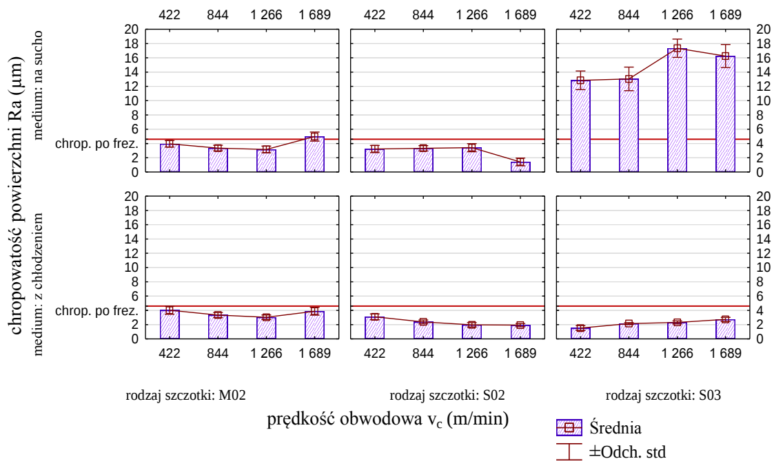
Rys. 4.37. Wpływ prędkości obwodowej w procesie szczotkowania stopu aluminium AlSi10Mg na chropowatość powierzchni (obróbka poprzedzająca – frezowanie kształtujące)
