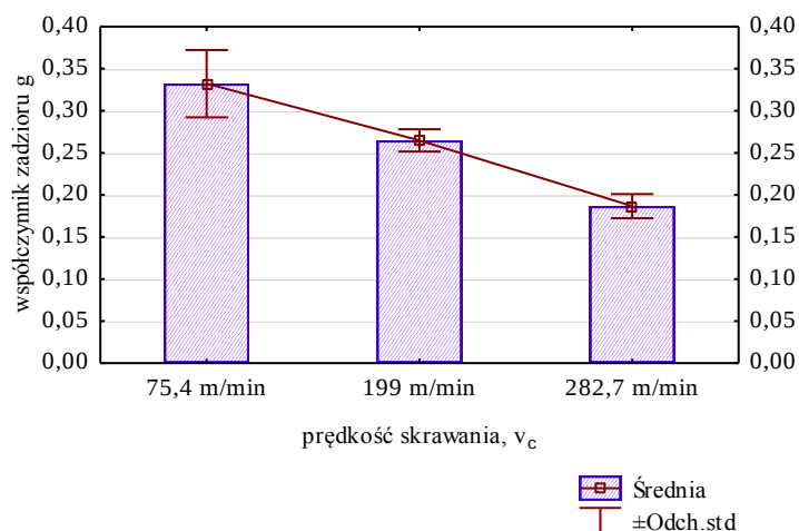
Rys. 4.15. Wpływ prędkości skrawania na współczynnik zadzioru – materiał AZ91HP
