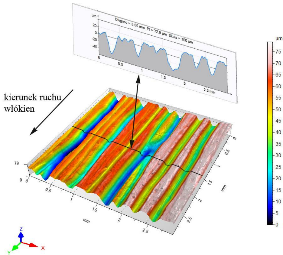
Rys. 4.33. Bruzdy po obróbce szczotkowaniem – narzędzie S03, medium: z chłodzeniem, v_c = 422 m/min, v_f = 370 mm/min
