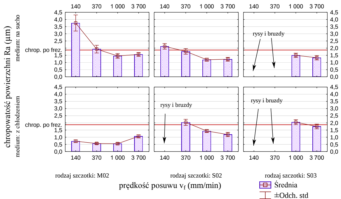
Rys. 4.50. Wpływ prędkości ruchu posuwowego w procesie szczotkowania stopu magnezu AZ91HP na chropowatość powierzchni (obróbka poprzedzająca – frezowanie wykończeniowe)
