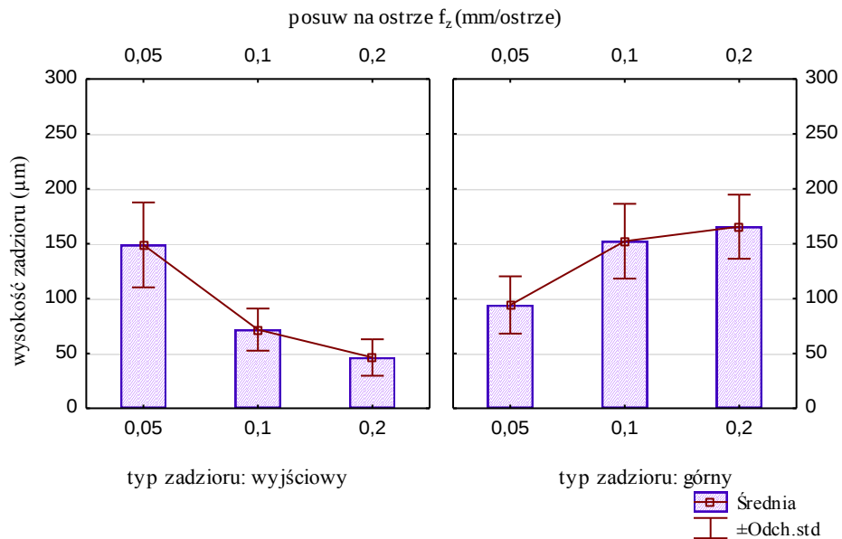
Rys. 4.12. Wpływ posuwu na ostrze na wysokość zadzioru wyjściowego oraz górnego – stop aluminium 7075-T651
