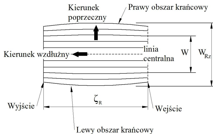
Rys. 2.18. Kierunkowość struktury po obróbce szczotkowaniem płaskiej powierzchni [98]
