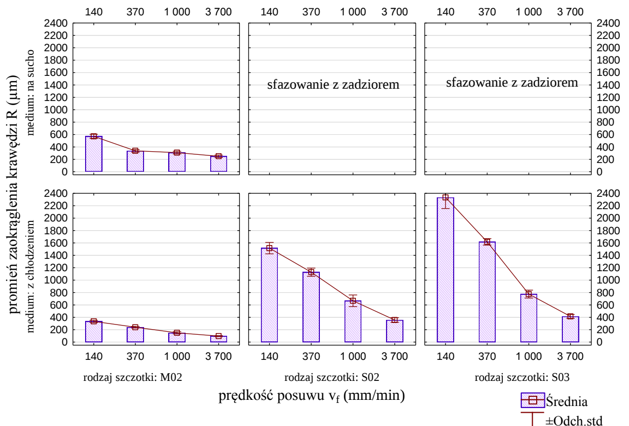
Rys. 4.30. Wpływ prędkości posuwu na promień zaokrąglenia krawędzi – materiał AlSi10Mg
