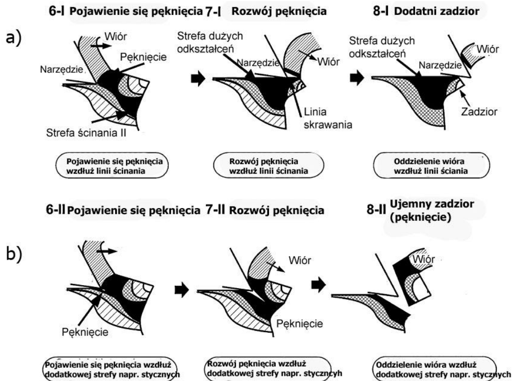
Rys. 2.5. Zjawiska zachodzące podczas procesu formowania się zadziorów: a) materiały plastyczne, b) materiały kruche [40]
