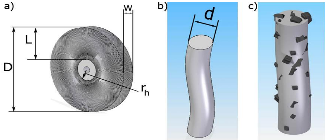
Rys. 2.15. Budowa szczotki: a) wymiary charakterystyczne, b) włókno monolityczne, c) włókno kompozytowe [opracowanie własne]
