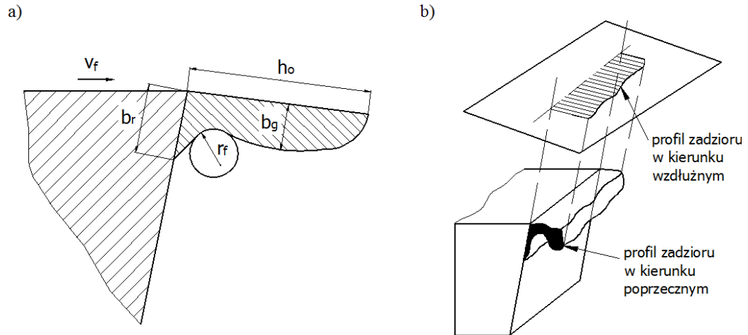
Rys. 2.11. Geometria zadzioru: a) przekrój poprzeczny, b) profil wzdłużny [89]
