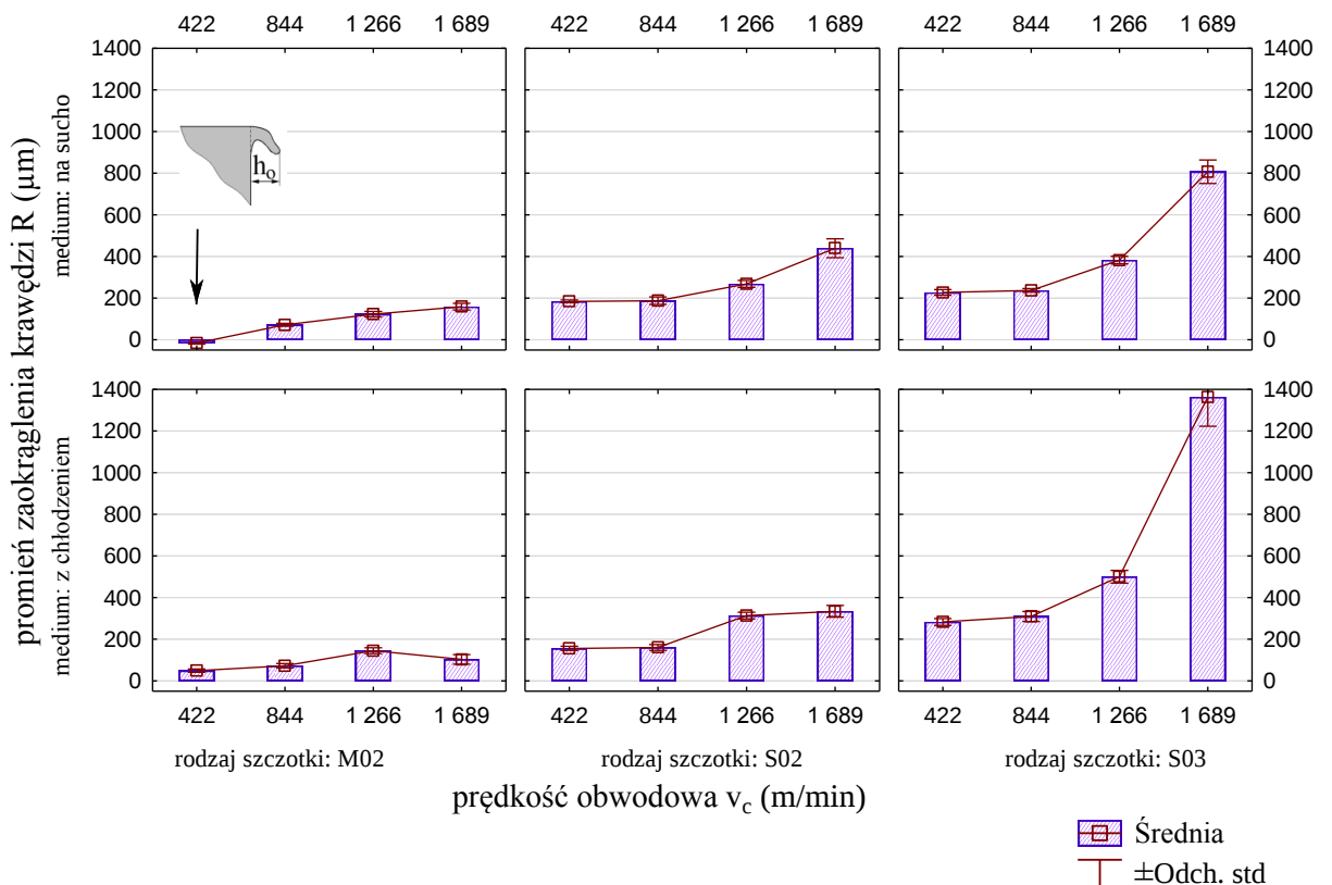
Rys. 4.19. Wpływ prędkości obwodowej na promień zaokrąglenia krawędzi – materiał AZ31
