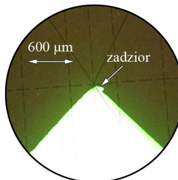
Rys. 4.25. Zadzior po obróbce szczotkowaniem – stop AZ91HP, szczotka M02, medium: na sucho, v_f = 1000 mm/min
