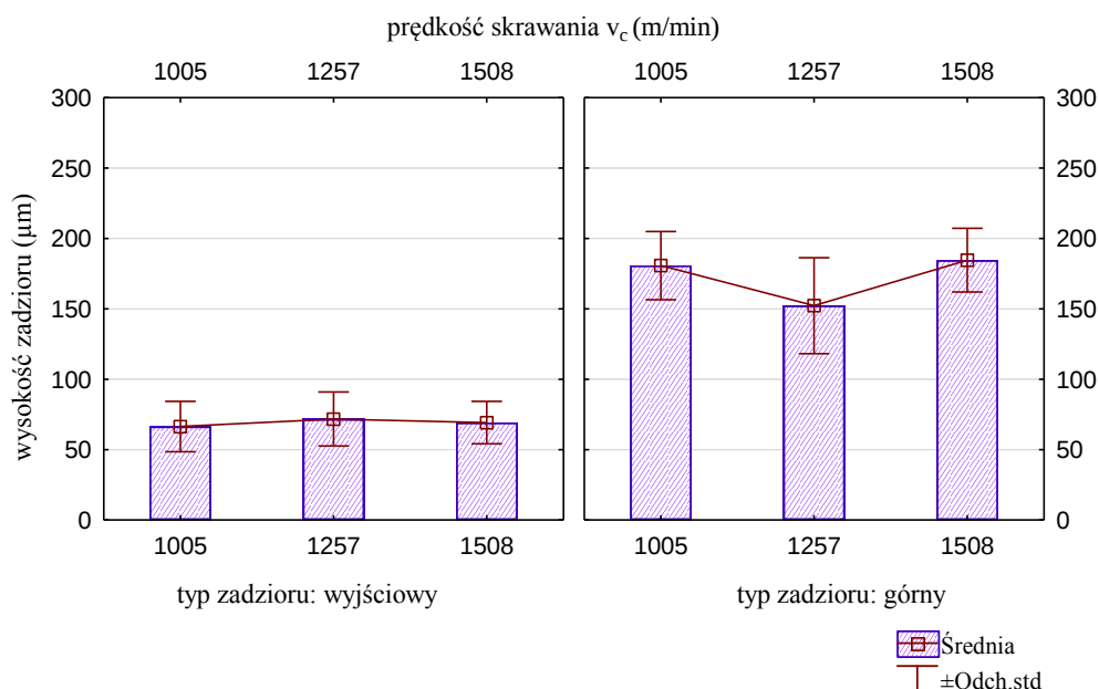
Rys. 4.11. Wpływ prędkości skrawania v_c na wysokość zadzioru wyjściowego oraz górnego – stop aluminium 7075-T651
