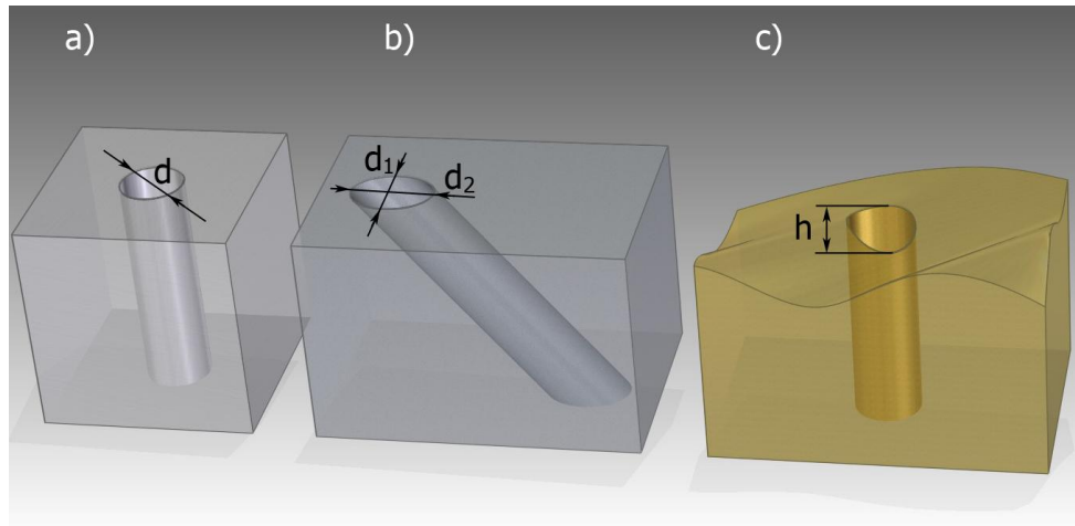
Rys. 2.13. Krawędzie po wykonaniu otworów: a) oś otworu prostopadła do powierzchni, b) oś otworu pochylona w stosunku do powierzchni, c) otwór na powierzchni krzywoliniowej [opracowanie własne]
