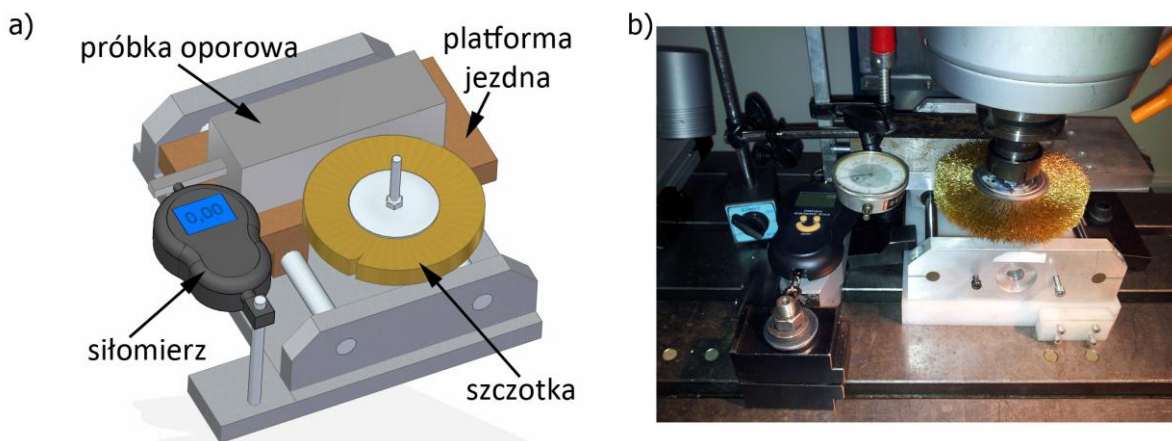
Rys. 4.7. Stanowisko do pomiaru średnicy dynamicznej szczotek: a) model stanowiska, b) widok rzeczywisty
