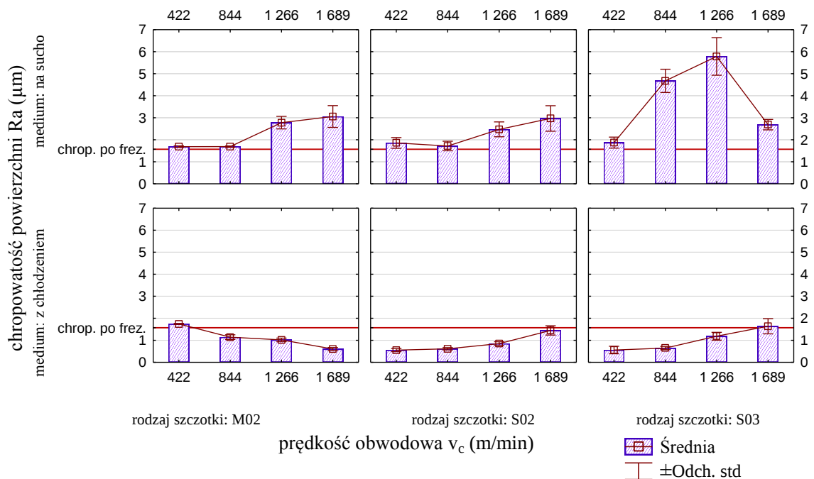
Rys. 4.47. Wpływ prędkości obwodowej w procesie szczotkowania stopu aluminium 7075-T651 na chropowatość powierzchni (obróbka poprzedzająca – frezowanie wykończeniowe)
