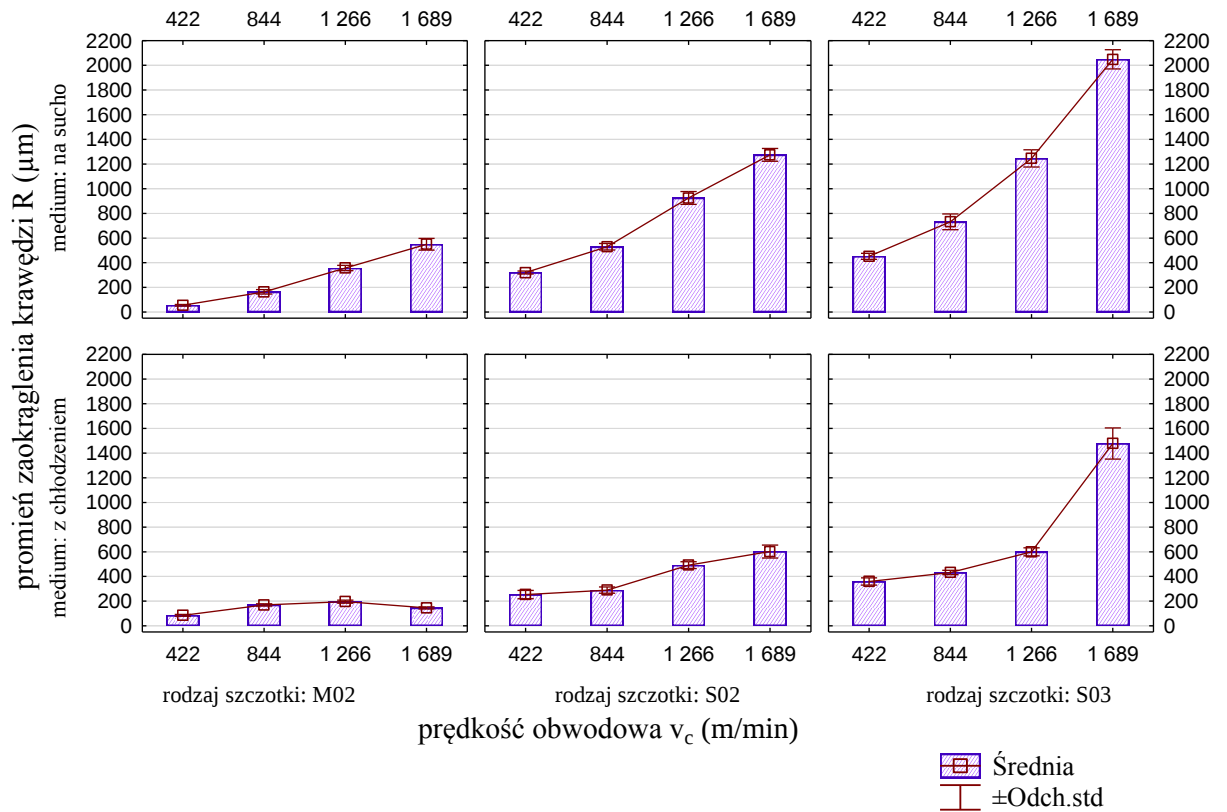
Rys. 4.21. Wpływ prędkości obwodowej na promień zaokrąglenia krawędzi – materiał 7075-T651
