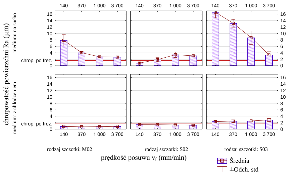
Rys. 4.53. Wpływ prędkości ruchu posuwowego w procesie szczotkowania stopu aluminium AlSi10Mg na chropowatość powierzchni (obróbka poprzedzająca – frezowanie wykończeniowe)
