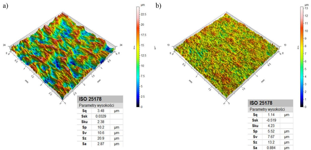
Rys. 4.52. Widok topografii powierzchni po obróbce szczotkowaniem narzędziem S02 stopu aluminium 7075-T651 ( v_f = 370 mm/min, v_c = 1266 m/min): a) obróbka na sucho, b) obróbka z chłodzeniem
