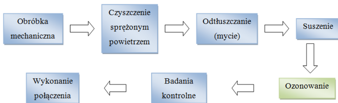
Rys. 1.6. Schemat blokowy typowej technologii łączenia z wykorzystaniem ozonowania
