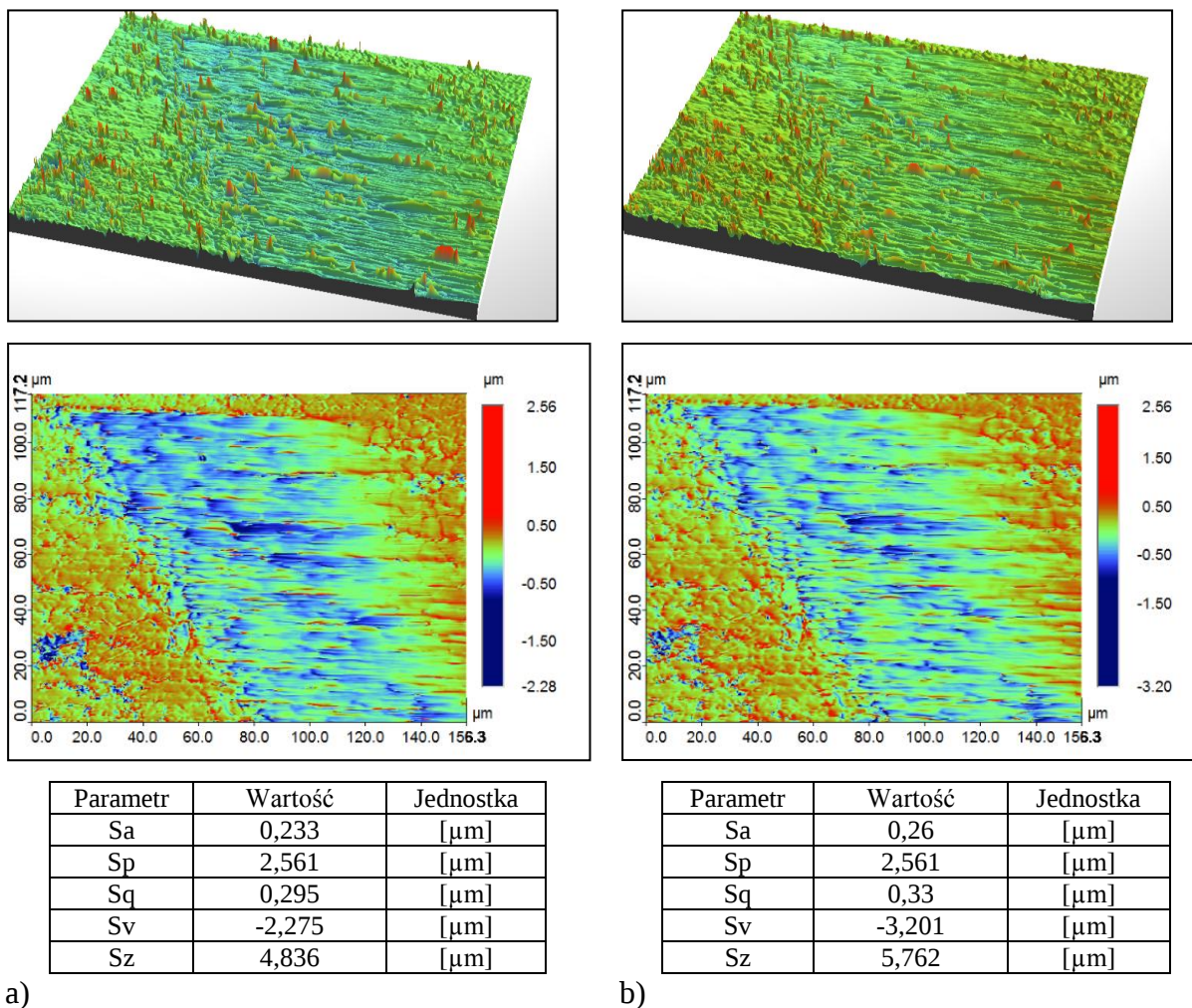
Rys. 5.6. Zdjęcie powierzchni oraz wartości wybranych parametrów chropowatości próbki ze stali 316L: a) przed ozonowaniem, b) po ozonowaniu
