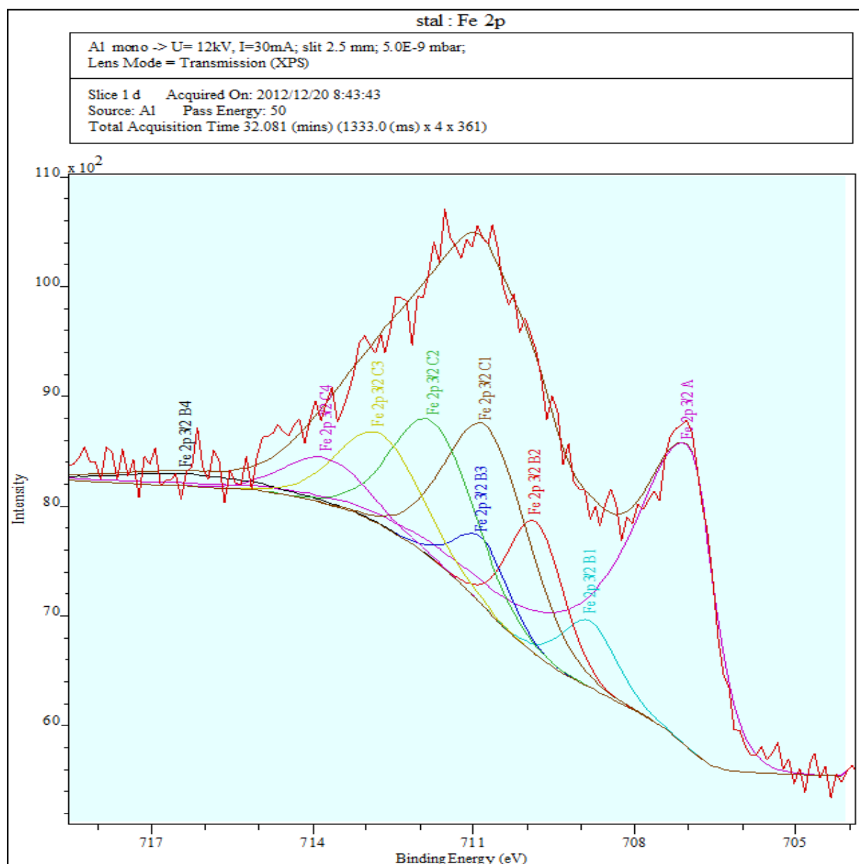
Rys. 5.22. Procedura dekonwolucji złożonego pasma przejść elektronowych Fe2p 3/2 w widmie XPS
