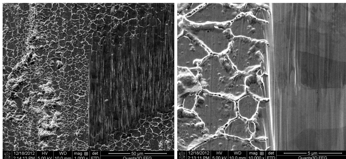
Rys. 5.11. Topografia powierzchni stali 316L przed ozonowaniem
