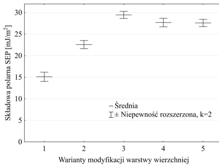
Rys. 5.39. Składowa polarna SEP stali 316L po obróbce mechanicznej dla różnych warunków ozonowania (patrz str. 102)
