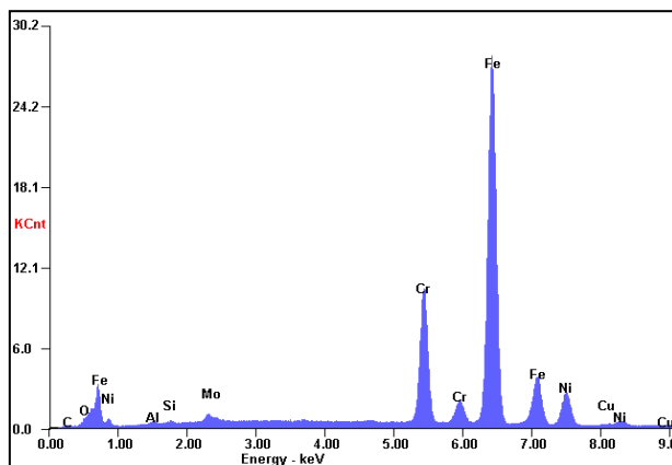
Rys. 5.14. Widmo EDX próbki stali 316L po ozonowaniu oraz wynik analizy elementarnej obszaru
