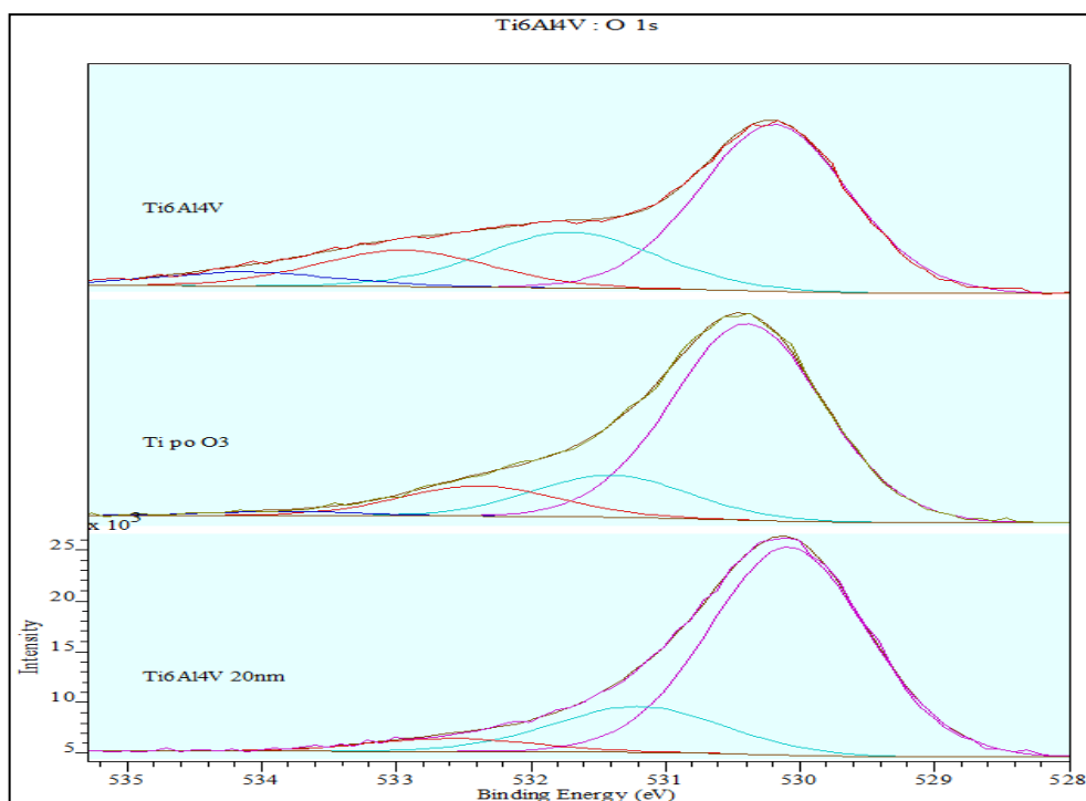
Rys. 5.33. Dekonwolucja widma XPS pasma O1s
