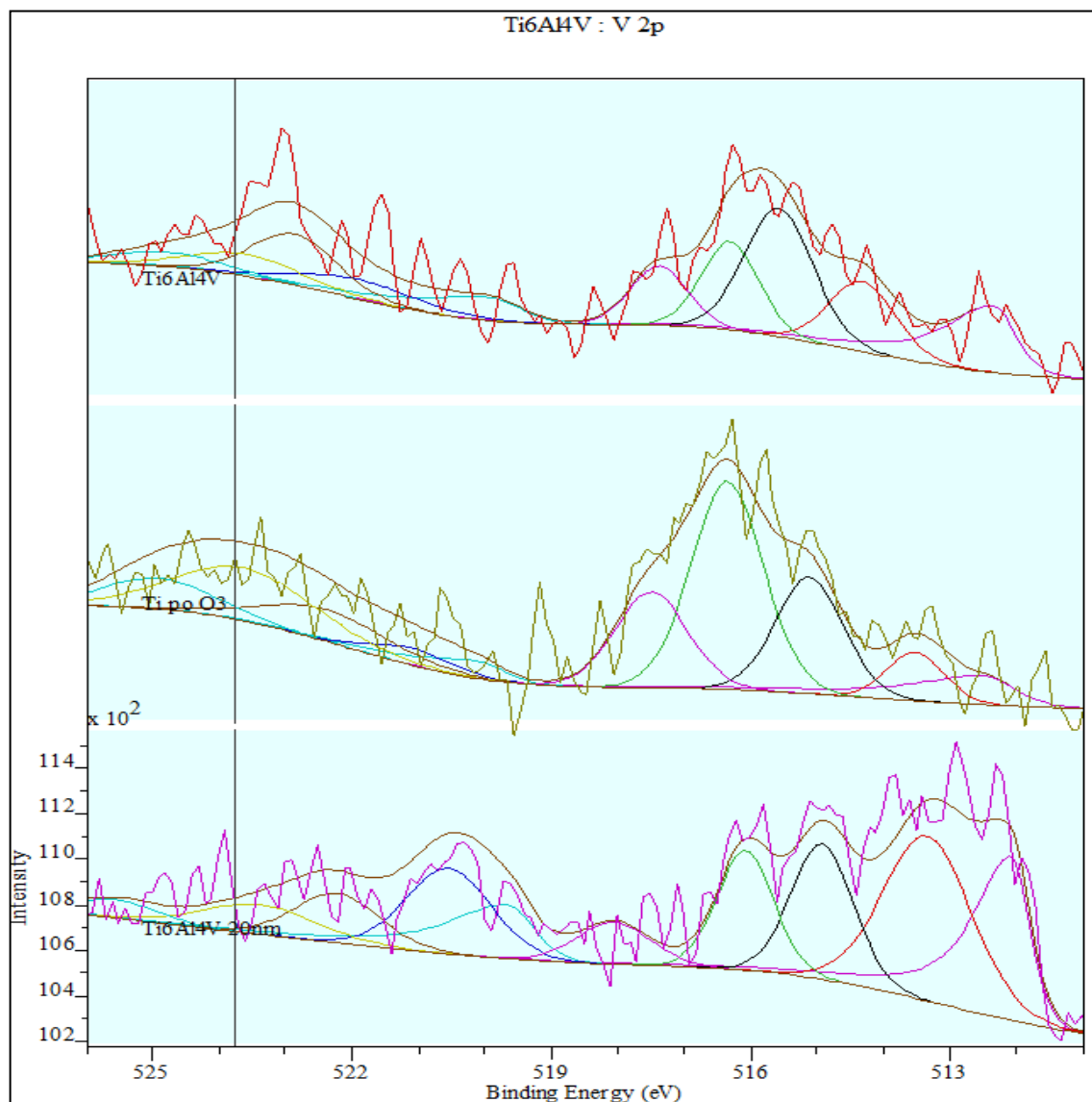
Rys. 5.31. Wpływ ozonowania na widmo XPS na podstawie przejść V2p
