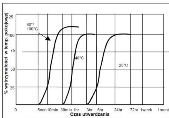
Rys. 3.1. Wytrzymałość na ścinanie w zależności od czasu utwardzania [133]
