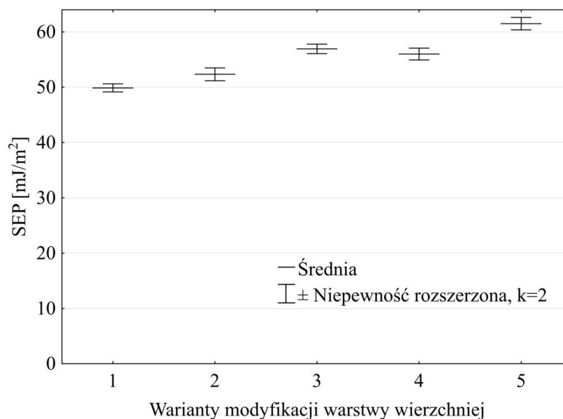
Rys. 5.40. Swobodna energia powierzchniowa stali 316L przed obróbką mechaniczną dla warunków ozonowania przedstawionych na str. 104
