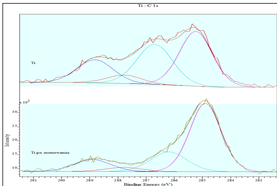
Rys. 5.34. Dopasowanie widma XPS pasma C1s
