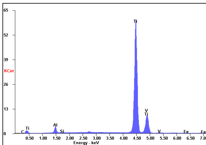
Rys. 5.18. Widmo EDX próbki stopu tytanu Ti-6Al-4V przed ozonowaniem oraz wyniki analizy elementarnej obszaru
