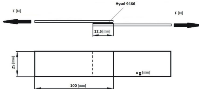
Rys. 3.3. Próbką jednozakładowa - schemat połączenia klejowego: g - grubość elementów klejonych, F - siła obciążająca połączenie
