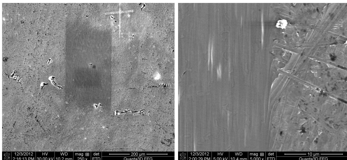
Rys. 5.17. Topografia powierzchni stopu tytanu Ti-6Al-4V po ozonowaniu
