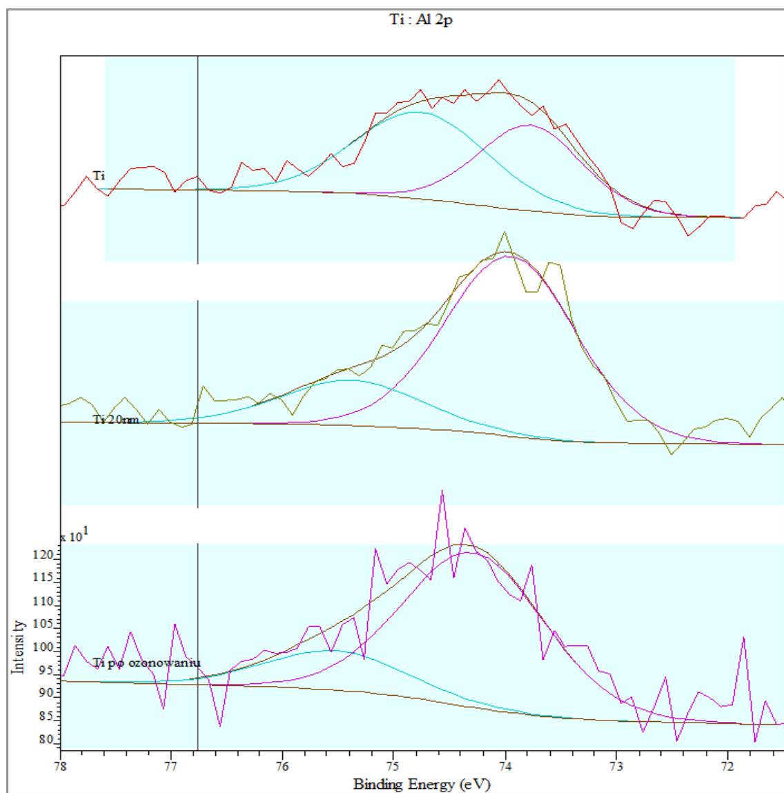
Rys. 5.32. Dekonwolucja widma XPS pasma Al2p: stop tytanu przed ozonowaniem (Ti), stop tytanu po czyszczeniu jonowym (Ti 20nm) oraz stop tytanu po ozonowaniu (Ti po ozonowaniu)
