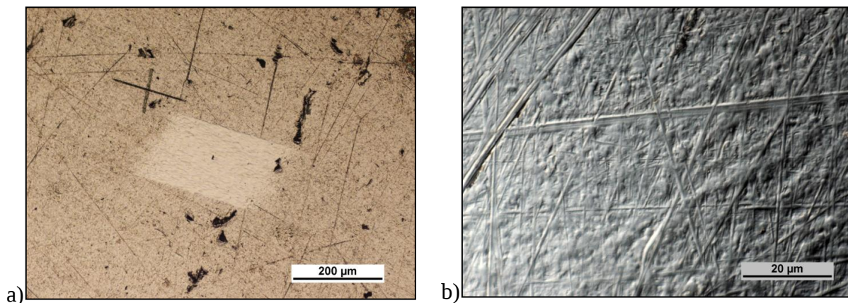
Rys. 5.3. Powierzchnia stopu tytanu Ti-6Al-4V: a) w świetle spolaryzowanym przy powiększeniu 50x, b) obraz DIC przy powiększeniu 1000x
