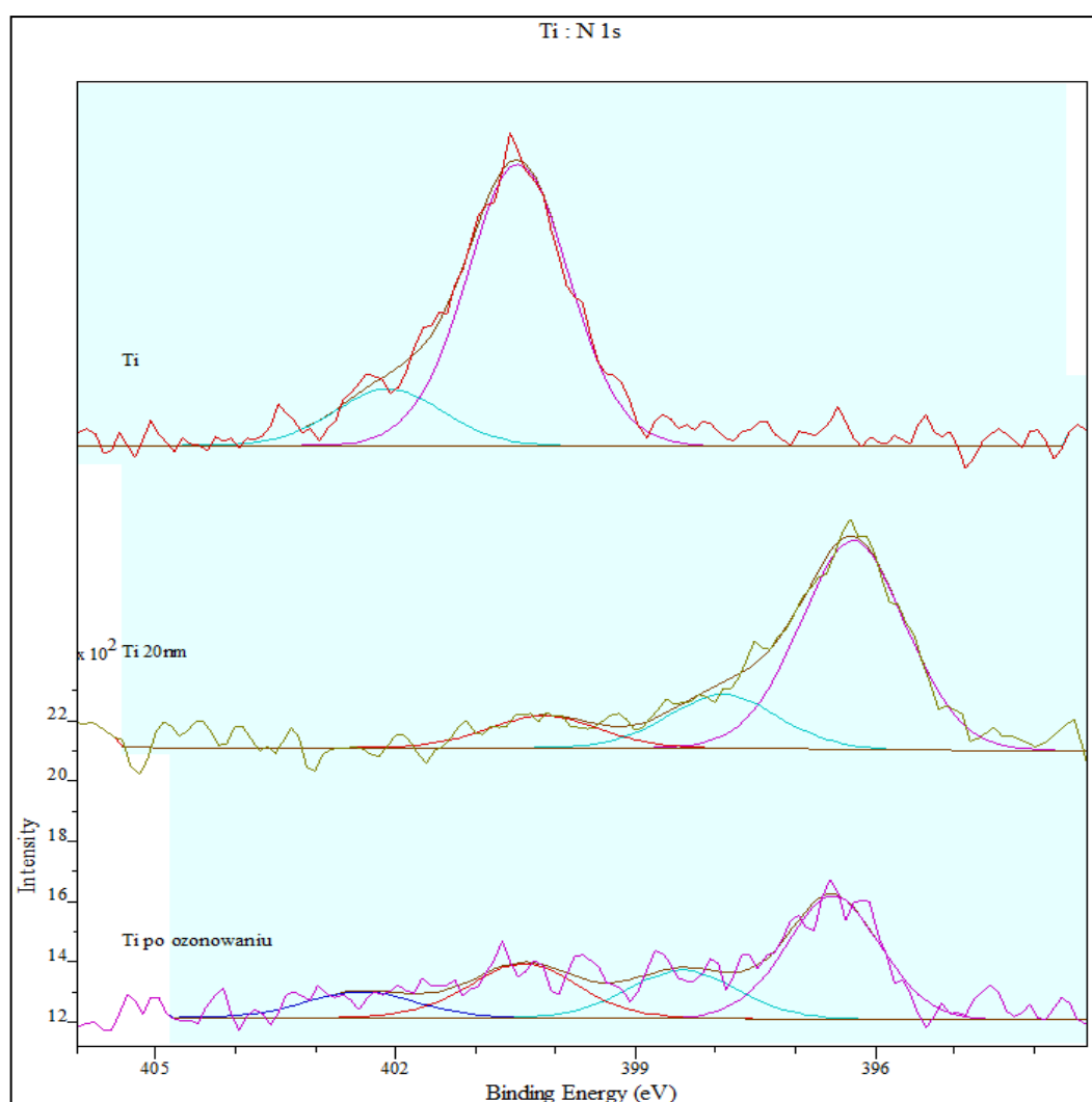
Rys. 5.35. Widmo XPS fotoelektronów azotu w próbce stopu tytanu
