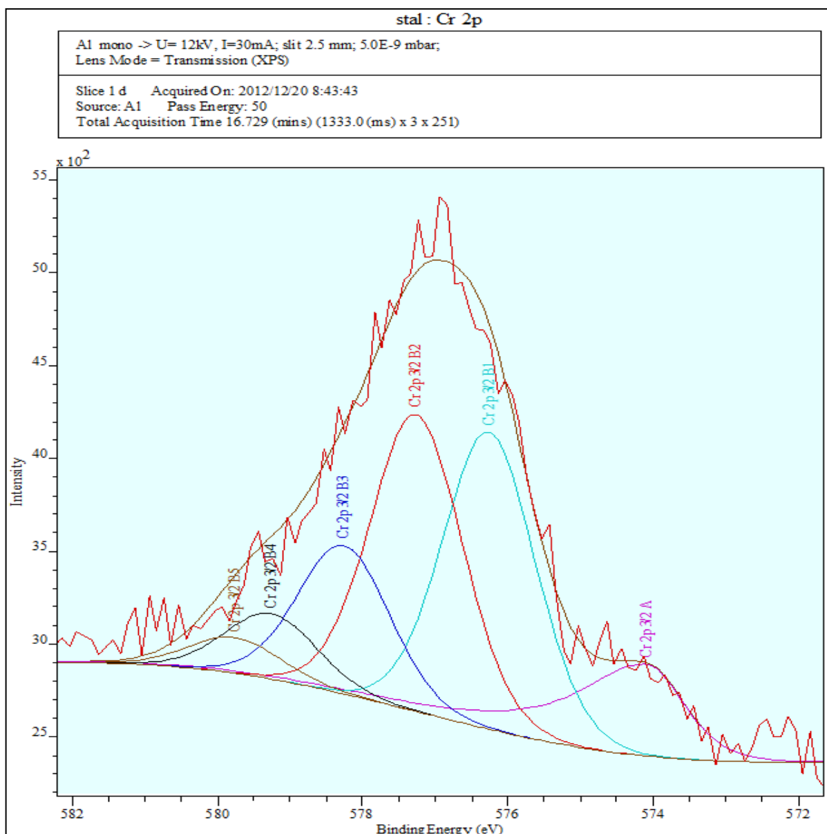
Rys. 5.23. Procedura dekonwolucji złożonego pasma gałęzi przejść elektronowych \text{Cr} 2p_{3/2} w widmie XPS
