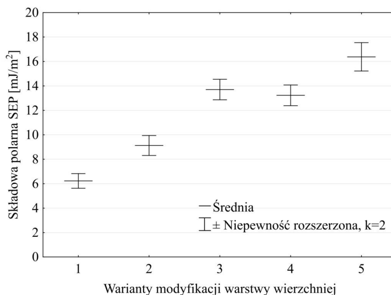
Rys. 5.41. Składowa polarna SEP stali 316L przed obróbką mechaniczną dla różnych warunków ozonowania (patrz str. 104)
