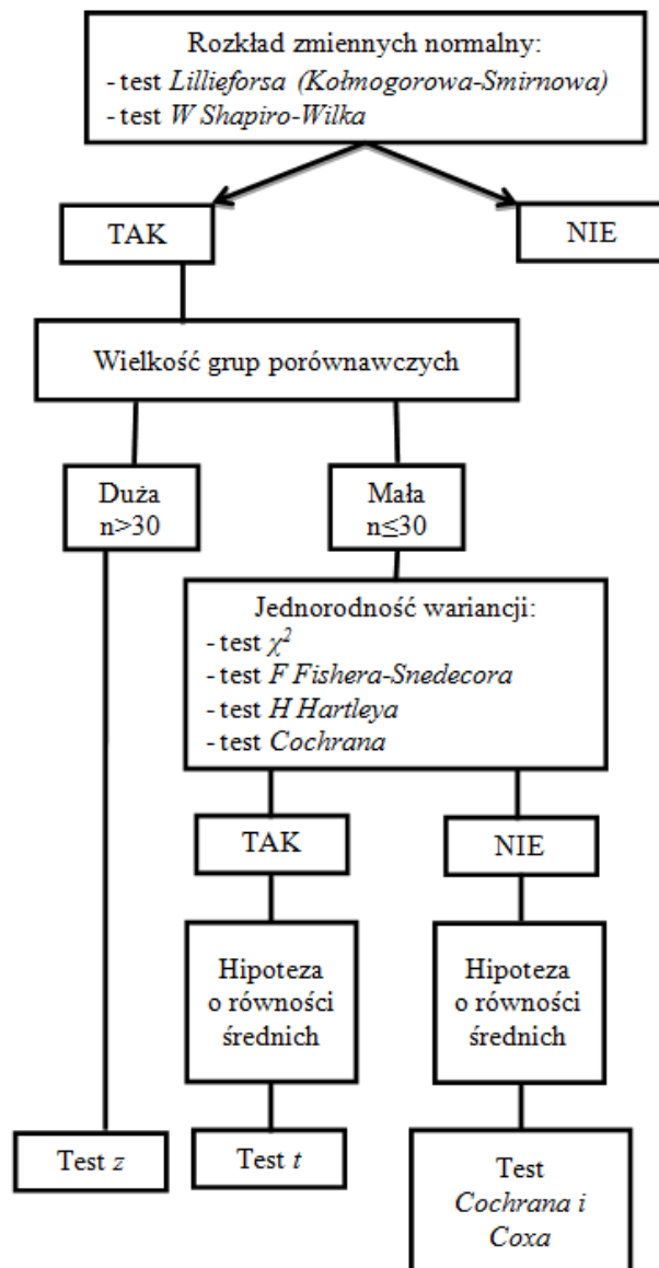
Rys. 6.1. Sposób postępowania podczas wyboru testu
