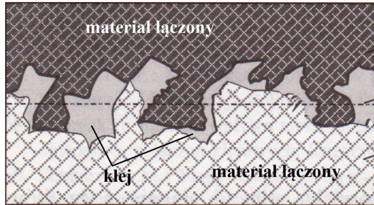
Rys. 1.4. Schemat połączenia adhezyjnego materiałów o chropowatej powierzchni, łączonych za pomocą kleju, przedstawiający mechaniczną teorię adhezji [111]
