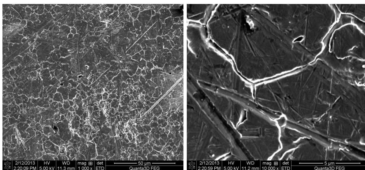
Rys. 5.12. Topografia powierzchni stali 316L po ozonowaniu
