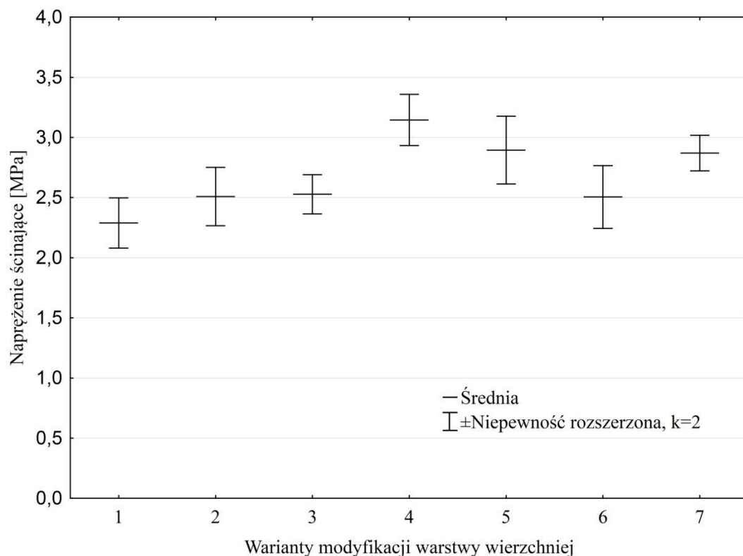
Rys. 5.44. Naprężenie ścinające uzyskane w badaniach eksperymentalnych dla próbek wykonanych z poliamidu 6 z użyciem kleju Hysol 9466 dla różnych warunków ozonowania (patrz str. 100)
