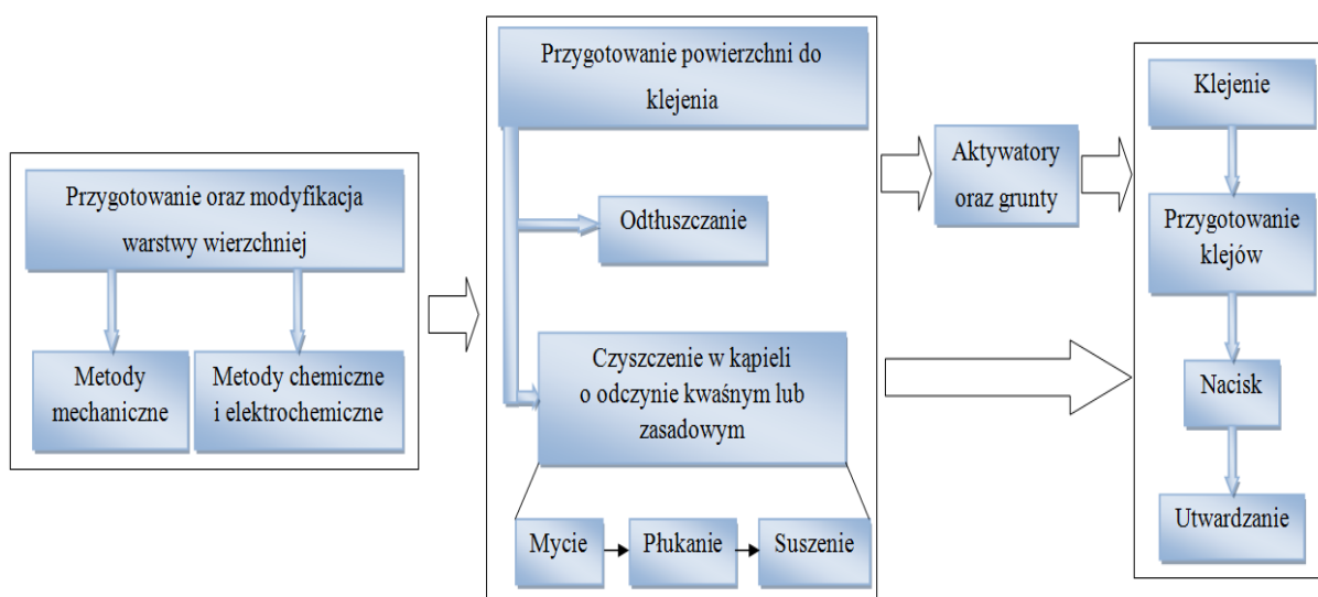
Rys. 1.5. Schemat operacji klejarskich
