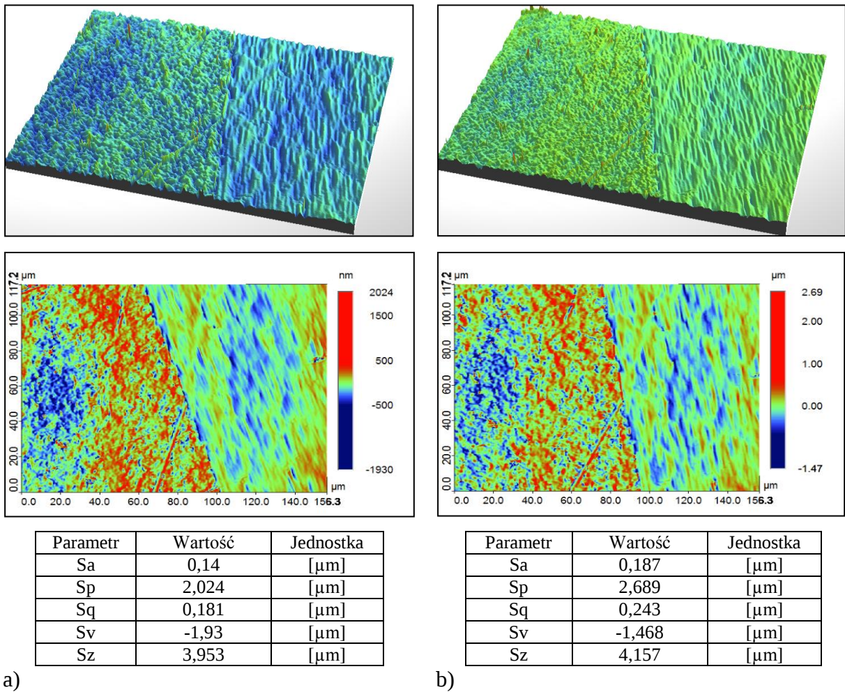
Rys. 5.7. Fotografie powierzchni próbki wykonanej ze stopu tytanu Ti-6Al-4V z wyraźną granicą po jonowym polerowaniu: a) przed ozonowaniem, b) po ozonowaniu
