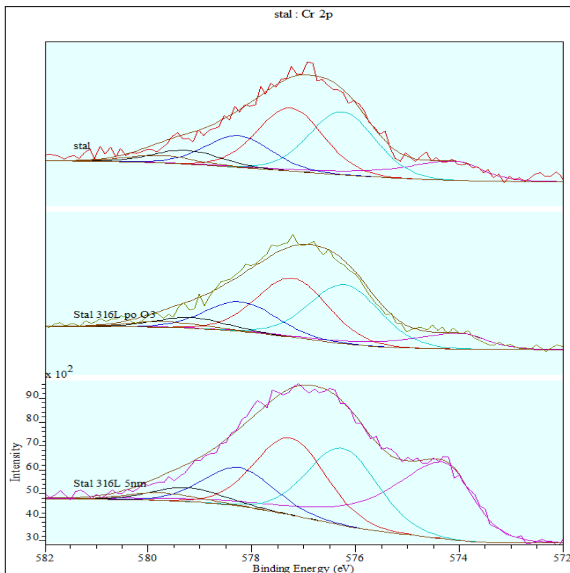
Rys. 5.27. Zestaw porównawczy widm XPS dla rejonu dubletu przejść Cr2p próbki stali 316L w kolejności, od góry: stal 316L przed ozonowaniem (stal), stal 316L po ozonowaniu (stal 316L po O3) oraz po czyszczeniu plazmowym (stal 316L 5nm)
