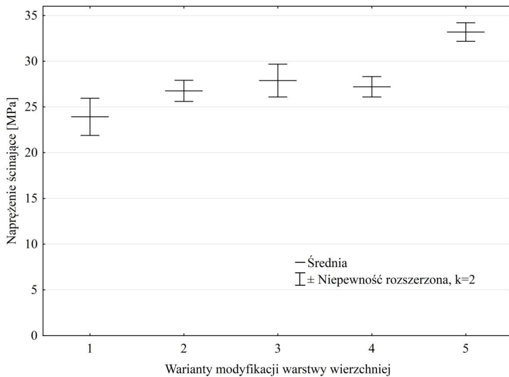
Rys. 5.45. Naprężenie ścinające uzyskane w badaniach eksperymentalnych dla próbek wykonanych ze stali 316L z użyciem kleju Hysol 9466 dla różnych warunków ozonowania (patrz str. 102)
