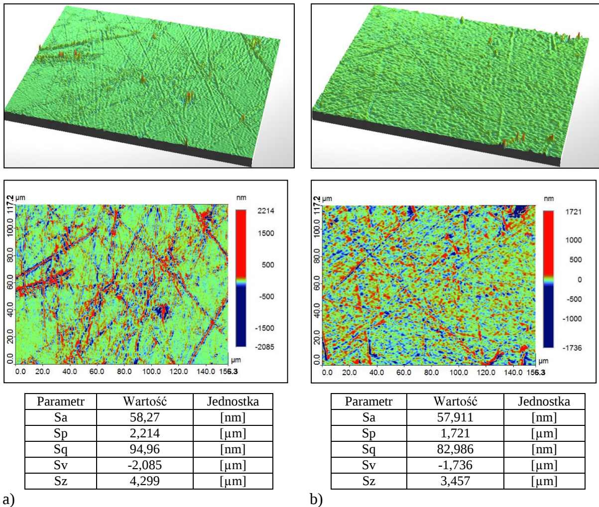
Rys. 5.4. Fotografie powierzchni oraz wartości wybranych parametrów chropowatości poliamidu 6 przed obróbką mechaniczną: a) przed ozonowaniem, b) po ozonowaniu
