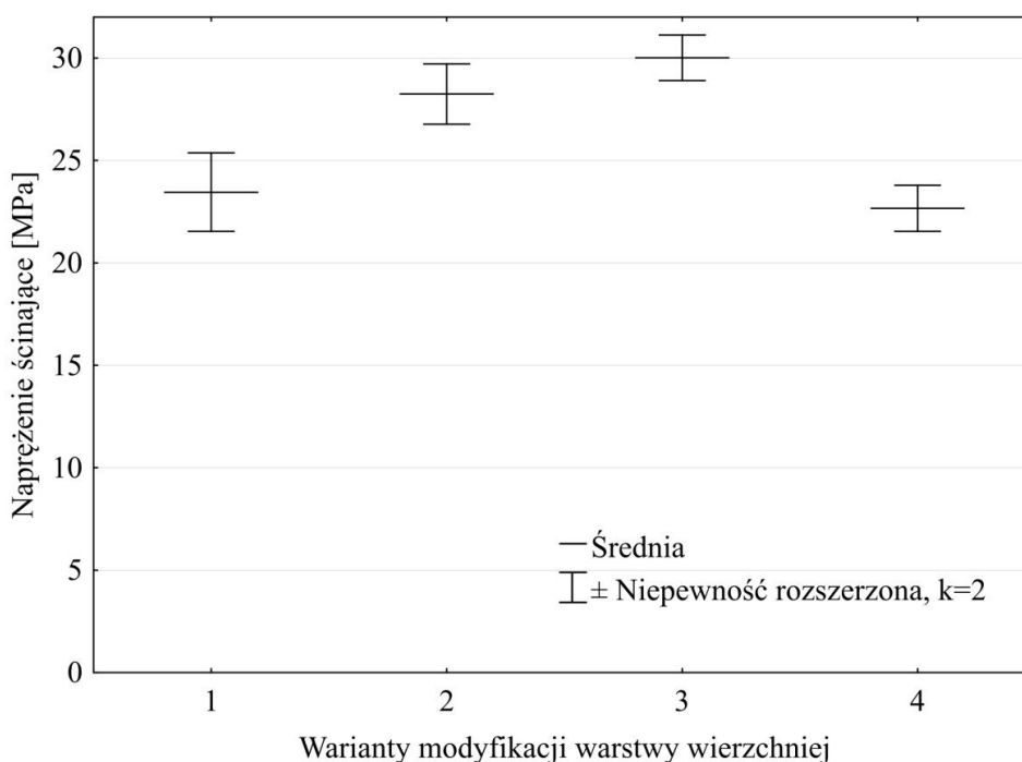
Rys. 5.46. Naprężenie ścinające w momencie zniszczenia, uzyskane w badaniach eksperymentalnych dla próbek wykonanych ze stopu tytanu Ti-6Al-4V z użyciem kleju Hysol 9466 dla różnych warunków ozonowania (patrz str. 105)
