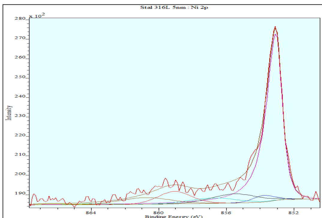
Rys. 5.24. Dekonwolucja widma XPS w rejonie Ni2p
