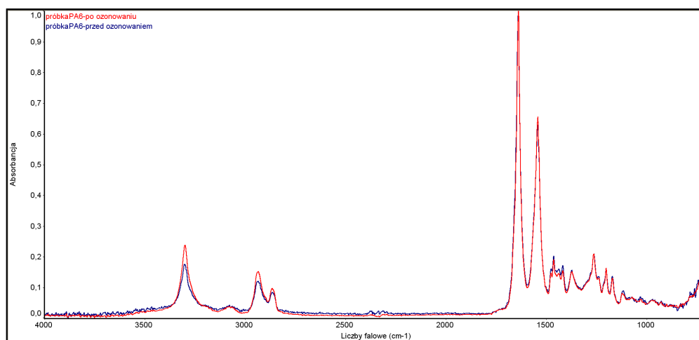
Rys. 5.10. Porównanie widm GATR polimeru, przed (kolor niebieski) i po ozonowaniu (kolor czerwony) - oś intensywności (absorbancja) znormalizowana
