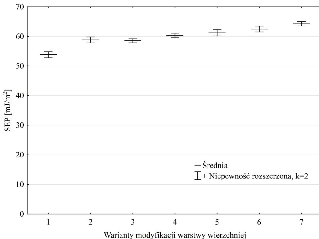
Rys. 5.36. Swobodna energia powierzchniowa poliamidu 6 po obróbce mechanicznej dla warunków ozonowania przedstawionych na str. 100
