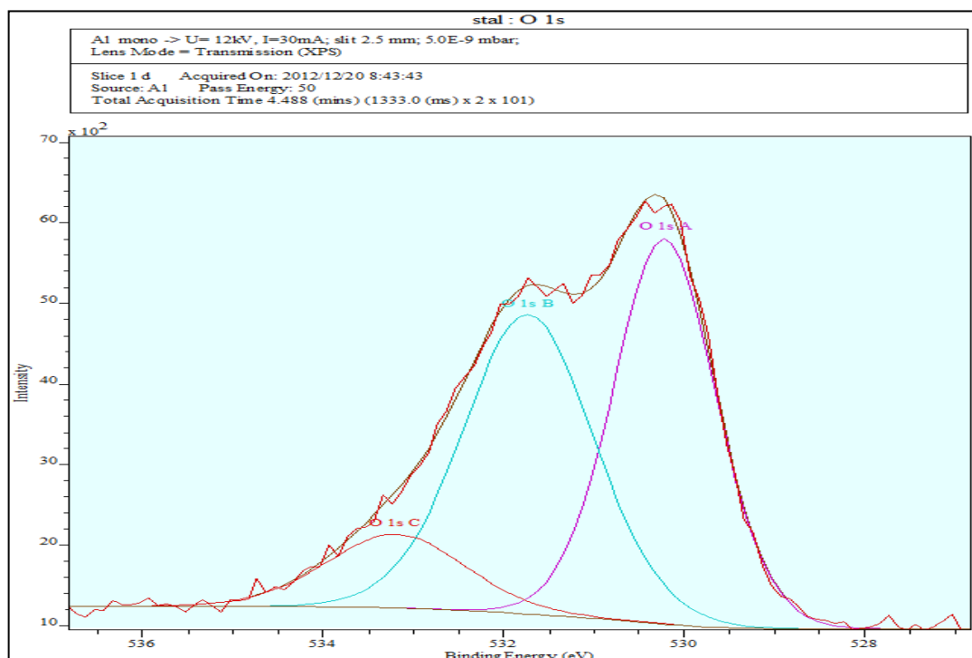
Rys. 5.25. Dekonwolucja widma XPS w rejonie tlenu
