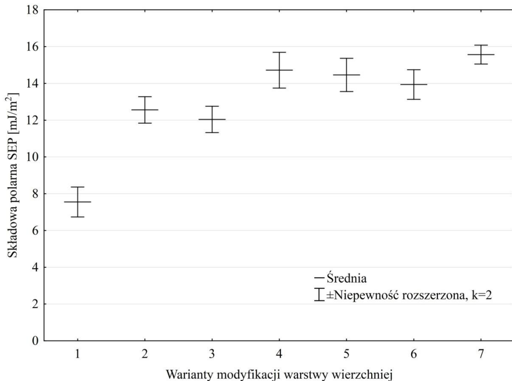
Rys. 5.37. Składowa polarna SEP poliamidu 6 po obróbce mechanicznej dla różnych warunków ozonowania (patrz str. 100)
