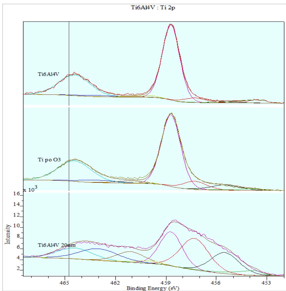
Rys. 5.30. Zmiany w paśmie dubletów przejść Ti2p
