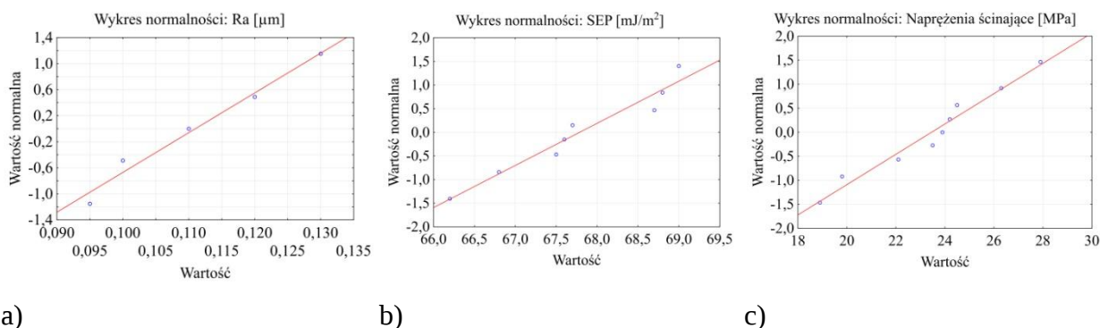
Rys. 6. 4. Wykresy normalności rozkładu wyników badań stopu tytanu Ti-6Al-4V: a) parametr chropowatości Ra, b) SEP, c) napężenia niszczące połączenie klejowe
