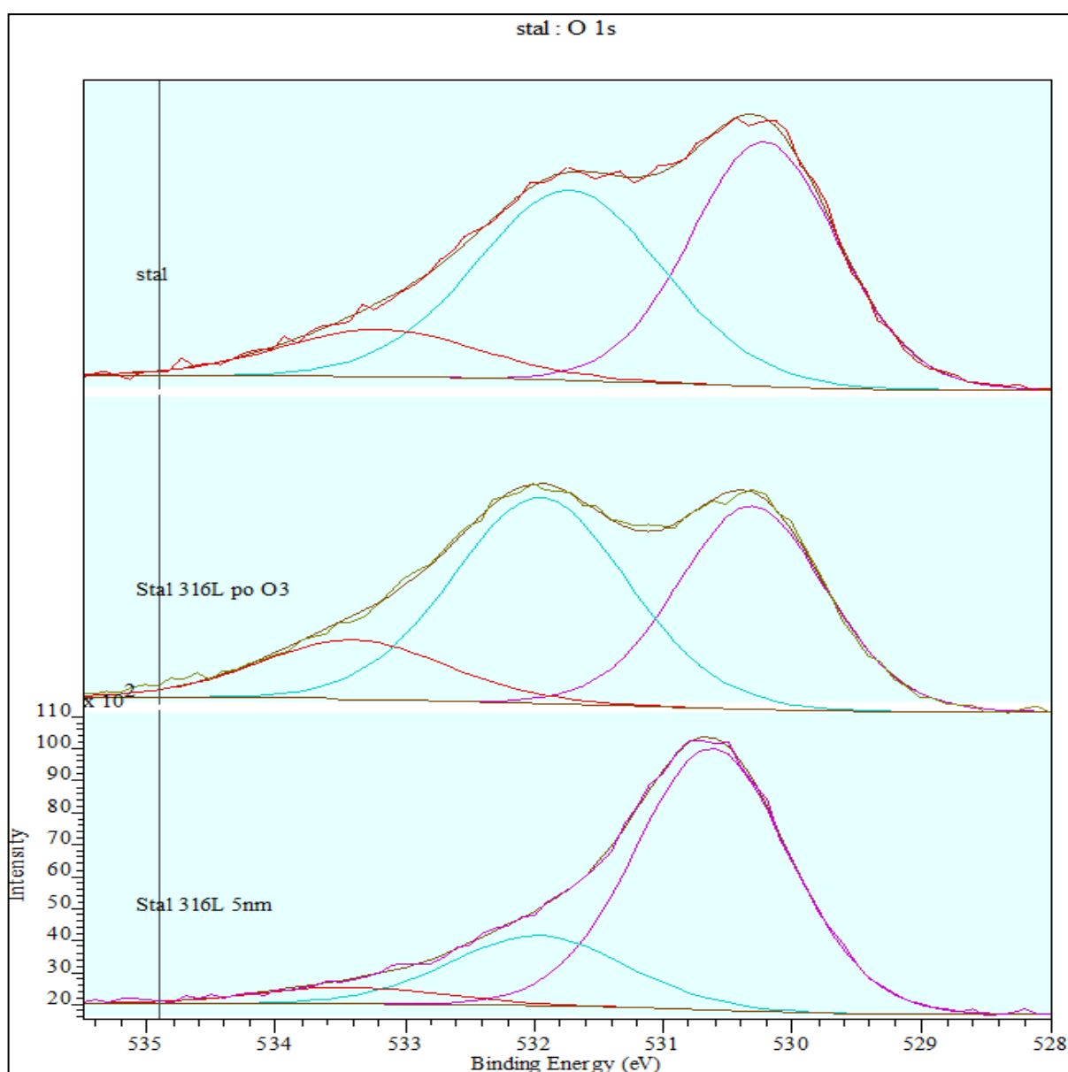
Rys. 5.28. Dekonwolucja widma XPS pasma O1s
