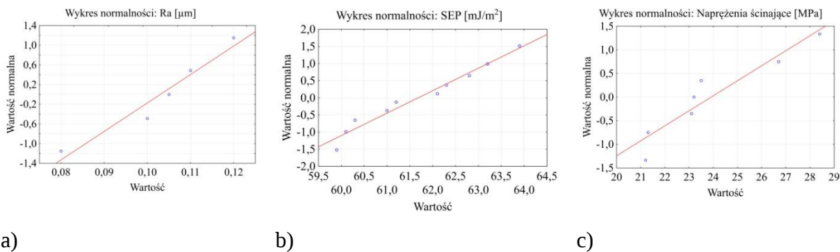
Rys. 6. 3. Wykresy normalności rozkładu wyników badań stali 316L: a) parametr chropowatości Ra, b) SEP, c) napężenia niszczące połączenie klejowe
