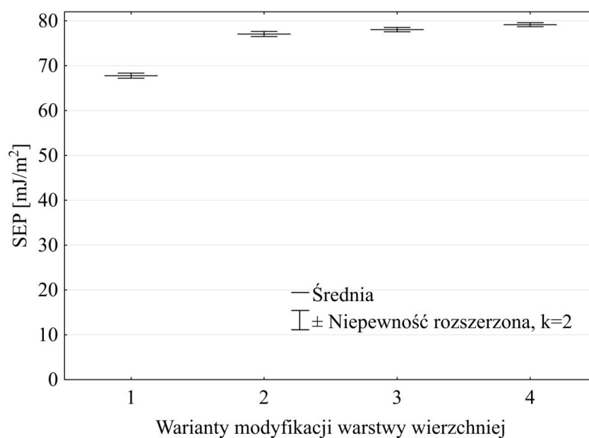
Rys. 5.42. Swobodna energia powierzchniowa stopu tytanu Ti-6Al-4V dla warunków ozonowania przedstawionych na str. 105
