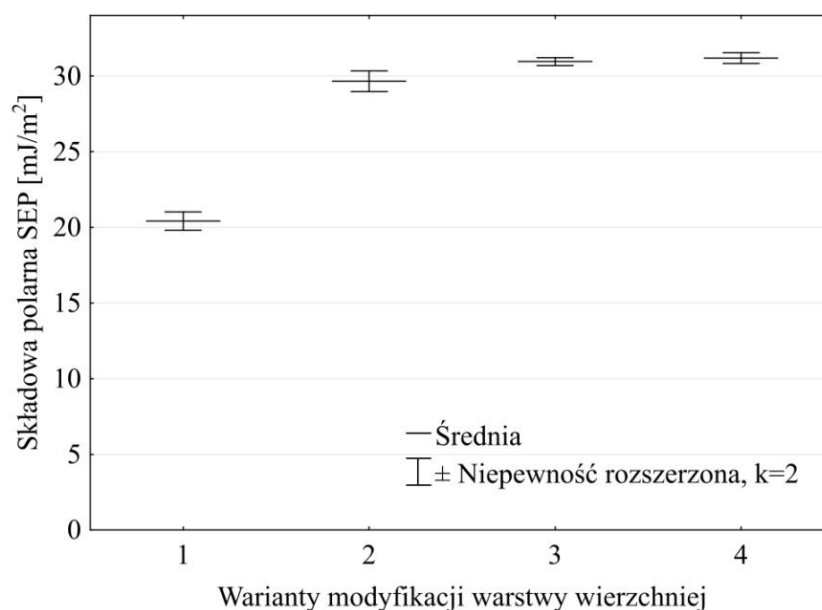
Rys. 5.43. Składowa polarna SEP stopu tytanu Ti-6Al-4V dla różnych warunków ozonowania (patrz str. 105)
