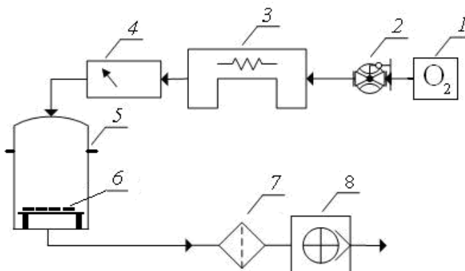
Rys. 3.5. Schemat stanowiska do ozonowania próbek materiałów konstrukcyjnych:
