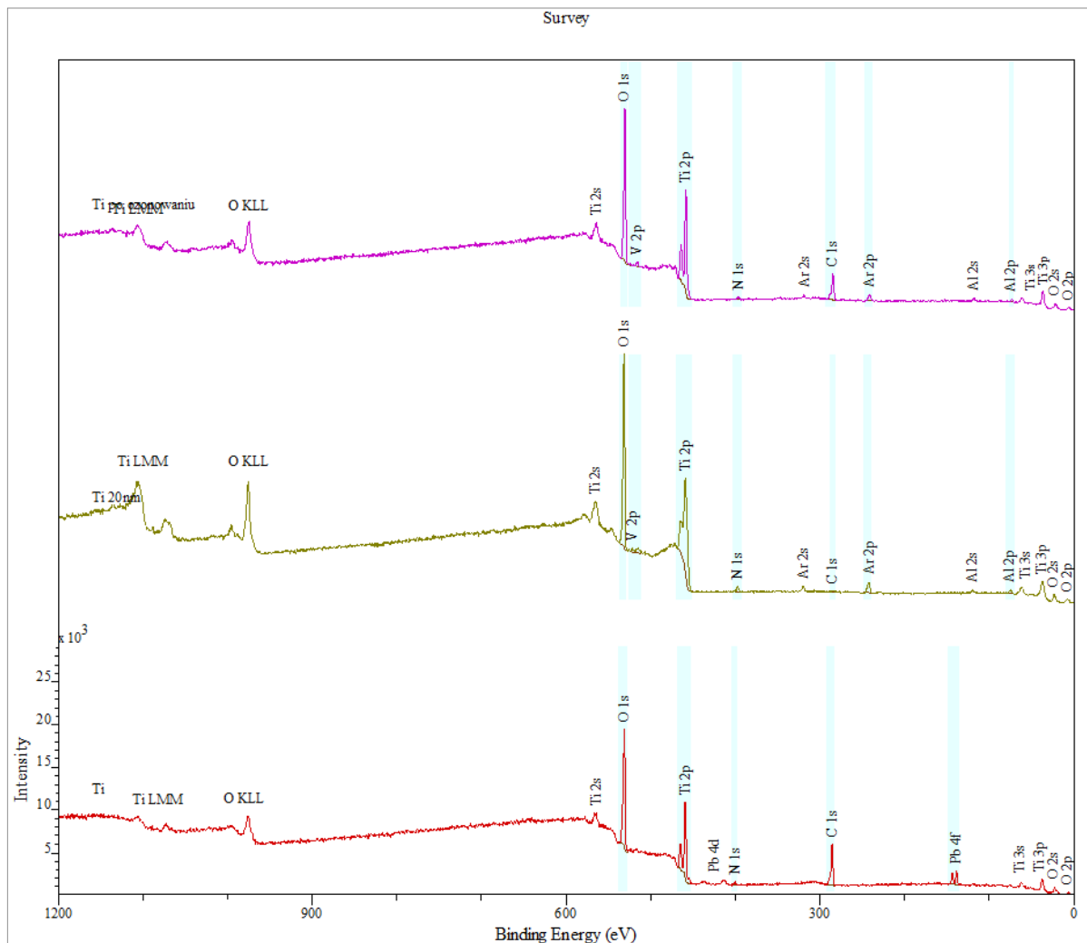
Rys. 5.29. Zestaw porównawczy szerokopasmowych widm XPS próbki stopu tytanu Ti-6Al-4V przedstawionych w kolejności: widmo stopu tytanu przed ozonowaniem (Ti), po czyszczeniu plazmowym (Ti 20nm) i po ozonowaniu (Ti po ozonowaniu)
