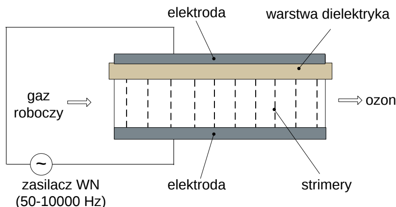
Rys. 1.7. Schemat generatora ozonu z wyładowaniami barierowymi [84]
