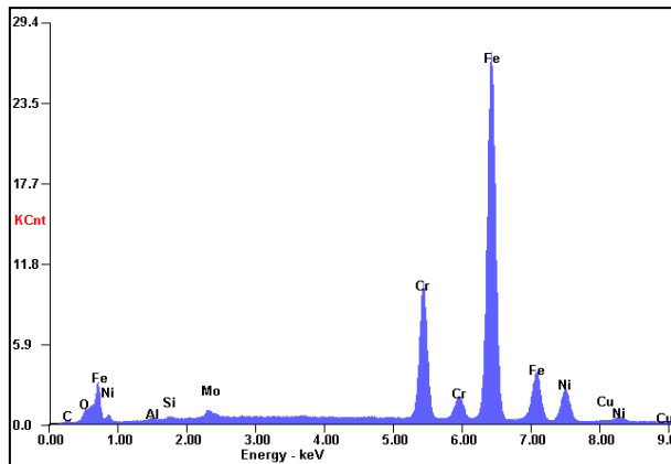
Rys. 5.13. Widmo EDX próbki stali 316L przed ozonowaniem oraz wynik analizy elementarnej obszaru
