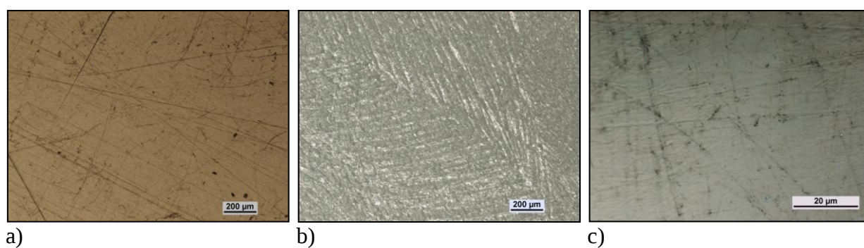
Rys. 5.1. Poliamid 6: a) powierzchnia poliamidu przed obróbką mechaniczną - powiększenie 50x, b) po obróbce mechanicznej - powiększenie 50x, c) obraz DIC powierzchni przed obróbką mechaniczną - powiększenie 1000x
