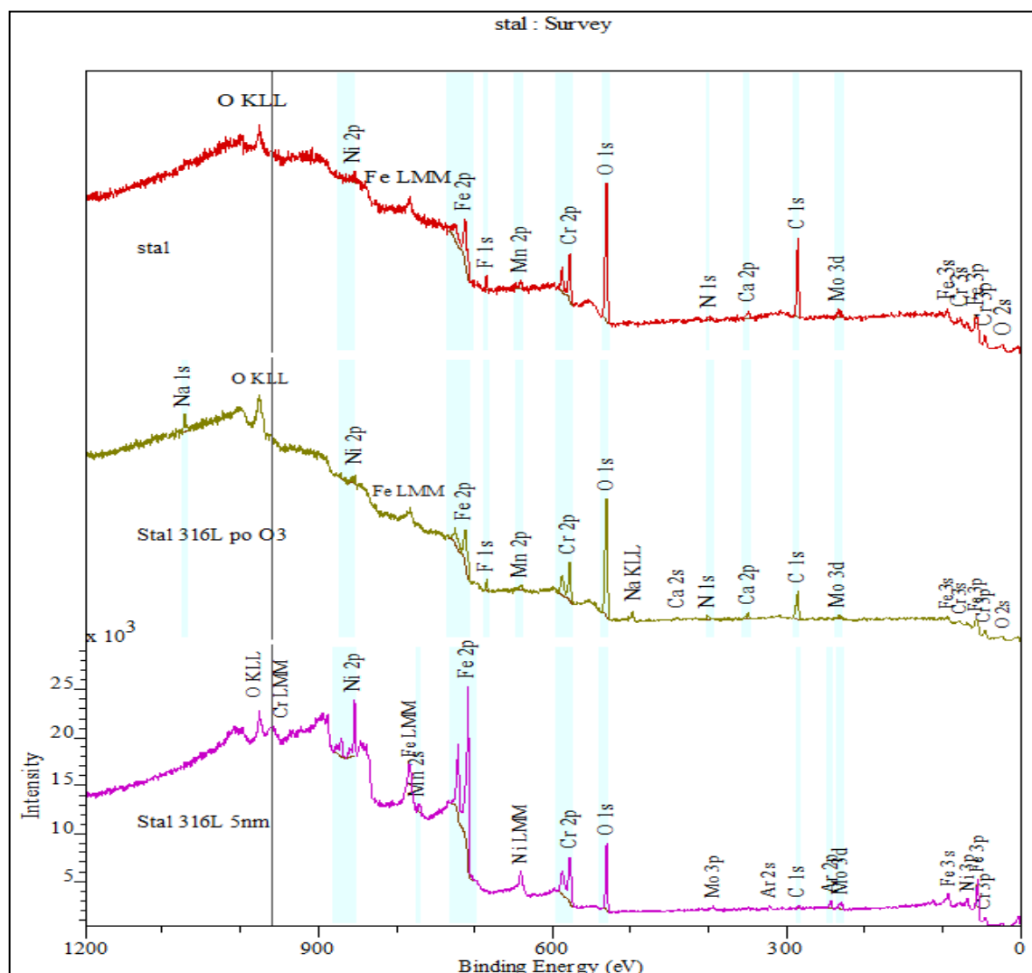
Rys. 5.21. Zestaw przeglądowych, szerokopasmowych widm XPS próbki stali 316L przedstawionych w kolejności: stal przed ozonowaniem (stal), po ozonowaniu (stal 316L po O3) oraz czyszczeniu plazmowym (stal 316L 5nm)
