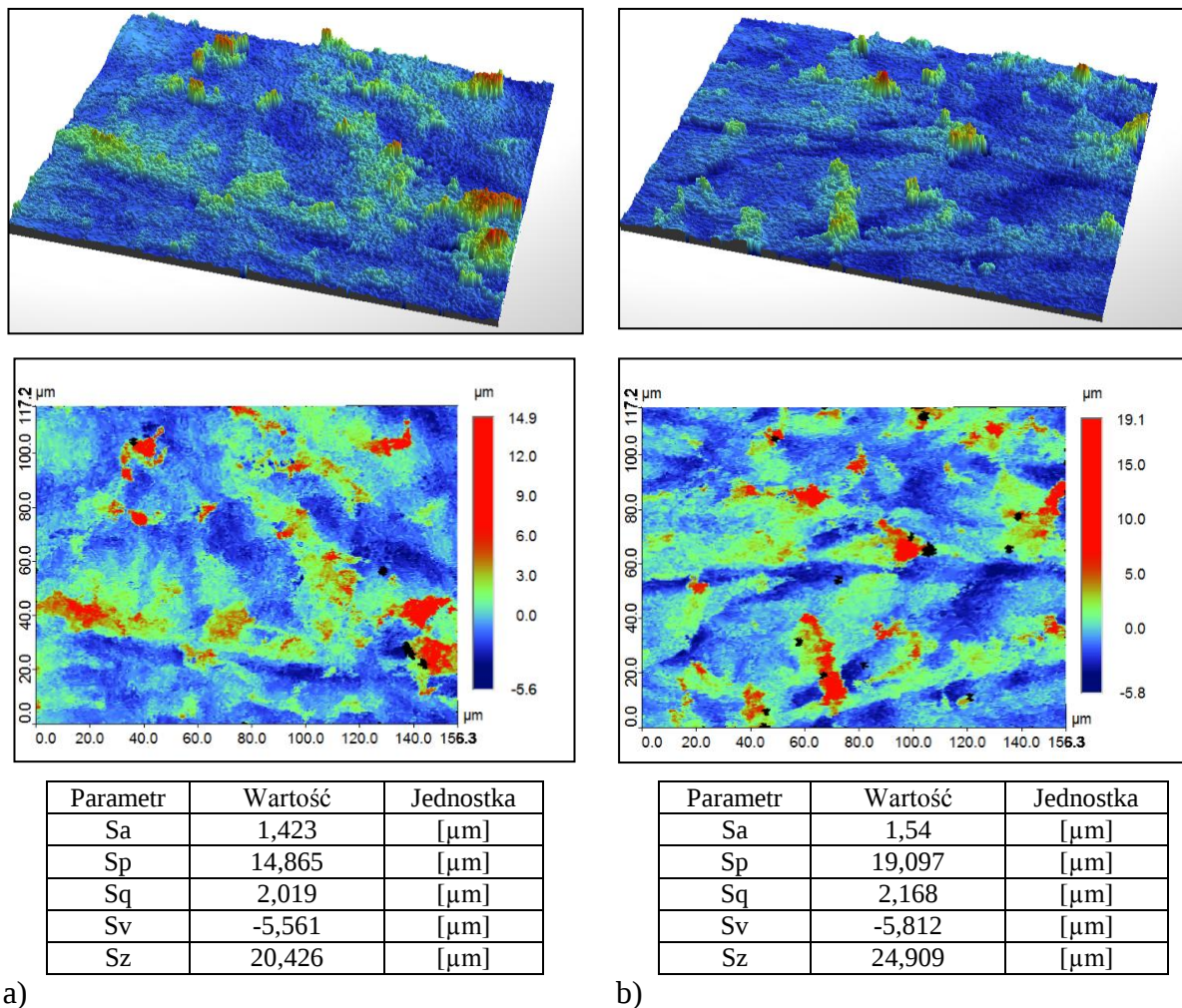
Rys. 5.5. Fotografie powierzchni oraz wartości wybranych parametrów chropowatości poliamidu 6 po obróbce mechanicznej: a) przed ozonowaniem, b) po ozonowaniu
