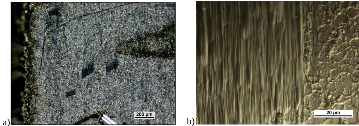
Rys. 5.2. Powierzchnia stali 316L: a) w świetle spolaryzowanym przy powiększeniu 50x, b) obraz DIC przy powiększeniu 1000x
