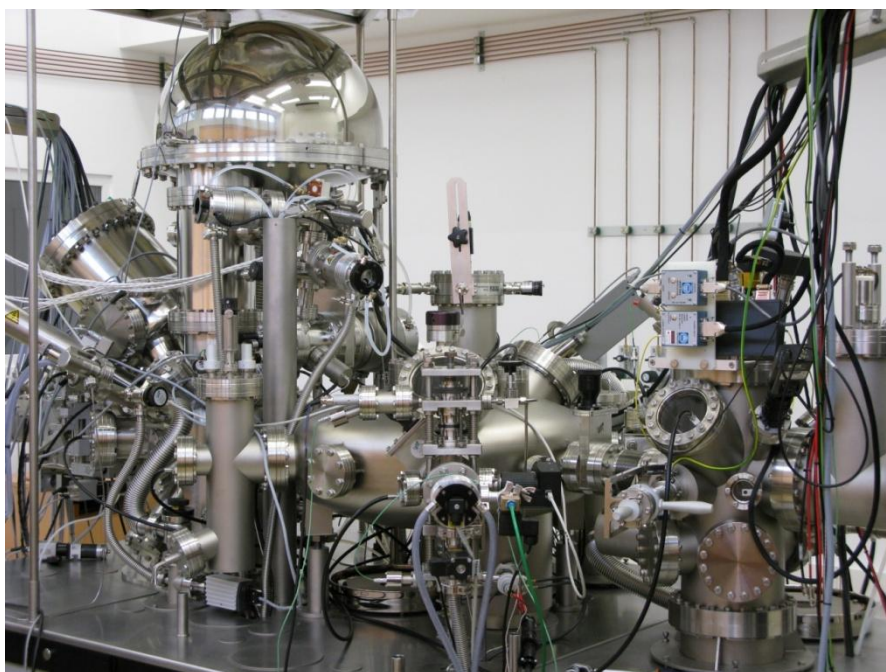
Rys. 3.10. Wielokomorowy system analityczny UHV
