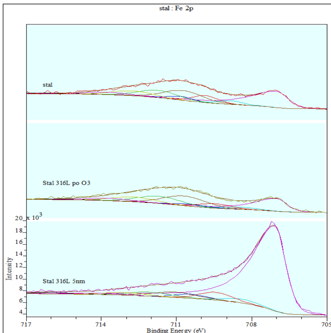
Rys. 5.26. Zestaw wysokorozdzielczych widm XPS dla rejonu dubletu przejść Fe2p próbki stali 316L przedstawionych w kolejności: stal przed ozonowaniem (stal), po ozonowaniu (stal 316L po O3) i po czyszczeniu jonowym (stal 316L 5nm)
