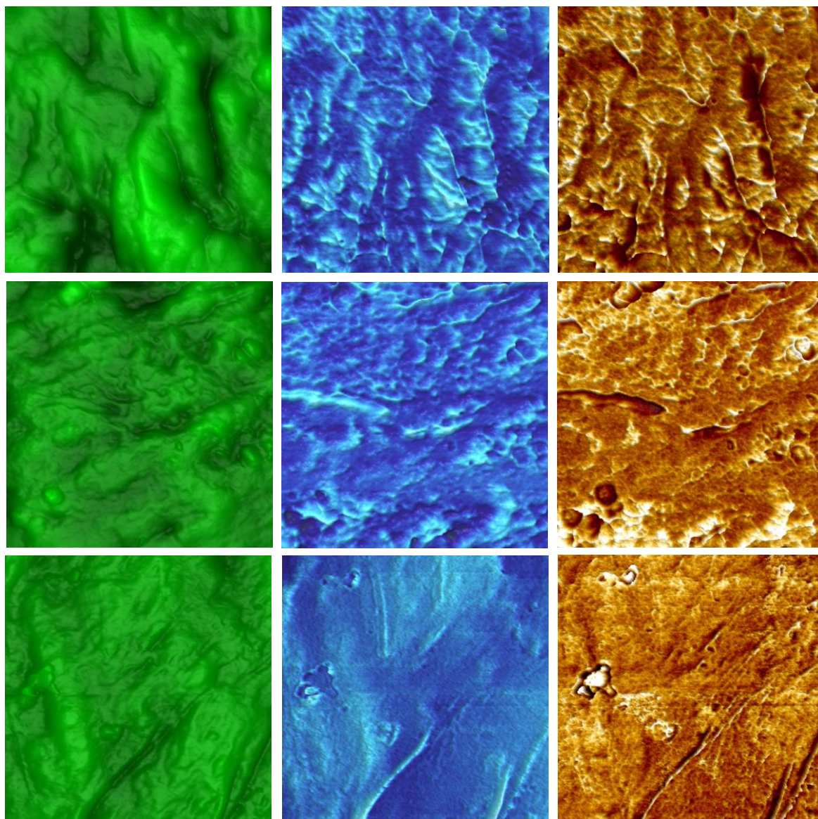
Rys. 5.8. Mapy topografii powierzchni (kolor zielony), adhezji (kolor niebieski) oraz modułu Young'a (kolor brązowy) dla poliamidu 6 przed modyfikacją (górny szereg) i po modyfikacji z pośrednią (panel środkowy) i minimalną wartością adhezji (panel dolny)
