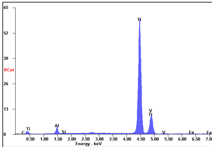
Rys. 5.19. Widmo EDX próbki stopu tytanu Ti-6Al-4V po ozonowaniu oraz wynik analizy elementarnej obszaru
