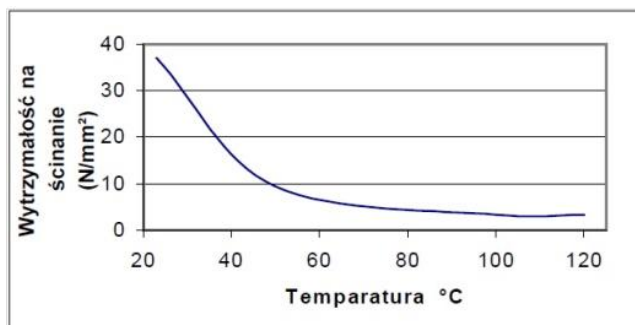
Rys. 3.2. Wytrzymałość na ścinanie w funkcji temperatury dla kleju Hysol 9466 [133]
