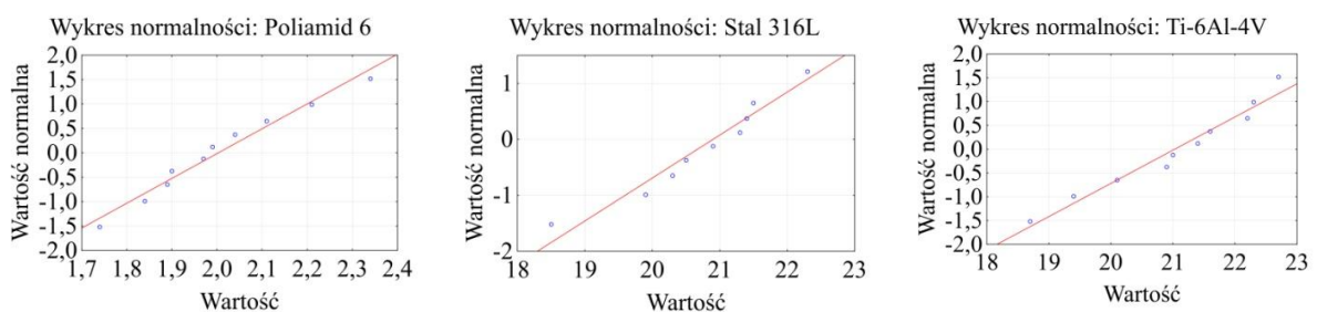
Rys. 4.1. Wykresy normalności rozkładu wyników naprężenia niszczącego
