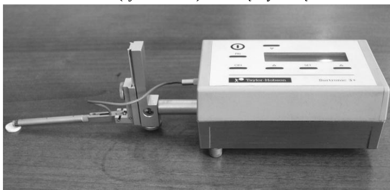
Rys. 3.8. Profilografometr firmy Taylor Hobson Surtronic3+
