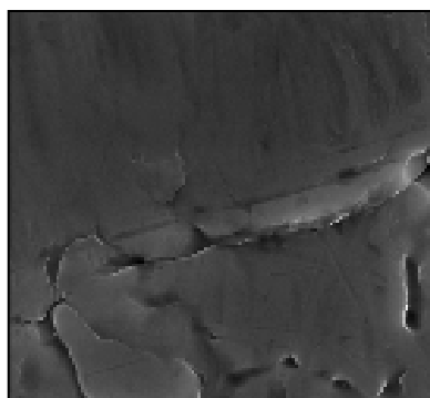
Rys. 5.15. Topografia próbki stali 316L, powiększenie 10000x
