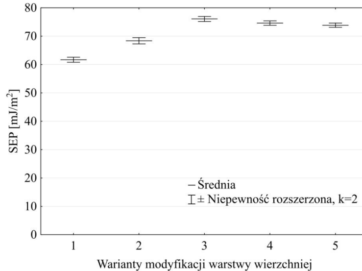
Rys. 5.38. Swobodna energia powierzchniowa stali 316L po obróbce mechanicznej dla warunków ozonowania przedstawionych na str. 102
