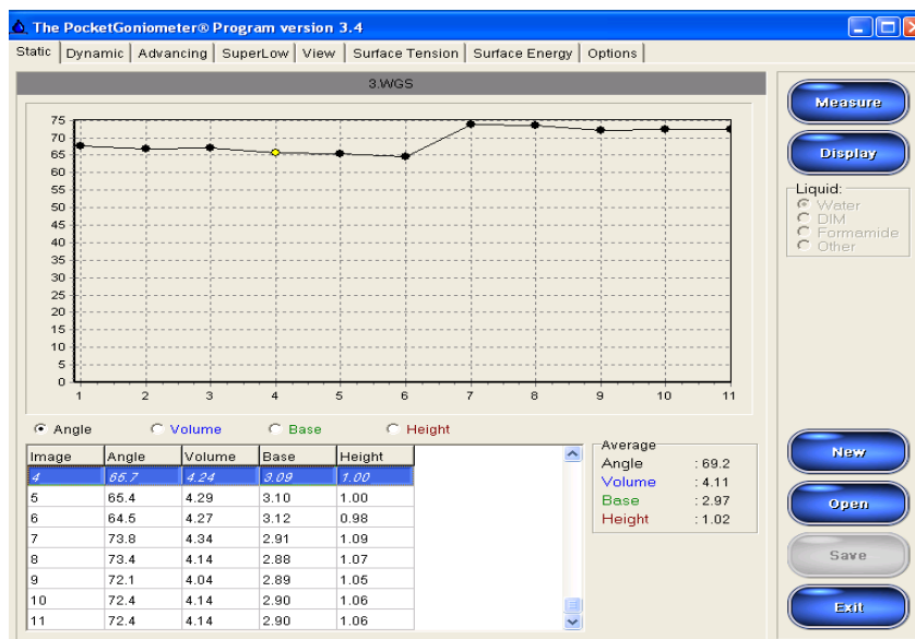
Rys. 3.7. Interfejs programowy goniometru PGX
