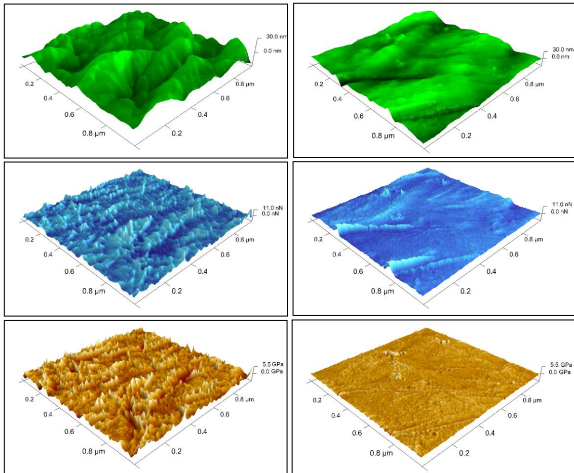
Rys. 5.9. Mapy 3D AFM, obszar skanowania: 1\mu\text{m} \times 1\mu\text{m} , skala wysokości znormalizowana, kolumna lewa - przed ozonowaniem, kolumna prawa - po ozonowaniu
