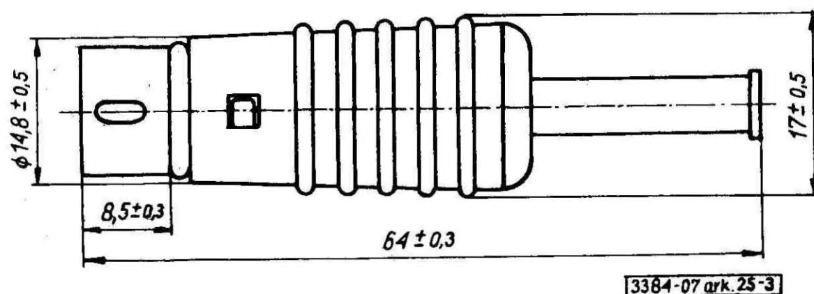
Rys. 3. Wspólne wymiary wtyczek WM 345-2 i WM 545-2
