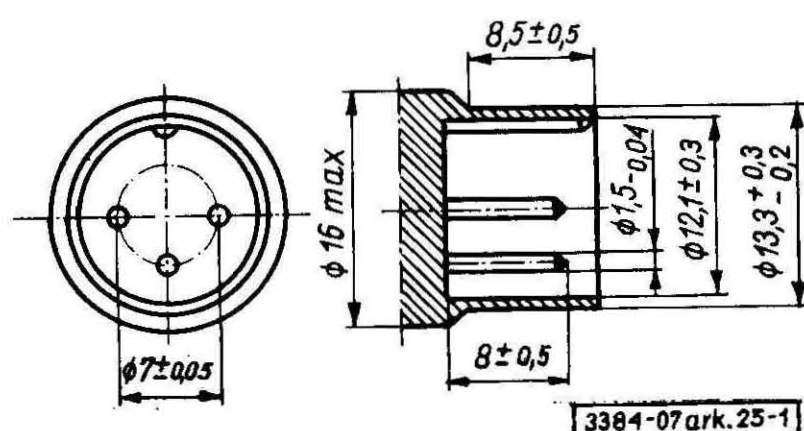
Rys. 1. Rozstawienie styków i wymiary części łączącej wtyczki WM 345-2
