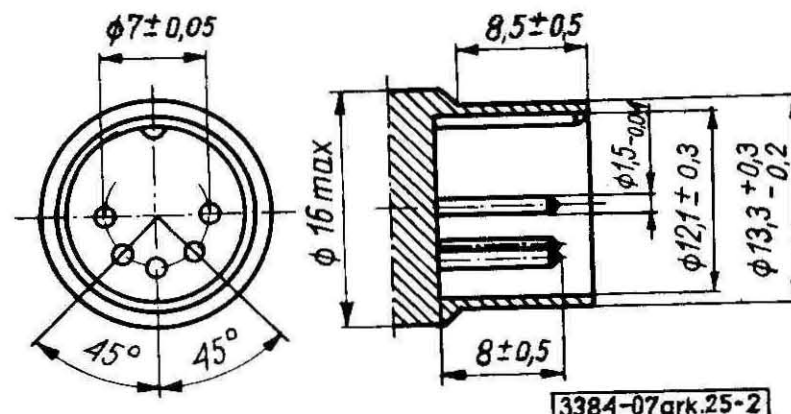
Rys. 2. Rozstawienie styków i wymiary części łączącej wtyczki WM 545-2
