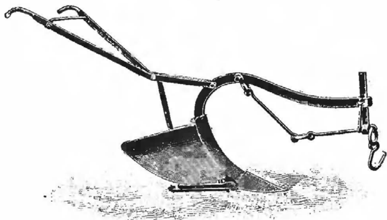
Radelko (obsypnik) całożelazne Gutowskiego.
