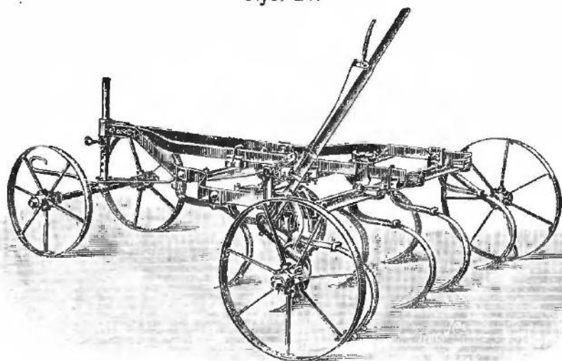
Kultywator sprężynowy o 7 zębach na kółkach.
