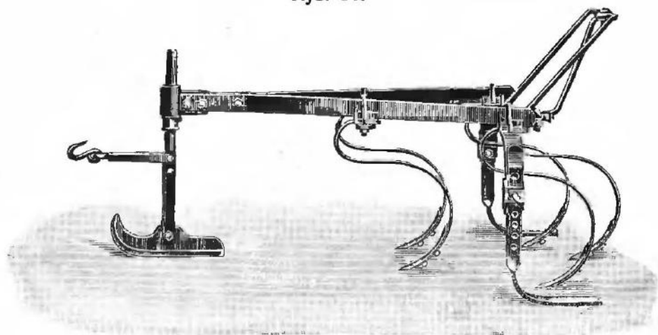
Kultywator sprężynowy pięciozębowy.
