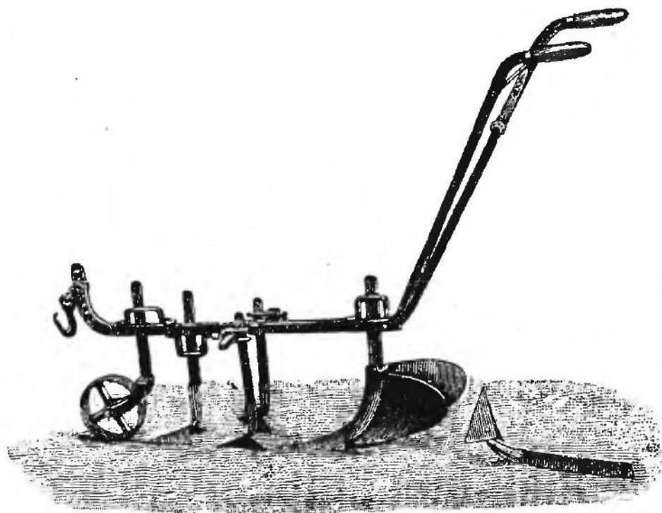
Rys. 39. Wypielacz-obsypnik angielski
