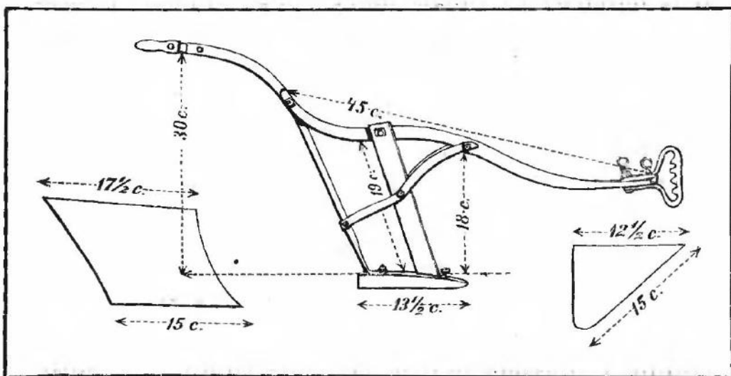
Rysunek (szablon) pługa na stolnicy, zbitej z desek. Na prawo pod regulatorem lemiesz, na lewo—odkładnica. Wymiary w calach.
