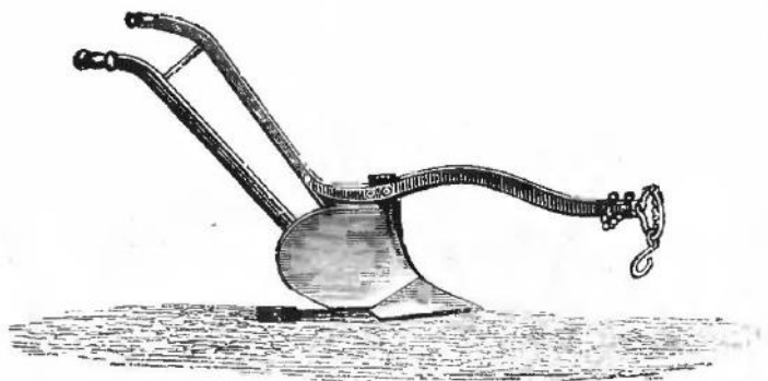
Rys. 18. Pług Cichowskiego № 1.
