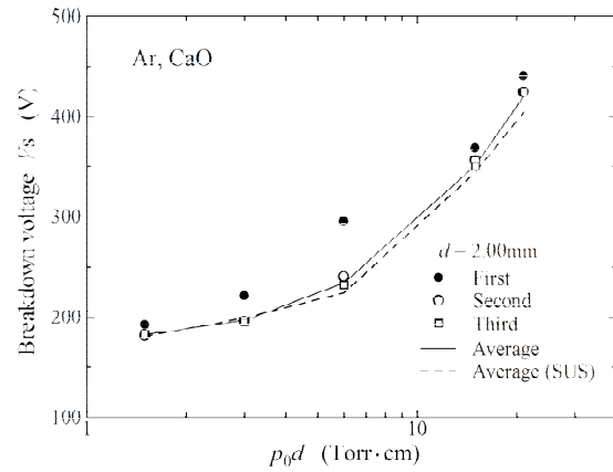
Fig. 10 Paschen curve.
