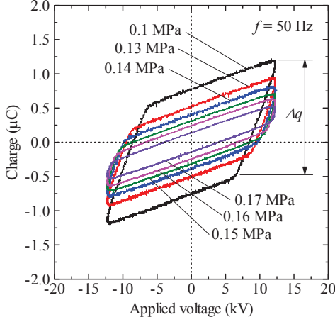
Fig. 5. Lissajous figures.
