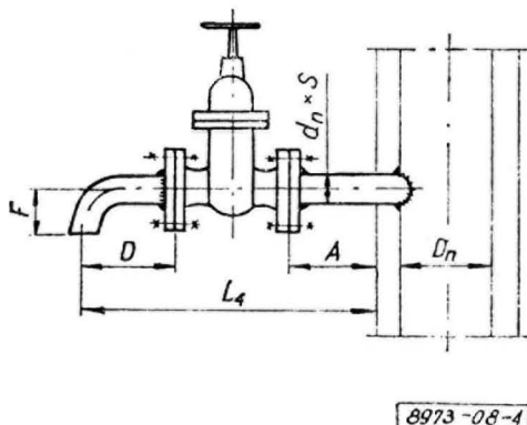
Rys. 4. Odwadniacz rurociągów pionowych rodzaju II odmiany B
