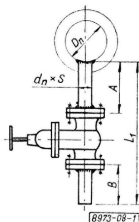
Rys. 1. Odwadniacz rurociągów poziomych rodzaju I odmiany A
