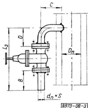
Rys. 3. Odwadniacz rurociągów pionowych rodzaju II odmiany A
