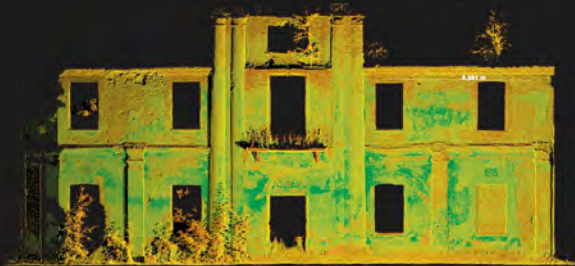
Ryc. 7.7. Elewacja północno-zachodnia - chmura punktów.
