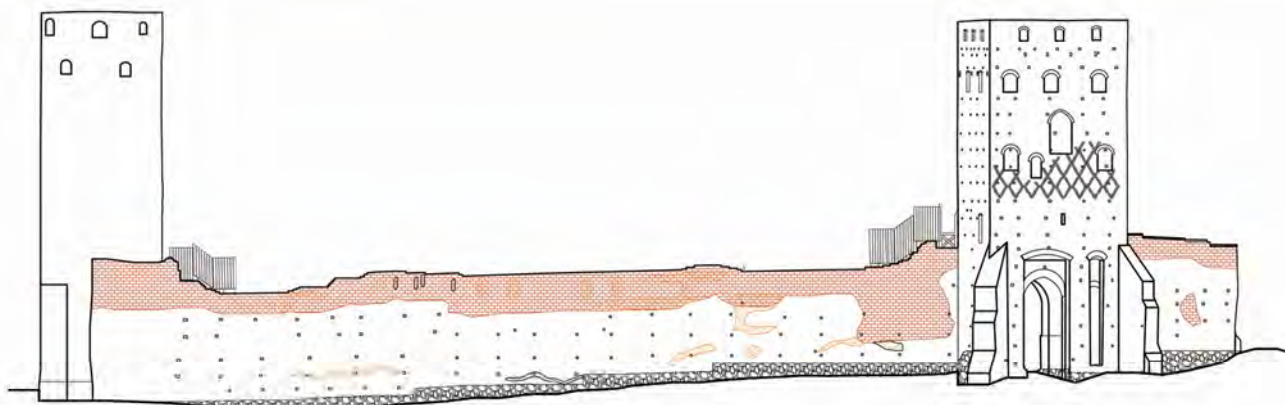
Ryc. 3.4. Elewacja wschodnia - widok od strony zewnętrznej. Widok elewacji wraz z oznaczeniem uszkodzeń.
