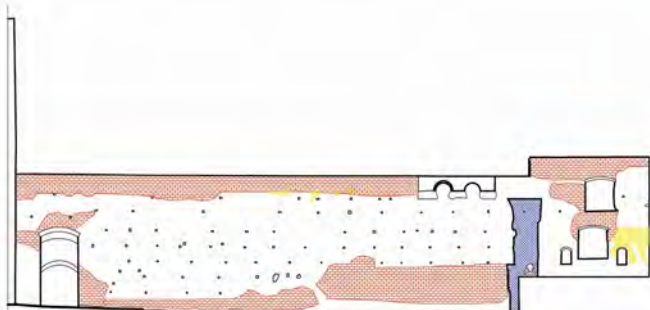
Ryc. 2.7. Elewacja zachodnia wewnętrzna.
