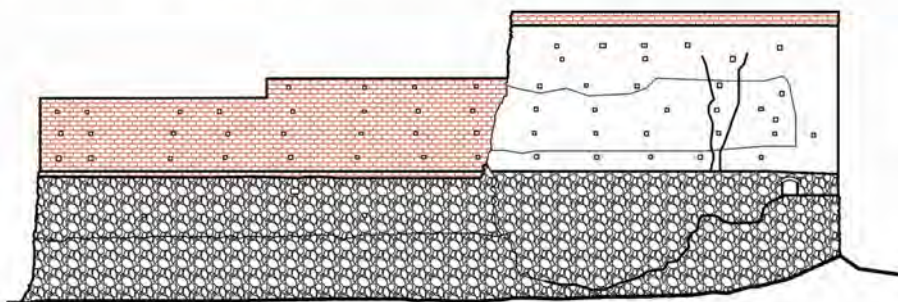
Ryc. 5.4. Elewacja północno-wschodnia zewnętrzna.
