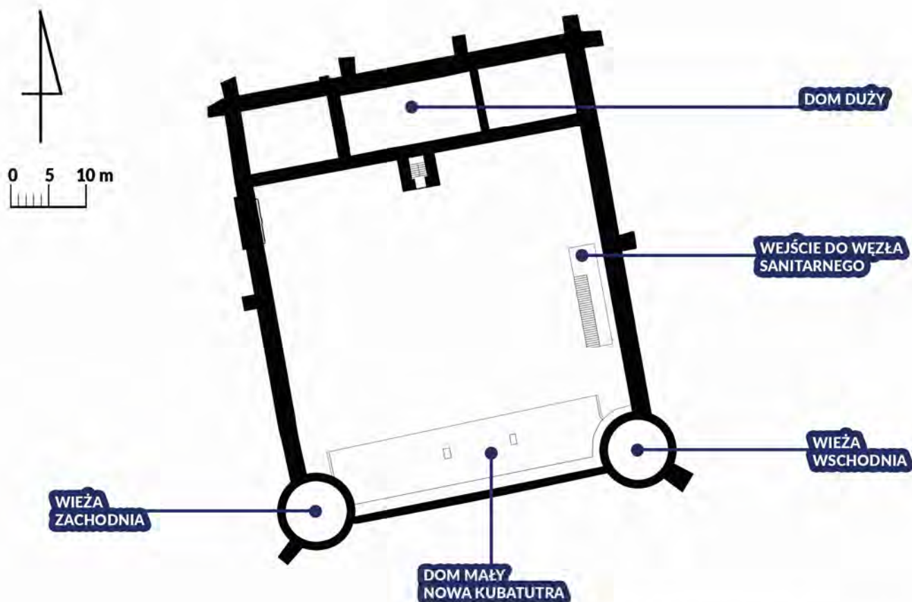
Ryc. 2.2. Plan Zamku Książąt Mazowieckich w Ciechanowie.
