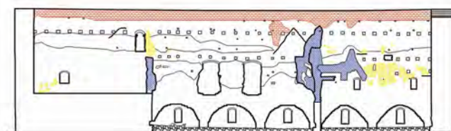
Ryc. 2.8. Elewacja północna wewnętrzna.
