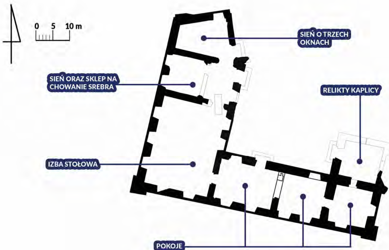
Ryc. 5.3. Plan Zamku Książąt Mazowieckich w Sochaczewie.
