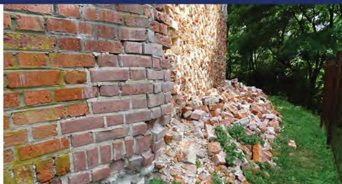
Fot. 3.12. Mur obwodowy północny.
