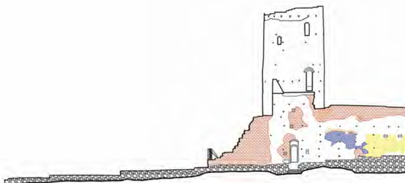
Ryc. 3.7. Elewacja zachodnia - widok od strony dziedzińca. Widok elewacji wraz z oznaczeniem uszkodzeń.
