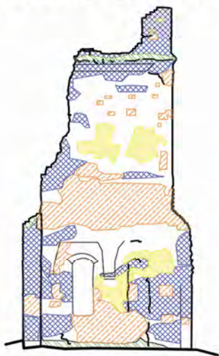
Ryc. 1.3. Elewacja południowa.
