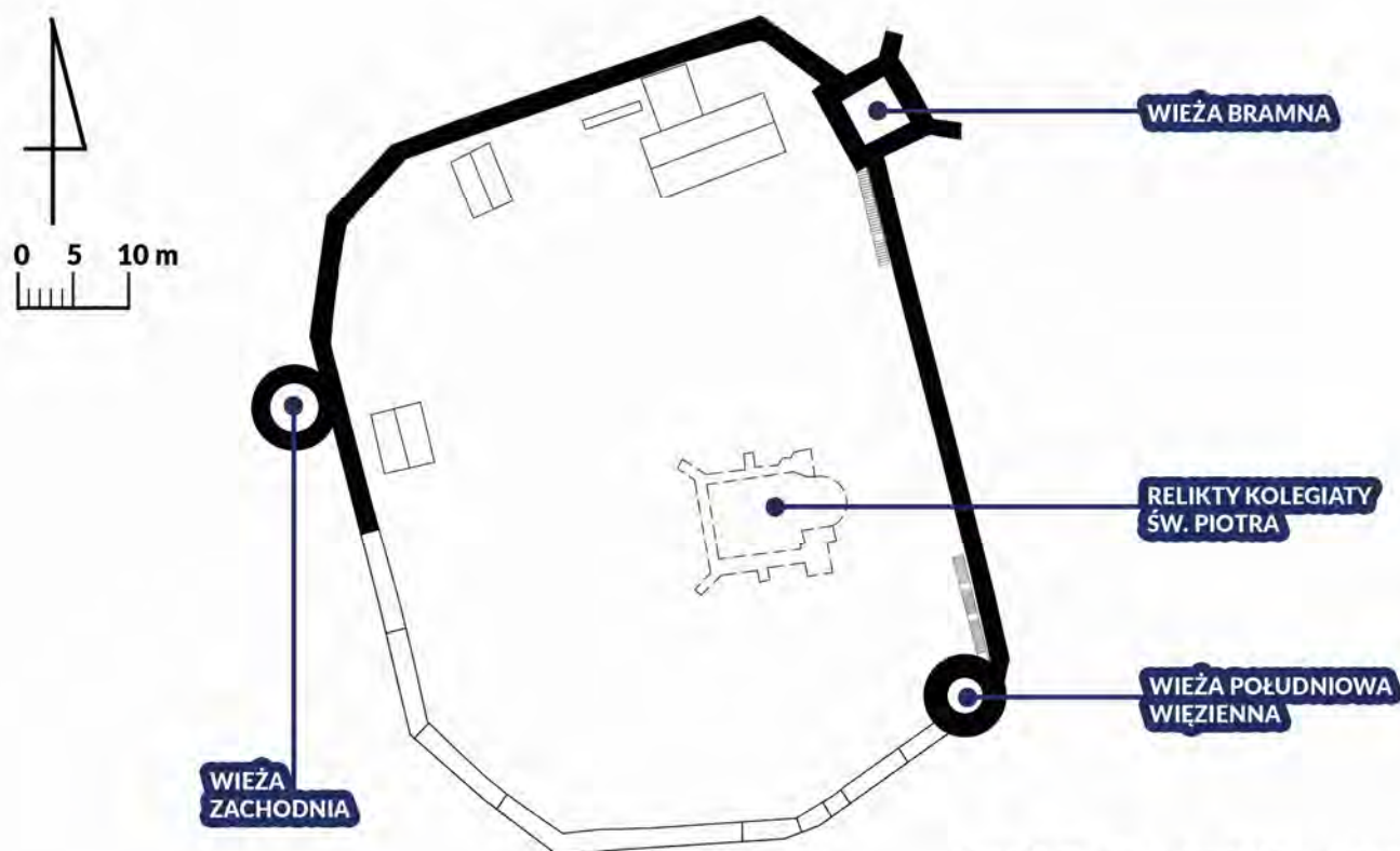
Ryc. 3.3. Plan Zamku Książąt Mazowieckich w Czersku.
