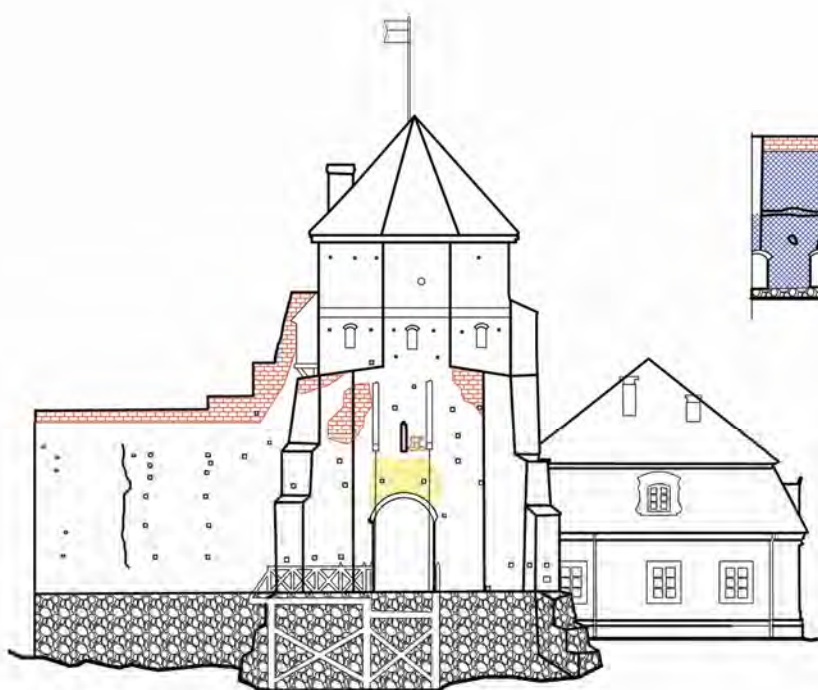
Ryc. 5.7. Elewacja północno-zachodnia zewnętrzna.
