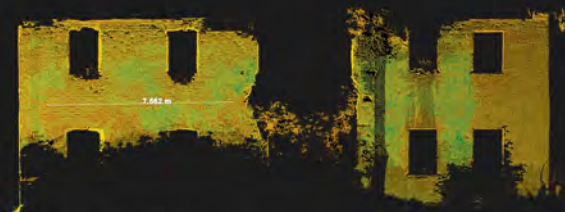
Ryc. 7.9. Elewacja południowo-wschodnia - chmura punktów.
