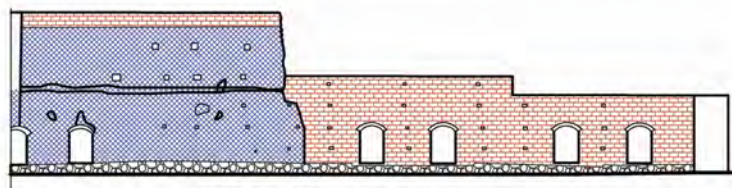
Ryc. 5.6. Elewacja południowo-wschodnia zewnętrzna.
