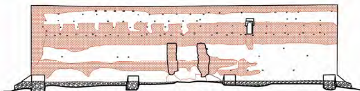
Ryc. 2.6. Elewacja północna zewnętrzna.
