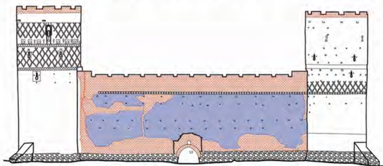
Ryc. 2.3. Elewacja południowa zewnętrzna.
