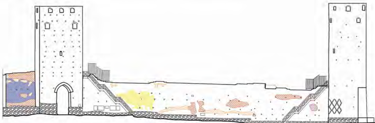
Ryc. 3.5. Elewacja wschodnia - widok od strony dziedzińca. Widok elewacji wraz z oznaczeniem uszkodzeń.
