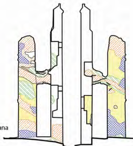
Ryc. 1.7. Wewnętrzna ściana południowa.
