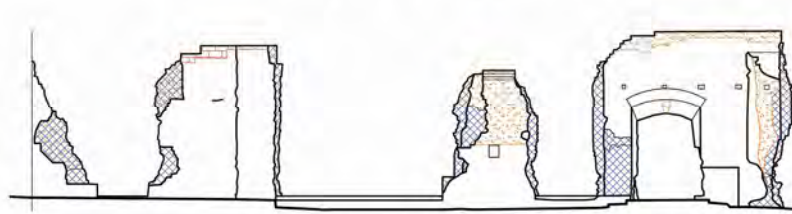
Ryc. 5.6. Elewacja południowo-wschodnia zewnętrzna.
