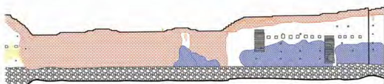
Ryc. 3.6. Elewacja północna - widok od strony dziedzińca. Widok elewacji wraz z oznaczeniem uszkodzeń.
