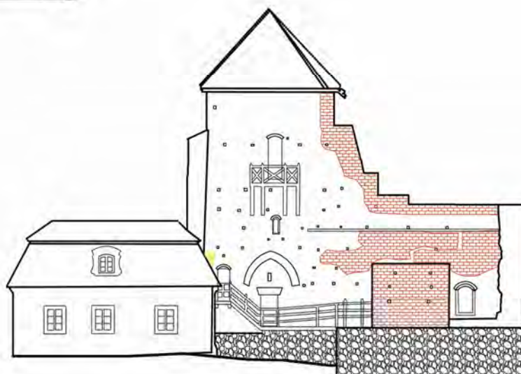
Ryc. 5.8. Elewacja północno-zachodnia wewnętrzna.
