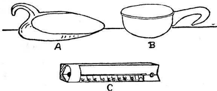
Ryc. 14. A kielnia, B czepak, C termometr w oprawie.
