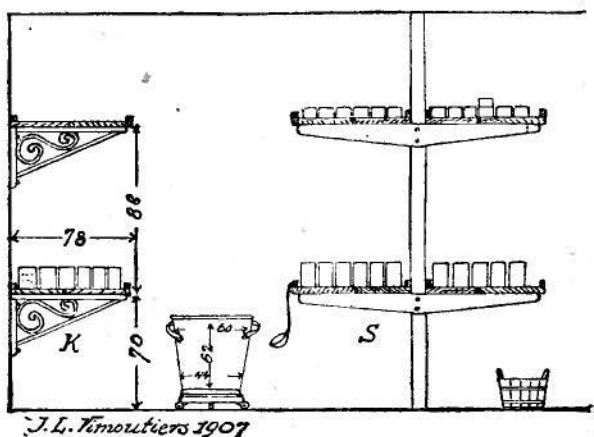
Ryc. 60. Stoły do formowania i ociekania serów camembert. K na konsoli, S na słupach ramiennych.
