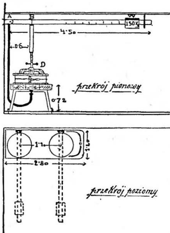
Ryc. 33. Prasa Schatzmanna.
