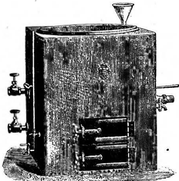
Ryc. 15. Kociołek Gaulina.
