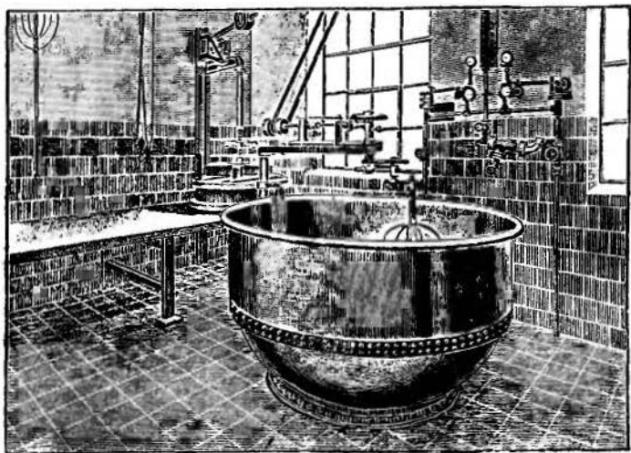
Ryc. 22. Kocioł do ogrzewania parą i wnętrze nowoczesnej warzelni (typ algauski).
