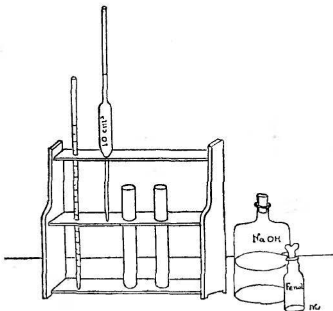
Ryc. 2. Najprostsze przybory do oznaczenia kwasowości.
