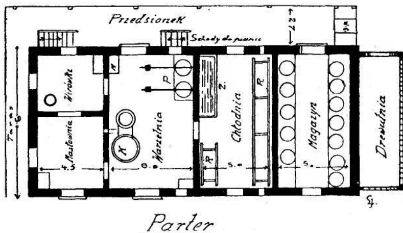
Ryc. 46. Rzut poziomy.
