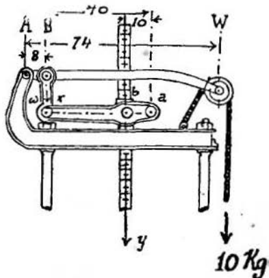
Ryc. 36. Działanie siły na złożonych dźwigniach (według Kirchnera).
