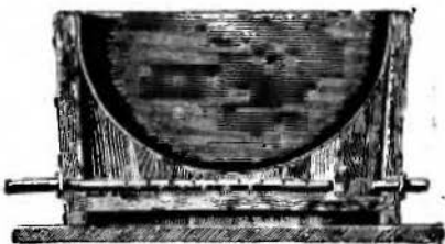
Ryc. 20. Kociołek ogrzewany parą, umieszczony w drewnianej kadzi.
