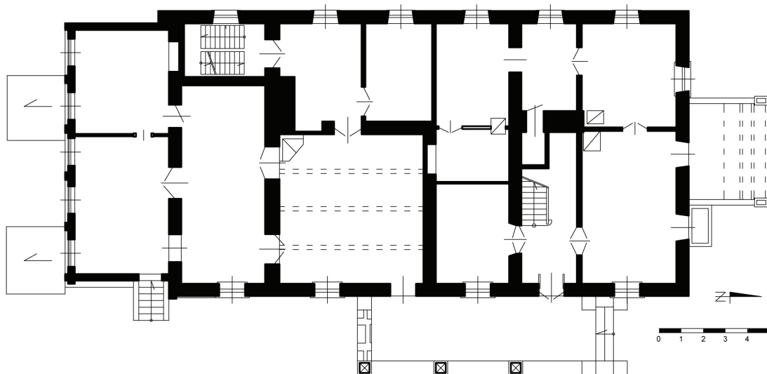
Il. 147. Schemat rzutu kondygnacji parteru, źródło: archiwum KAUiPP
