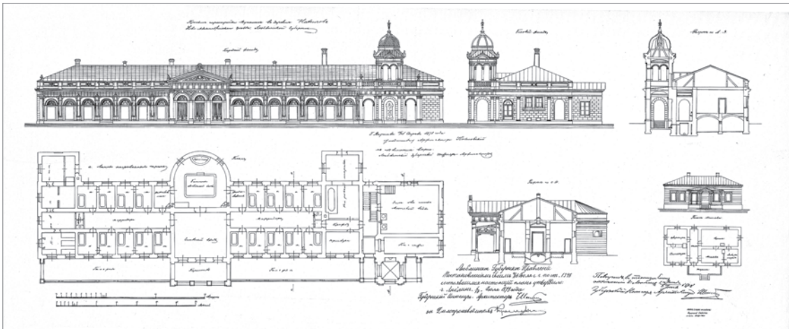
Il. 109. Projekt rozbudowy Starych Łazienek z 1878 r., autorstwa K. Kozłowskiego, 1878, rys. R. Jaruga, źródło: archiwum LWKZ
