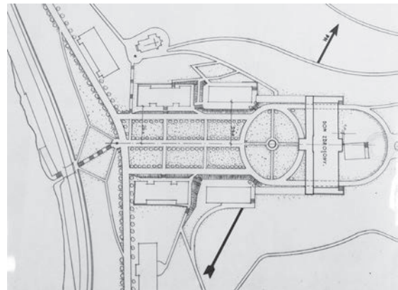
Il. 25. Żegiestów Zdrój. Nowy dom zdrojowy, 1928, proj. A. Szyszko-Bohusz, perspektywa i fragment planu sytuacyjnego. Źródło: ANK, Sz-Boh, sygn. 222
