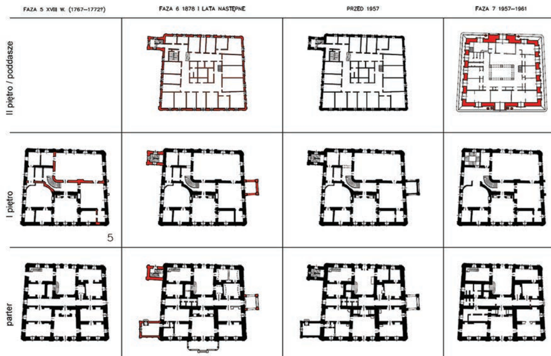
Il. 104. Fazy przebudowy pałacu Małachowskich od XVIII wieku do 1961. Oprac. W. Pawlak na podstawie: A. Kasi-borski, M. Stasiak, Badania architektoniczne, Nałęczów, Pałac Małachowskich, Chronologiczne rozwarstwienie faz budowy, 1985
