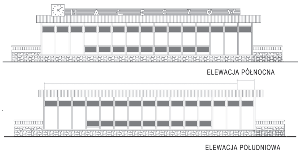
Il. 85. Projekt pawilonu dworca PKS – elewacja południowa i północna, oprac. N. Przesmycka na podstawie dokumentacji archiwalnej w posiadaniu LWKZ
