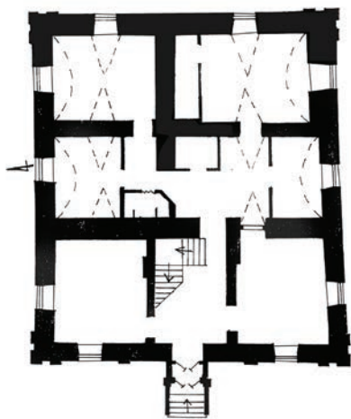
Il. 107. Rzut parteru starego pałacu na podstawie karty ewidencyjnej zabytku, po prawej: lata 70. XX wieku przebudowa oficyny, fot. S. Butrym, źródło: Miejsko-Gminna Biblioteka Publiczna im. Faustyny Morzyckiej w Nałęczowie
