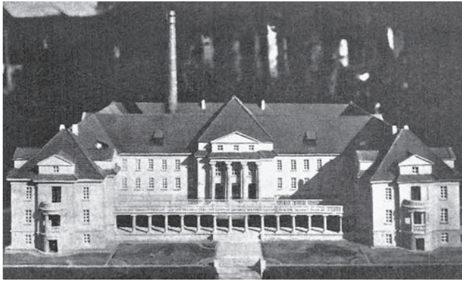
Il. 18. Nowe łaźienki w Krynicy, widok ogólny i rzut parteru, źródło: „Architektura i Budownictwo”, 1926, z. 10–11
