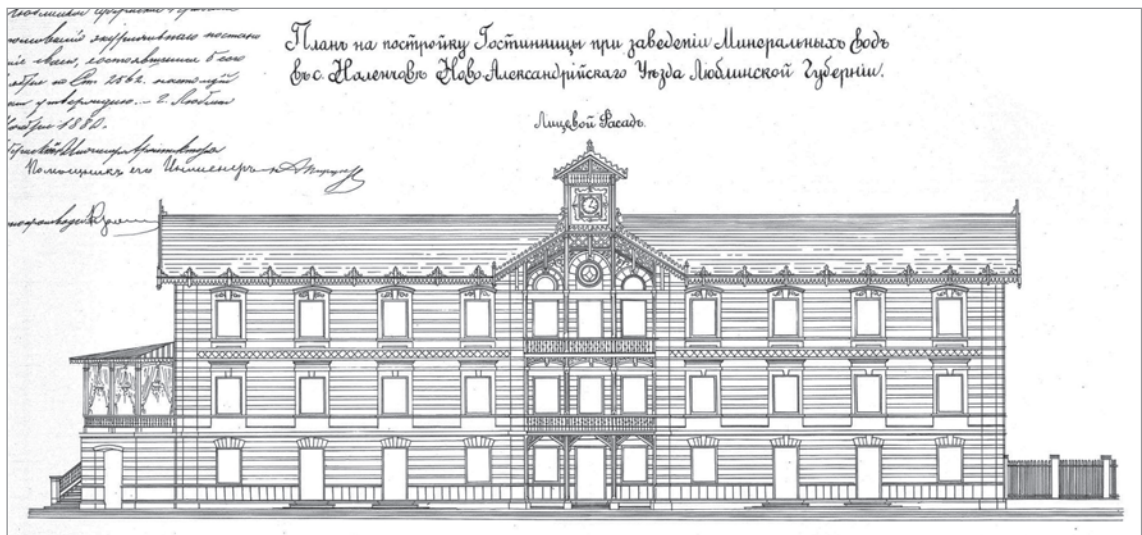
Il. 121. Budynek hotelu dla gości. Projekt K. Kozłowski, 1889, przerys R. Jaruga, źródło: archiwum LWKZ
