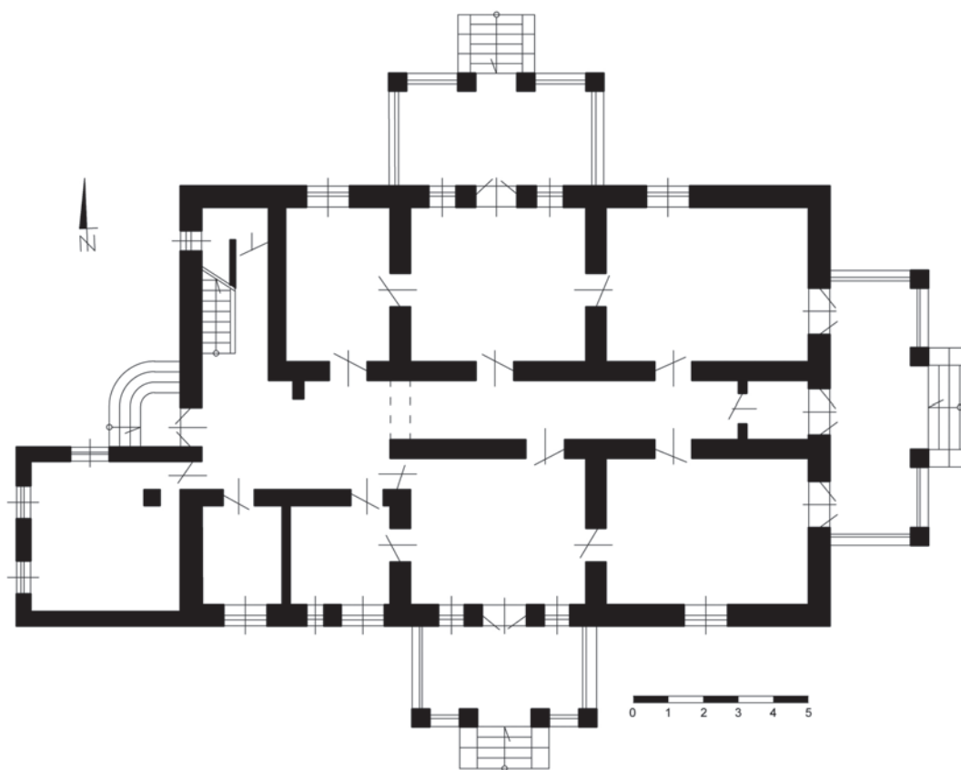
Il. 157. Schemat rzutu parteru willi „Uciecha”, źródło: archiwum KAUiPP
