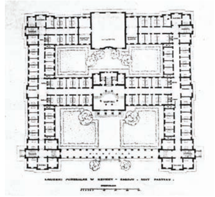
Il. 18. Nowe łaźienki w Krynicy, widok ogólny i rzut parteru, źródło: „Architektura i Budownictwo”, 1926, z. 10–11
