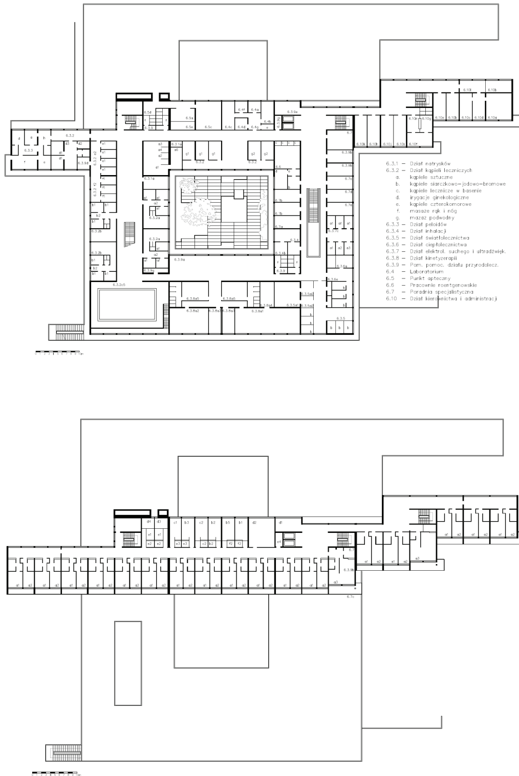
Il. 209. Schematy rzutów parteru (wyżej) i piętra (niżej), na podstawie projektu S. Fijałkowskiego, oprac. W. Pawlak
