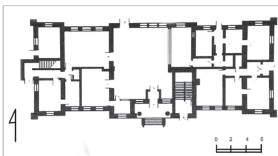
Il. 70. Budynek dworca kolejowego w Nałęczowie, źródło: NAC, po prawej schemat rzutu parteru, źródło: archiwum KAU i PP
