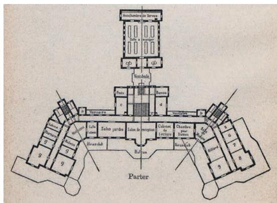
Il. 31. Schemat rzutów sanatorium w Hohenhonnef i w Zakopanem – porównanie, źródło: H. Dobrzycki, Sanatorium dla chorych piersiowo w Zakopanem , 1903
