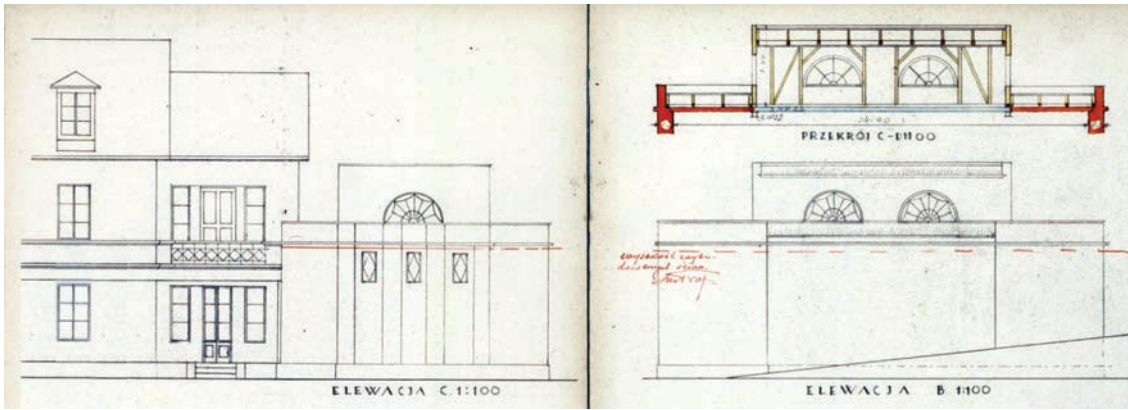
Il. 119. Projekt rozbudowy hydroterapii z lat 30. XX wieku o część kąpielową z pomieszczeniami mieszkalnymi (na poddaszu). Fragment, źródło: APL, UWL, sygn. 1946
