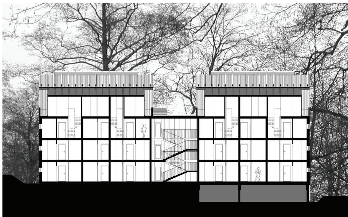
Il. 217. „Jesienna Rezydencja”, schemat rzutu kondygnacji przyziemia i przekrój podłużny, źródło: Biuro Architektoniczne Stelmach i Partnerzy
