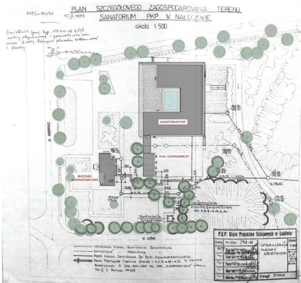
Il. 190. Zagospodarowanie terenu Kolejowego Szpitala Kardiologicznego, oprac. K. Krupa, na podstawie projektu architektonicznego z zasobów LWKZ Lublin
