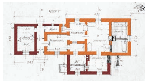
Il. 141. Projekt rozbudowy łaźni im. B. Prusa w Nałęczowie, pow. puławski, proj. architekt powiatowy inż. Zygmunt Trojanowski. Źródło: APL, UWL, KBJ, sygn. 1952
