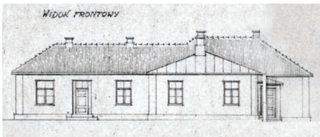
Il. 141. Projekt rozbudowy łaźni im. B. Prusa w Nałęczowie, pow. puławski, proj. architekt powiatowy inż. Zygmunt Trojanowski. Źródło: APL, UWL, KBJ, sygn. 1952
