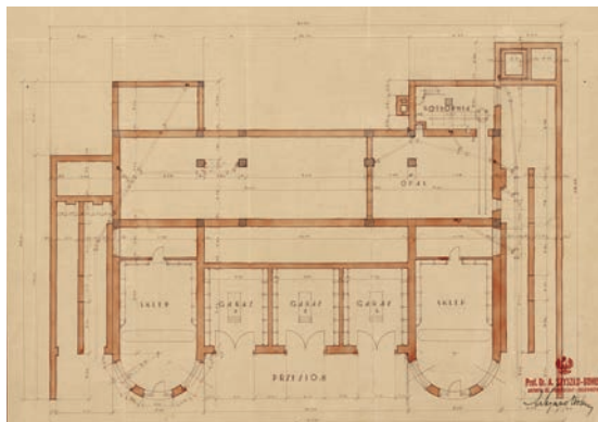
Il. 49. Projekt pensjonatu dla dra Bielińskiego w Krynicy, proj. A. Szyszko-Bohusz, ANK, Sz-Boh, sygn. 232_3-6
