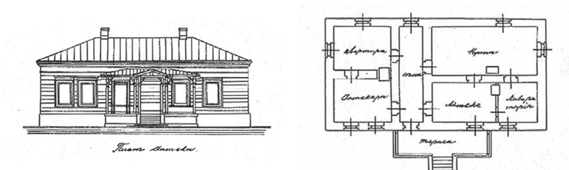
Il. 127. Domek Biskupi – projekt przebudowy autorstwa K. Kozłowskiego, 1878, rys. R. Jaruga, źródło: archiwum LWKZ
