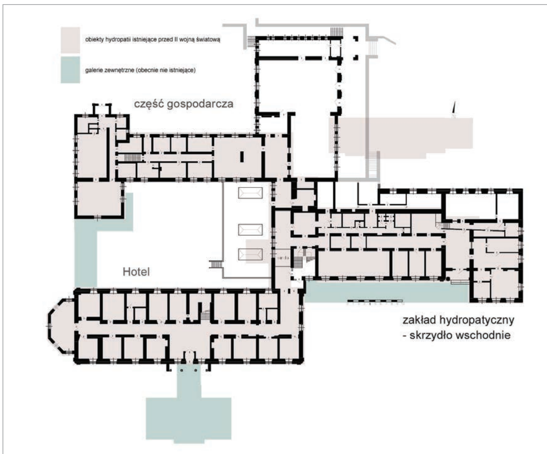
Il. 120. Układ funkcjonalny parteru budynków zakładu hydroterapii i hotelu. Rys. N. Przesmycka na podstawie Karty Ewidencyjnej Zabytku
