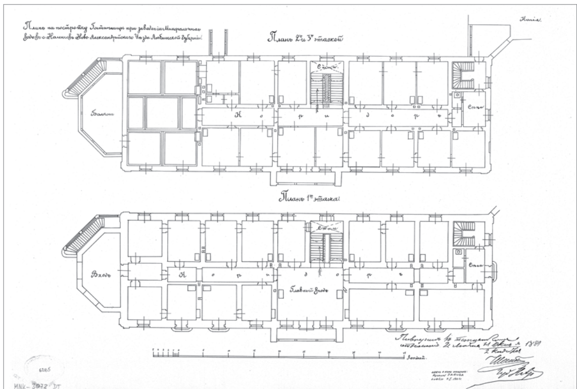
Il. 122. Hotel – rzuty parteru i piętra, proj. K. Kozłowski, 1889, przerys R. Jaruga, źródło: archiwum LWKZ
