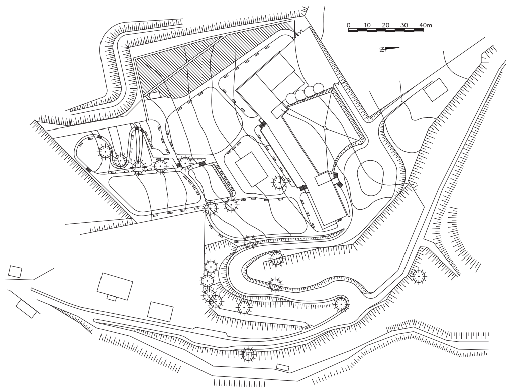
Il. 201. Zagospodarowanie terenu Sanatorium ZNP. Oprac. na podstawie dokumentacji projektowej W. Pawlak
