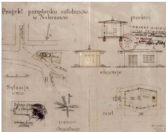
Il. 71. Przystanek autobusowy, projekt, źródło: APL, UWL, 1938, sygn. 1965, po prawej przystanek w 1956 roku, fot. J. Szandomirski, źródło: archiwum LWKZ
