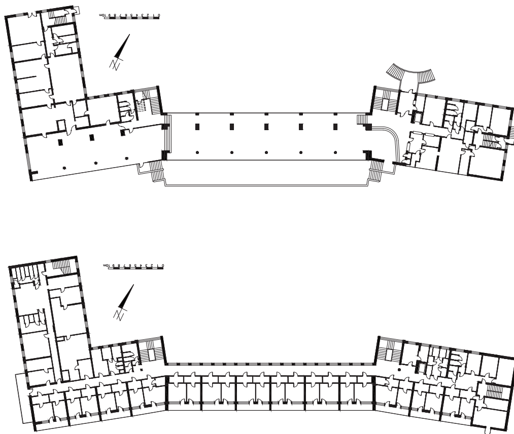
Il. 202. Schemat rzutów parteru i I piętra Sanatorium ZNP. Oprac. na podstawie dokumentacji projektowej W. Pawlak
