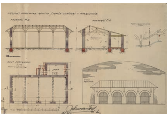
Il. 73. Projekt przebudowy remizy strażackiej w Nałęczowie, APL, UWL, sygn. 1959, oraz budynek straży pożarnej w latach 60. XX wieku, źródło: Miejsko-Gminna Biblioteka Publiczna im. Faustyny Morzyckiej w Nałęczowie
