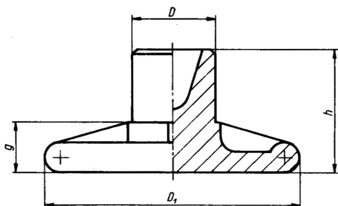
Rys. 1. Podstawka wsuwana W
