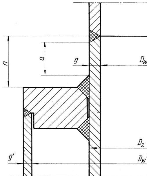
Rys. Z-3. Rozwiązanie dla g'_{max} > 16 \text{ mm}
