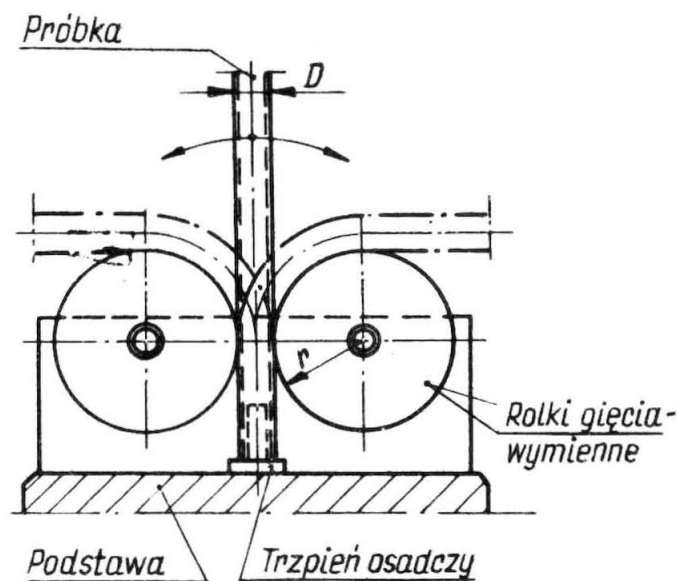
Rys. 7. Przyrząd do zginania rur karbowanych
