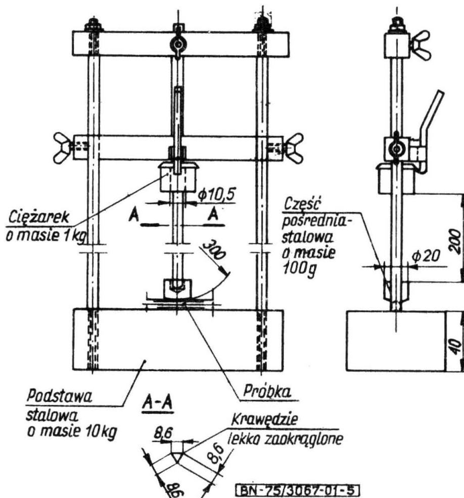
Rys.5. Przyrząd do próby odporności na uderzenia rur
