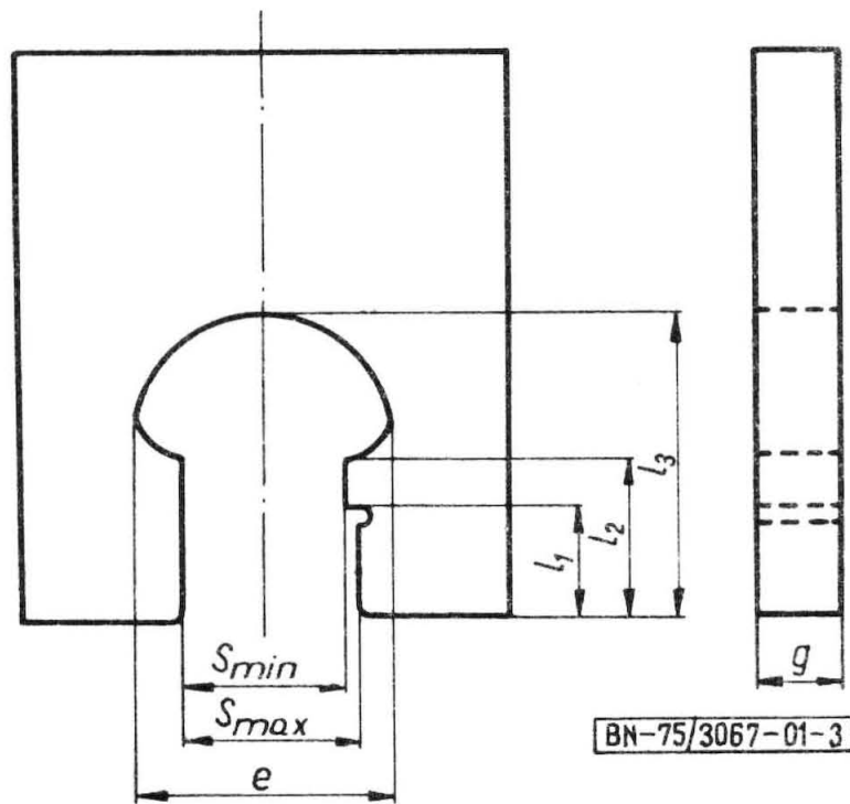
Rys. 3. Sprawdzian średnicy zewnętrznej rur
