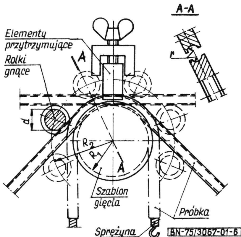
Rys. 6. Przyrząd do zginania rur sztywnych
