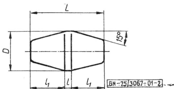
Rys. 2. Sprawdzian średnicy wewnętrznej rur karbowanych
