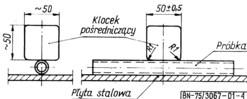
Rys. 4. Przyrząd do próby zgniatania
