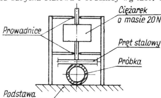
Rys. 9. Przyrząd do badania twardości rur i złązek karbowanych
