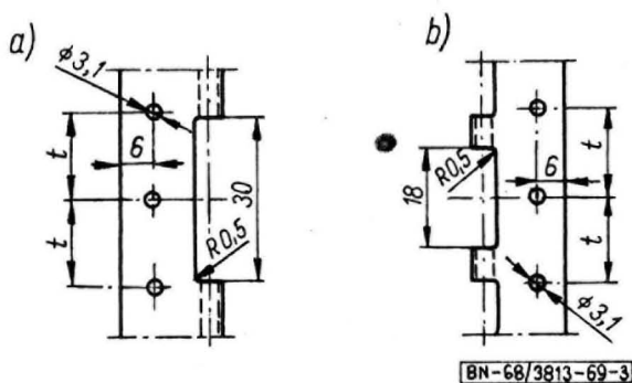
Rys. 3. Wycięcia skrzydeł i otwory pod nity
