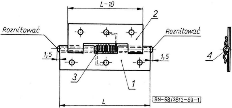
Rys. 1. Zawiasa
