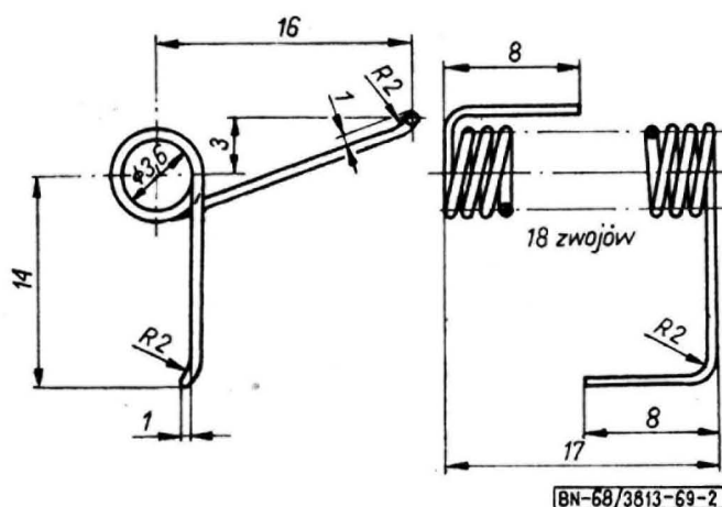
Rys. 2. Sprężyna odciągająca
