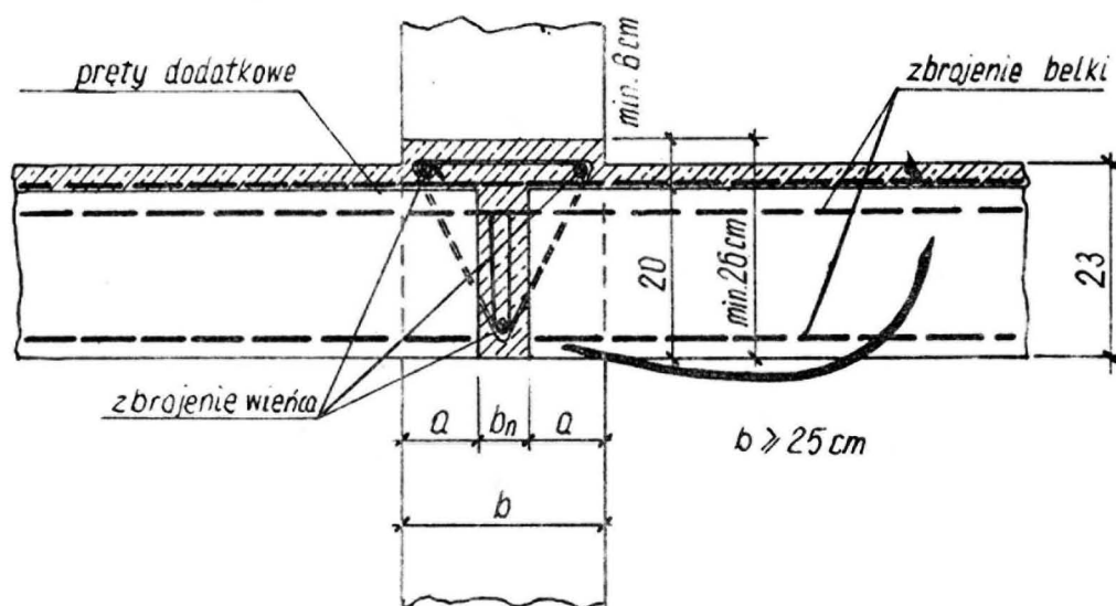
Rys. 11 Oparcie stropów częściowo zamocowanych na ścianach
