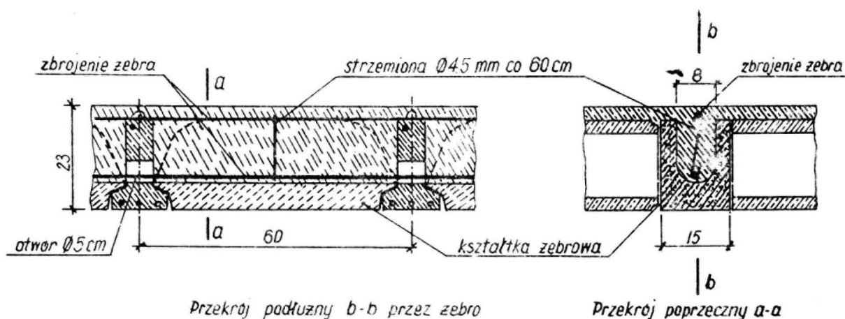
Rys.2 Żebro rozdzielcze
