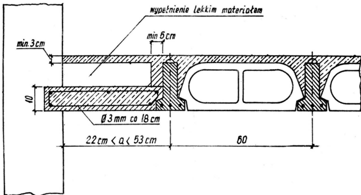
Rys. 5 Przesklepienie płytą betonową, wykonywaną na budowie
