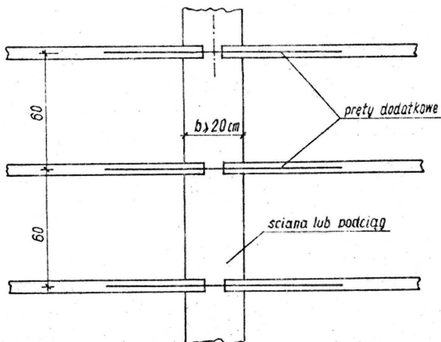
Rys.9. Belki DZ-3 ułożone w jednej osi
