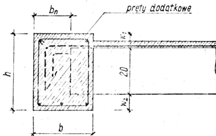
Rys.12. Oparcie stropów częściowo zamocowanych na podciągach
