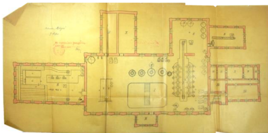
Ryc. 192. Projekt budynku rafinacji cukrowni w Milejowie. Rzut I, II i III piętra (APL UWL w. kom. – bud. sygn. 346).
