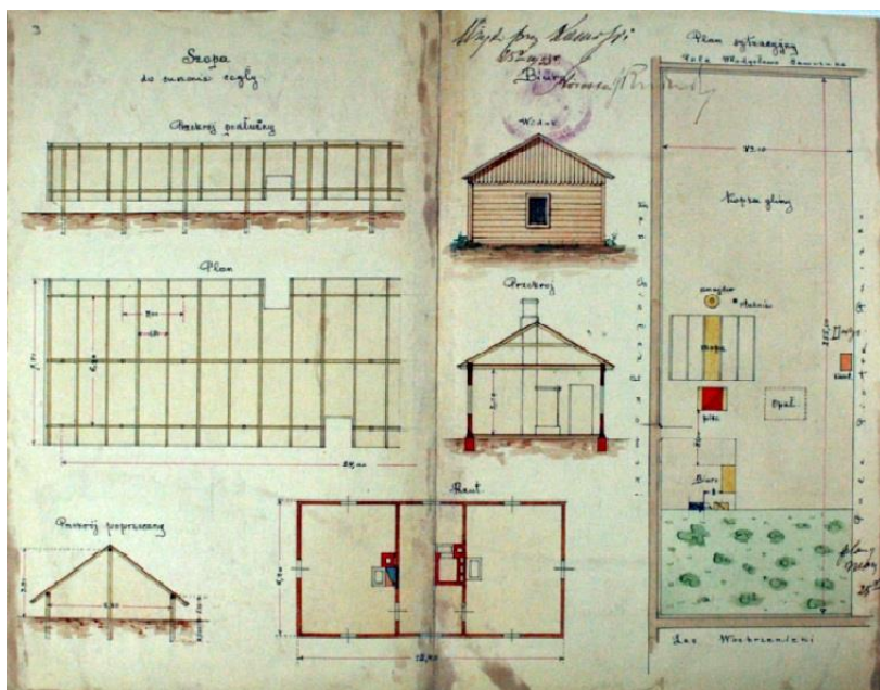
Ryc. 31. Projekt wiaty do suszenia cegły we wsi Kalitków z 1923 r. (APL, UWL w. kom.-bud. Sygn. 333).
