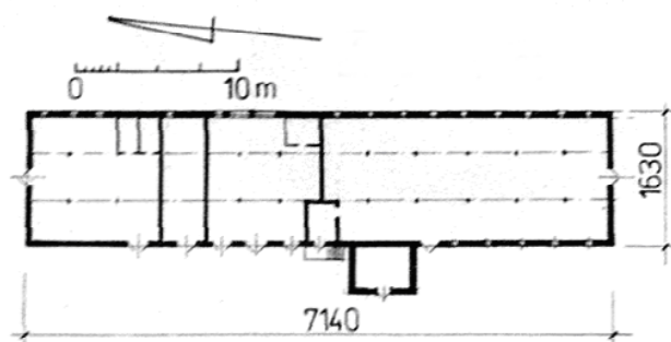
Ryc. 269. Wierzchowiska, obora, rzut przyziemia, inwentaryzacja. Stan w 2003 roku. Opr. autor.
