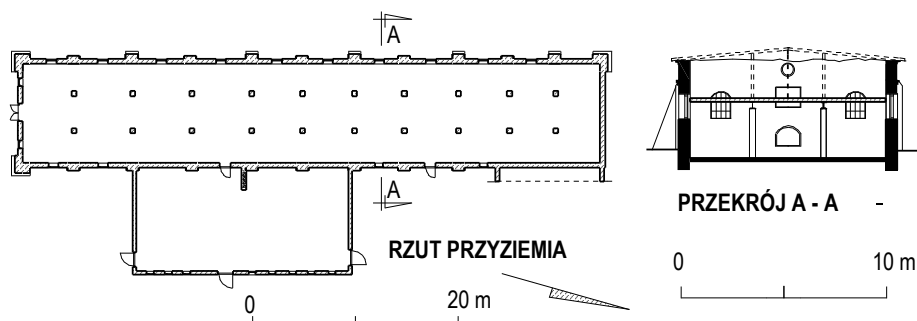
Ryc. 94. Brzezice, obora, inwentaryzacja, rzut przyziemia i przekrój A – A. Stan w 2003 roku. Opr. autor.
