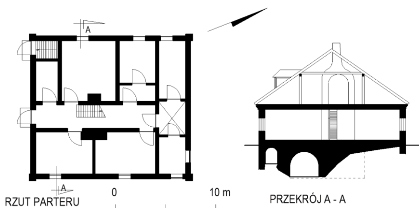
Ryc. 107. Kuchnia dworska, inwentaryzacja, rzut parteru i przekrój A-A. Stan w 2003 roku. Opr. autor.
