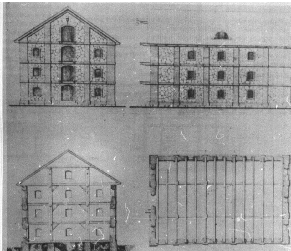
Ryc. 17. Projekt spichlerza w Janowie Podlaskim wykonany przez H. Marconiego w 1839 roku (Za J. Dumnicki, Spichlerze polskie , Warszawa, 1987r. rys. 200).
