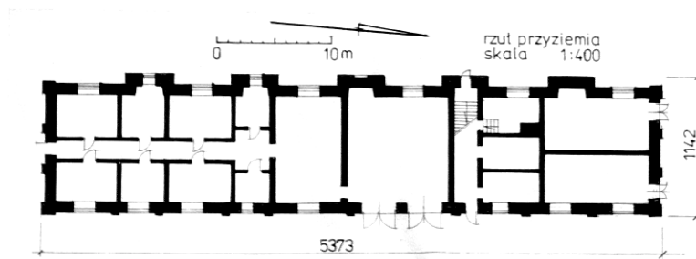
Ryc. 258. Wierchowiska, stajnia, rzut przyziemia, inwentaryzacja. Stan w 2003 roku. Opr. autor.
