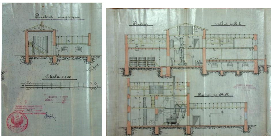
Ryc. 163. Jabłonna, projekt gorzelni przekroje pionowe, (APL, UWL w. kom. – bud. Sygn. 353).
