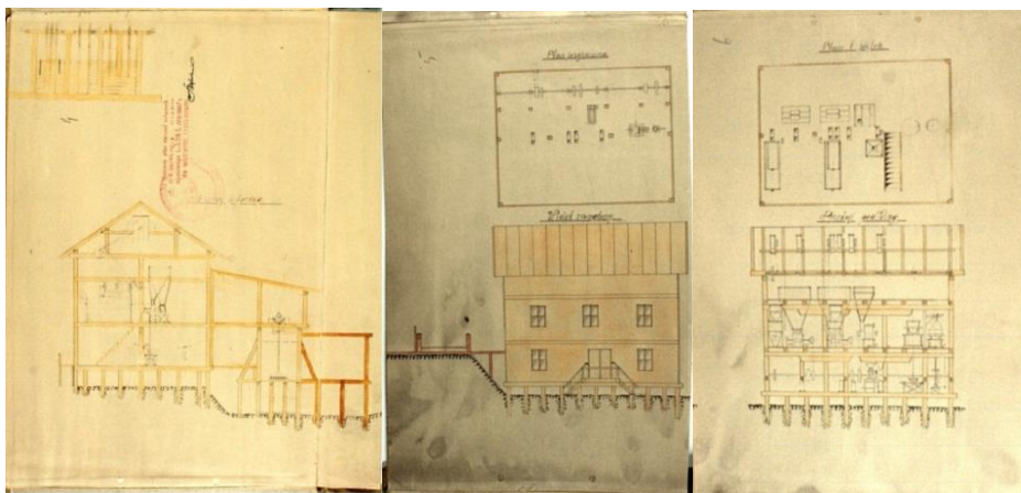
Ryc. 58. Projekt młyna i tartaku parowego w Czemiernikach (APL, UWL w. kom.-bud. sygn. 444).
