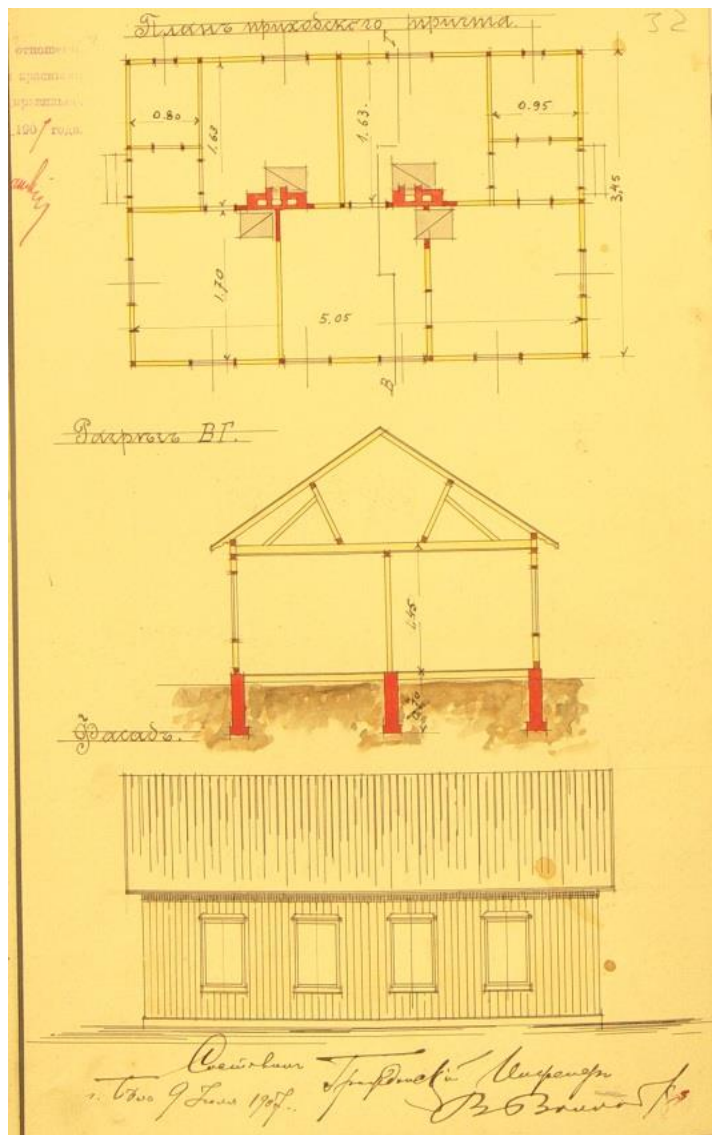
Ryc. 62. Projekt domu mieszkalnego dla dwóch rodzin pracowników folwarcznych w folwarku Ostrówki. (APL, RGS sygn. 295).
