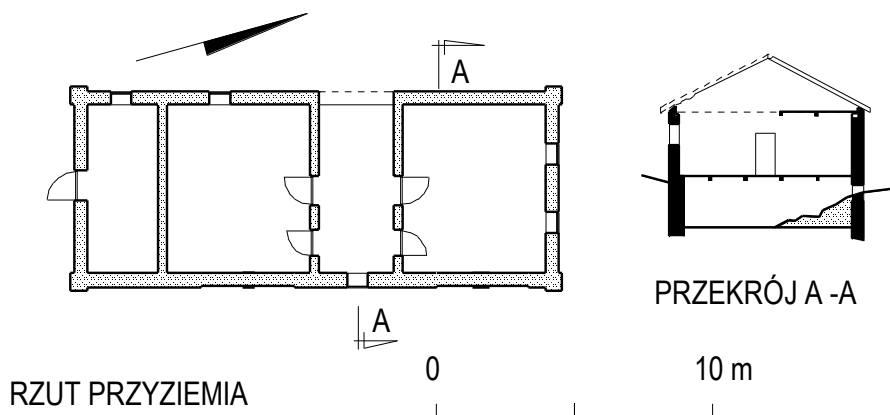
Ryc. 104. Brzezice, oranżeria, inwentaryzacja, rzut przyziemia i przekrój A-A. Stan w 2003 roku. Opr. autor.
