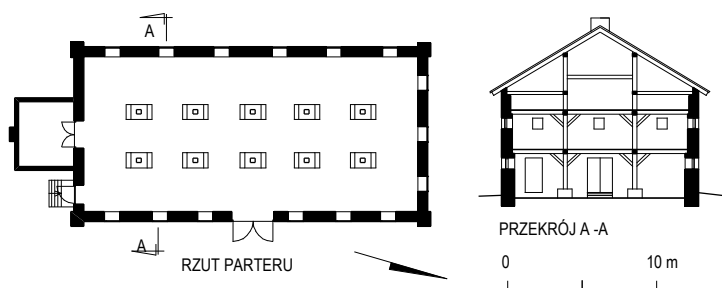
Ryc. 98. Brzezice, stodoła, inwentaryzacja, rzut przyziemia i przekrój A-A. Stan w 2003 roku. Opr. autor.
