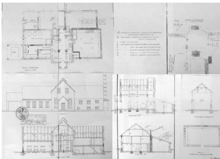
Ryc. 34. Zabudowania gorzelni i magazynu spirytusu w folwarku „Kłątwy” (APL UWL, wyd. kom.- bud. Sygn. 251).
