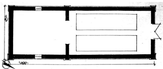
Ryc. 83. Bojanówka, magazyn spirytusu, rzut parteru, inwentaryzacja. Stan w 2005 roku. Opr. autor.
