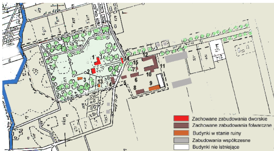
Ryc. 86. Brzezice, plan sytuacyjny folwarku.. Oznaczenia: 1- pałac, 2- kuchnia dworska, 3-oranżeria, 4-stajnia dworska, 5-ruiny kuźni, 6-spichlerz, 7-stelmarnia, 8-stodoła, 9-fundamenty stodoły, 10- obora, 11-stajnia fornalska, 12-obora, 13- ruiny lodowni, 14- brama, 15- fragment muru. Stan w 2003 roku. Opr. autor.
