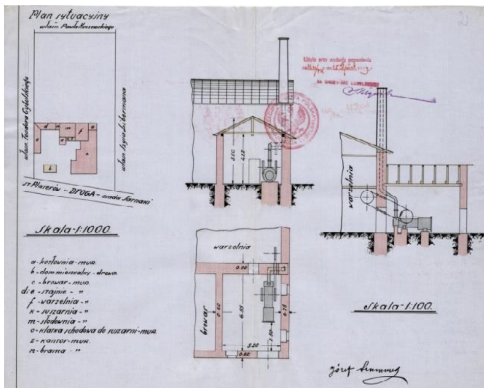
Ryc. 45. Projekt kotłowni parowej i plan sytuacyjny browaru w Sarnakach (APL, UWL w. kom.-bud. Sygn. 109).
