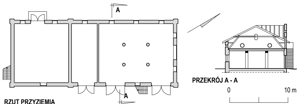
Ryc. 87. Brzezice, stajnia koni wierzchowych, inwentaryzacja, rzut parteru i przekrój A-A. Stan w 2003 roku. Opr. autor.
