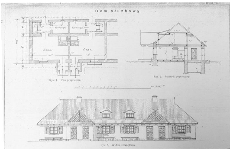
Ryc. 61. Projekt „nowoczesnego” budynku dla służby folwarczej, wg arch. B. Rogaczewskiego, 1915 r.
