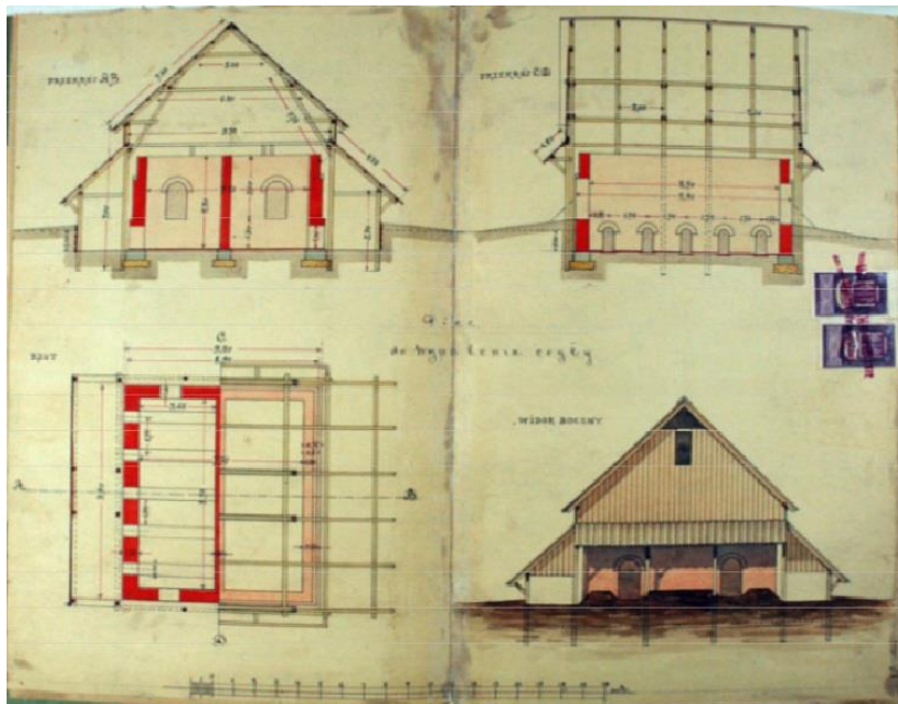
Ryc. 30. Projekt pieca do wypalania cegły we wsi Kalitków (APL, UWL w. kom.-bud. Sygn. 333).
