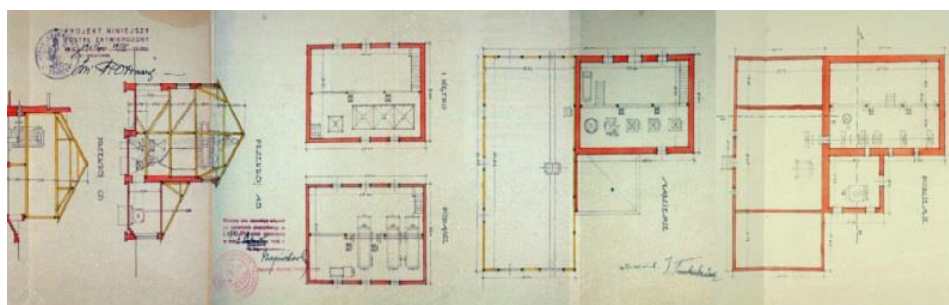
Ryc. 59. Projekt młyna i tartaku parowego w Czemiernikach (APL, UWL w. kom.-bud. sygn. 444).
