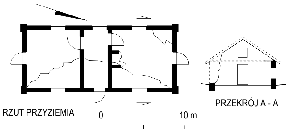
Ryc. 102. Brzezice, kuźnia, inwentaryzacja, rzut przyziemia i przekrój A-A. Stan w 2003 roku. Opr. autor.
