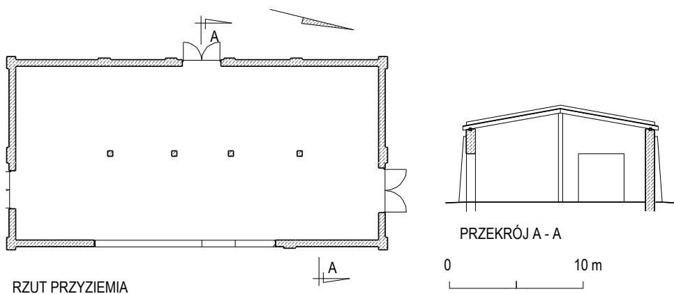
Ryc. 96. Brzezice, stodoła, inwentaryzacja, rzut przyziemia i przekrój A – A. Stan w 2003 roku. Opr. autor.
