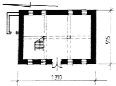
Ryc. 265. Wierchowiska, spichlerz, rzut przyziemia, inwentaryzacja. Stan w 2003 roku. Opr. autor.
