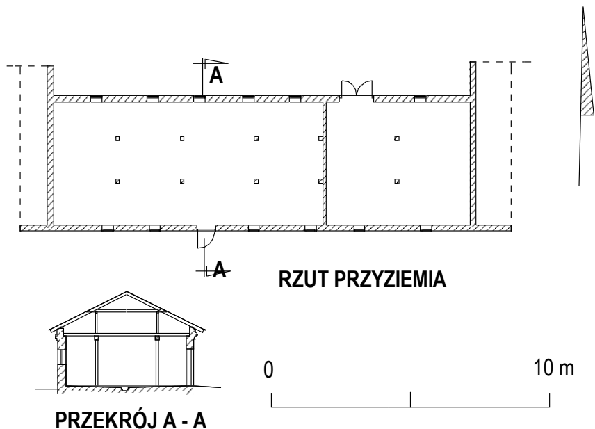
Ryc. 90. Brzezice, stajnia koni pociągowych, inwentaryzacja, rzut przyziemia i przekrój A-A. Stan w 2003 roku. Opr. autor.
