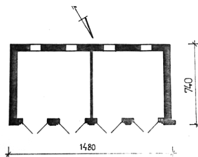
Ryc. 116. Bystrzyca, wozownia, inwentaryzacja, rzut parteru. Stan w 1984 roku. Opr. R. Gapski.
