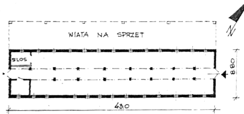
Ryc. 246. Turka, rzut parteru, inwentaryzacja. Stan w 2003 roku. Opr. Autor.
