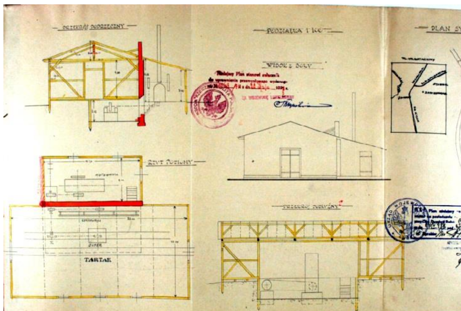
Ryc. 23. Projekt tartaku parowego w miejscowości Annówka z 1928 r. APL, UWL w kom.- bud. Sygn. 315).
