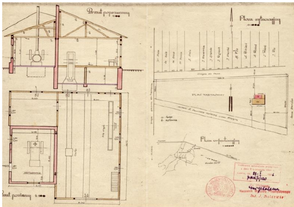
Ryc. 20. Plany tartaku parowego w Konstantowie z 1936 r. (APL, UWL w. kom.-bud. Sygn.83).
