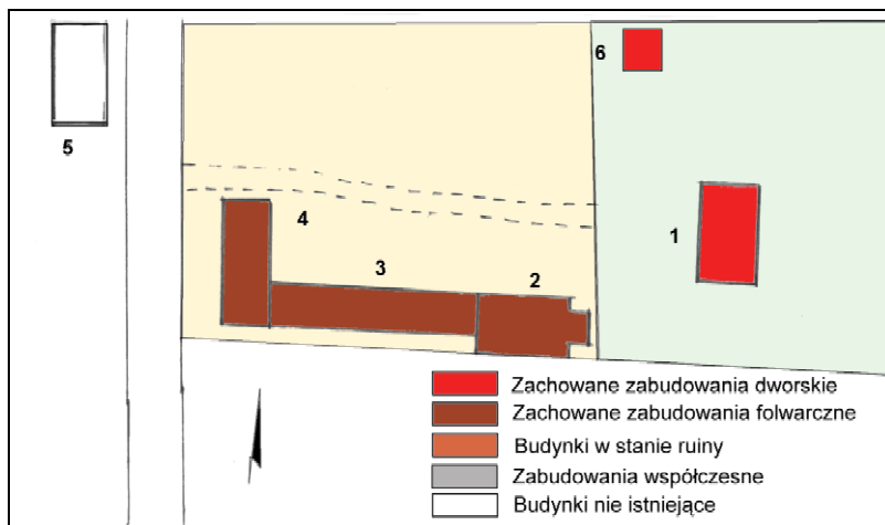
Ryc. 68. Babianka, plan sytuacyjny folwarku. Oznaczenia: 1- rządcówka, 2- spichlerz, 3- obora, 4- stajnia, 5- nieistniejące czworaki, 6- stróżówka. Stan w 2003 roku. Opr. autor.
