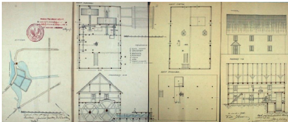
Ryc. 52. Projekt młyna wodnego w dobrach Kockich (APL, UWL w. kom.-bud. sygn. 459).
