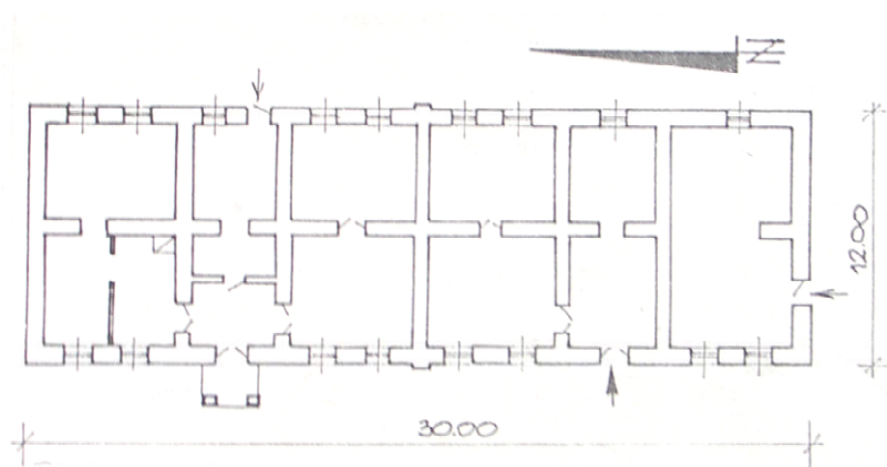
Ryc. 144. Jabłonna. Rzut przyziemia. Inwentaryzacja. Opr. autor za W. Boruch.
