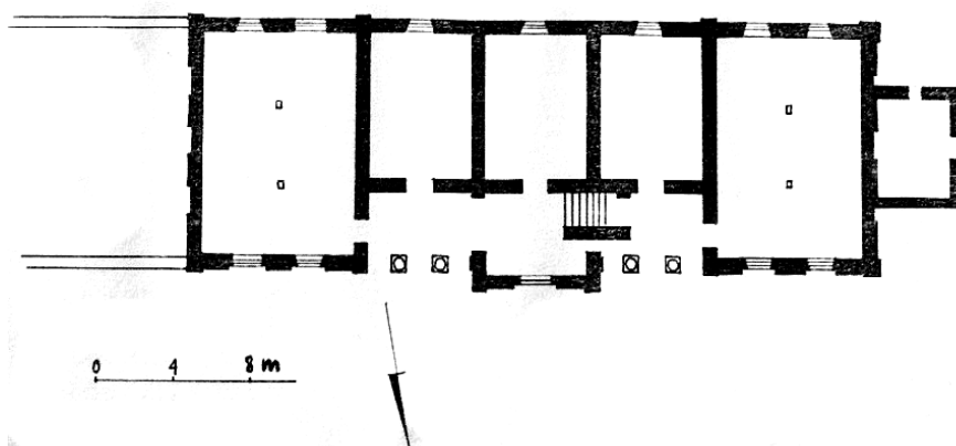
Ryc. 205. Pilaszkowice. Rzut parteru spichlerza. Inwentaryzacja. Stan w 2003 roku. Opr. autor.
