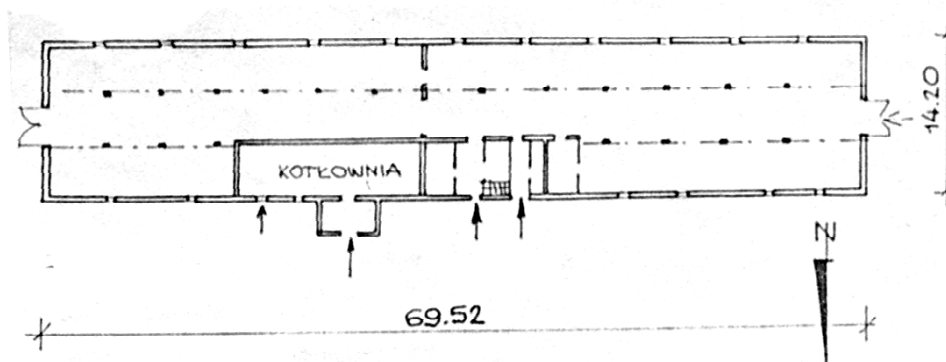
Ryc. 148. Jabłonna. Rzut przyziemia. Inwentaryzacja. Opr. autor, za W. Boruch.
