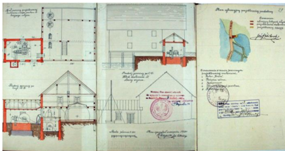
Ryc. 53. Projekt młyna wodnego w dobrach Kockich (APL, UWL w. kom.-bud. sygn. 459).
