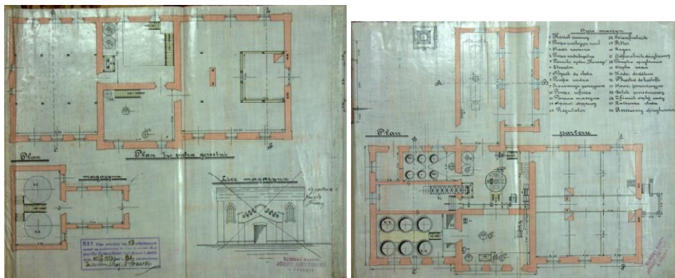
Ryc. 162. Jabłonna, projekt gorzelni, rzuty poziome, (APL, UWL w. kom. – bud. Sygn. 353).
