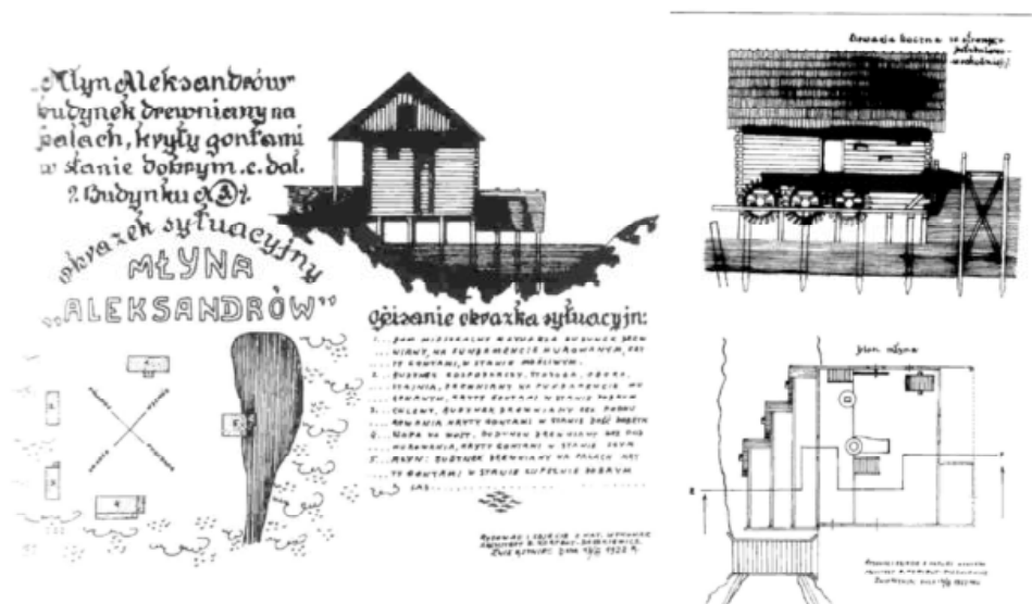
Ryc. 55. Młyn wodny w Aleksandrowie z 1922 roku (APL, AOZ 1029).
