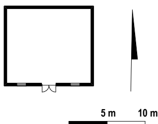
Ryc. 214. Pilaszkowice. Rzut parteru magazynu spirytusu. Inwentaryzacja. Stan w 2003 roku. Opr. autor.
