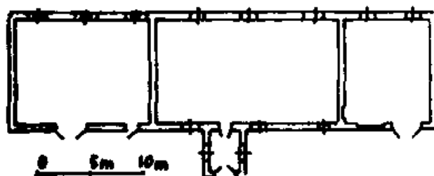
Ryc. 239. Stryjno. Rzut parteru stajni i wozowni. Inwentaryzacja. Stan w 2004 roku. Opr. autor za Z. Pastuszek.
