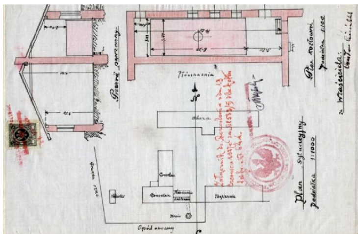
Ryc. 32. Plan sytuacyjny gorzelni w Kębłowie i projekt kotłowni parowej. (APL, UWL w. kom.-bud. Sygn. 128).
