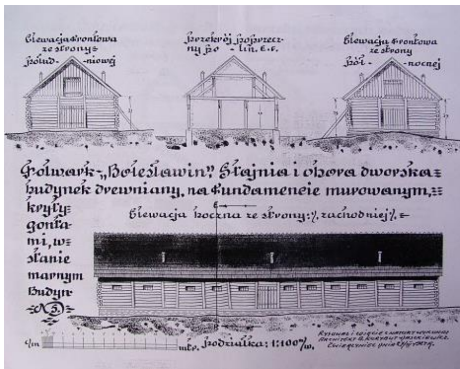
Ryc. 19. Inwentaryzacja stajni i obory w folwarku Bolesławin (AOZ, Plany, sygn. 1030/1).
