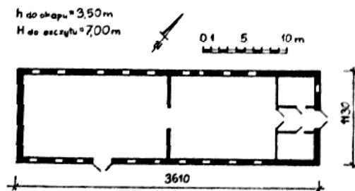
Ryc. 129. Bystrzyca, stajnia. Inwentaryzacja rzut parteru. Stan z 1984 roku, opr. R. Gapski.
