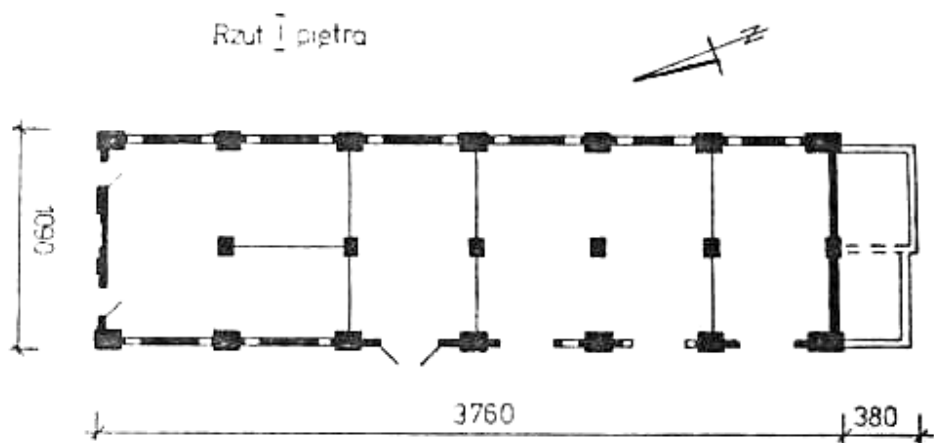
Ryc. 120. Bystrzyca, obora, inwentaryzacja, rzut I piętra. Stan w 1984 r. Rys. R. Gapski.
