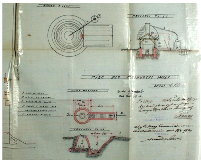
Ryc. 26. Projekt smolarni w folwarku Marianka (APL, UWL w. kom.-bud. Sygn. 334).
