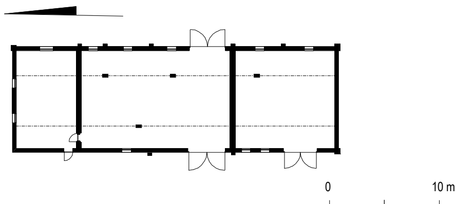
Ryc. 73. Babianka, rzut parteru stajni, inwentaryzacja. Stan w 2003 roku. Opr. autor.
