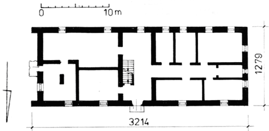
Ryc. 254. Wierchowiska, czworaki, rzut parteru, inwentaryzacja. Stan z 2003 roku. Opr. autor.
