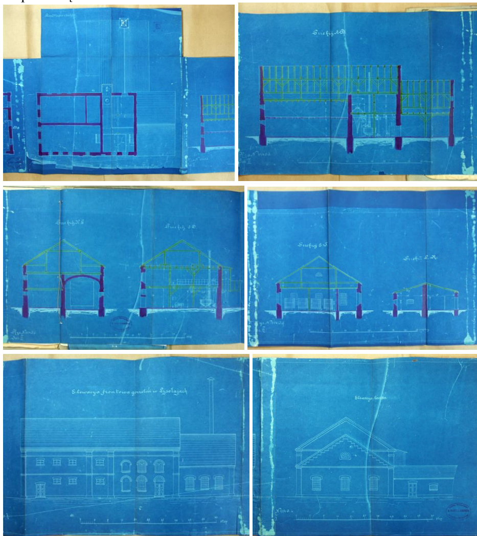
Ryc. 174. Projekt gorzelni w Łysolajach (APL, UWL w. kom. – bud. sygn. 354)
