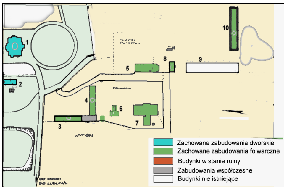
Ryc. 135. Plan sytuacyjny folwarku w Jabłonnej. Oznaczenia: 1- pałac, 2- budynek gospodarczy, 3- stajnia, 4- obora, 5- dom administratora, 6- magazyn spirytusu, 7- gorzelnia, 8- spichlerz, 9- fundamenty dawnej stodoły, 10- obora.. Stan w 2004roku. Opr. autor.
