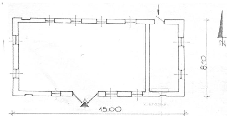
Ryc. 160. Jabłonna. Rzut przyziemia. Inwentaryzacja. Opr. autor, za W. Boruch.
