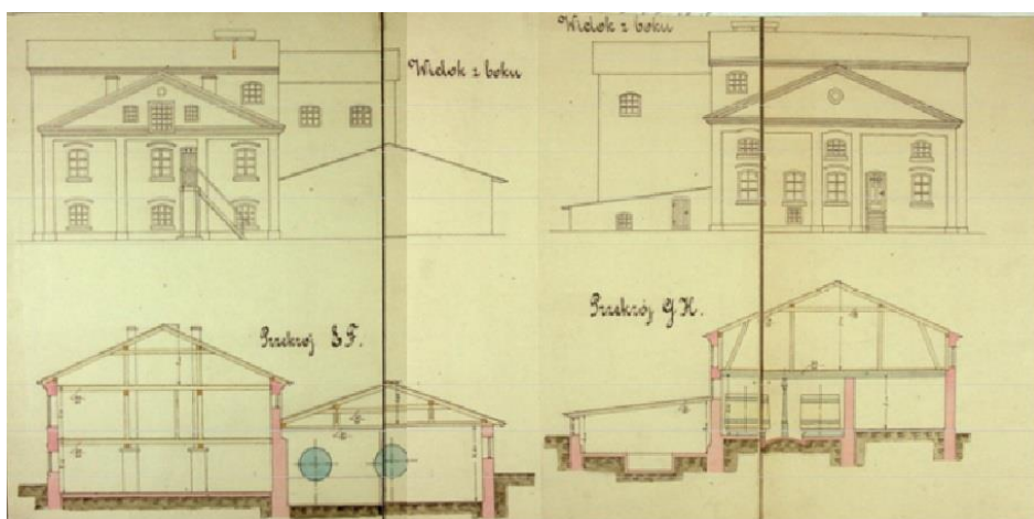
Ryc. 40. Projekt gorzelni w Różance, elewacje i przekroje. (APL UWL w. kom.-bud. sygn. 358).
