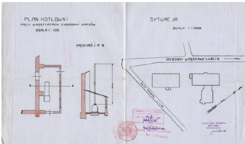
Ryc. 41. Projekt kotłowni parowej i plan sytuacyjny zabudowań cukrowni „Garbów” (APL, UWL w. kom.-bud. Sygn. 116).
