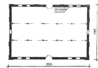
Ryc. 127. Bystrzyca, obora, inwentaryzacja, rzut parteru. Stan w 1984 roku. Opr. R. Gapski.
