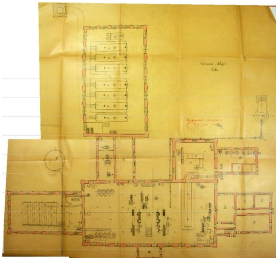
Ryc. 43. Rzut parteru budynku rafinacji cukrowni w Milejowie (APL UWL w. kom.-bud. Sygn. 346).
