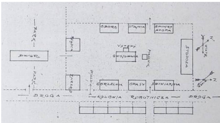
Ryc. 13. Schemat modelowego obejścia gospodarczego wg planów arch. B. Rogaczewskiego. 263
