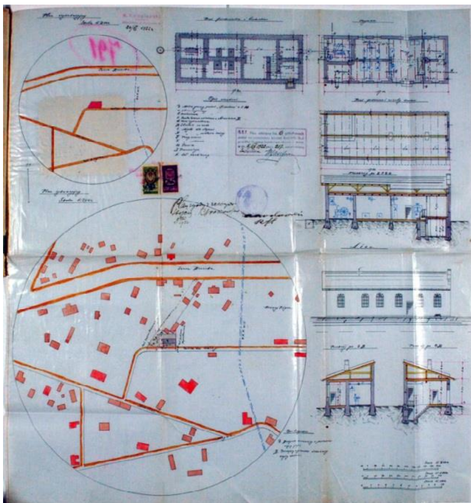
Ryc. 63. Projekt olejarni i kaszarni w Białej Podlaskiej (APL, UWL w. kom.-bud. sygn.311).
