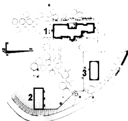
Ryc. 234. Plan sytuacyjny założenia dworsko-folwarcznego w Stryjnie. Oznaczenia: 1- dwór, 2- stajnia z wozownią, 3- oficyna. Stan w 2004 roku. Opr. autor.
