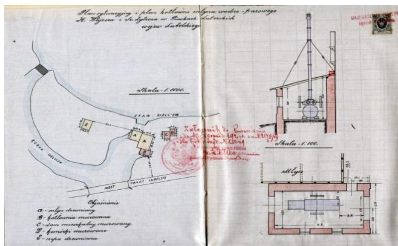
Ryc. 48. Plan sytuacyjny młyna i projekt kotłowni parowej w Piaskach Luterskich (APL, UWL w. kom.-bud. sygn. 141).
