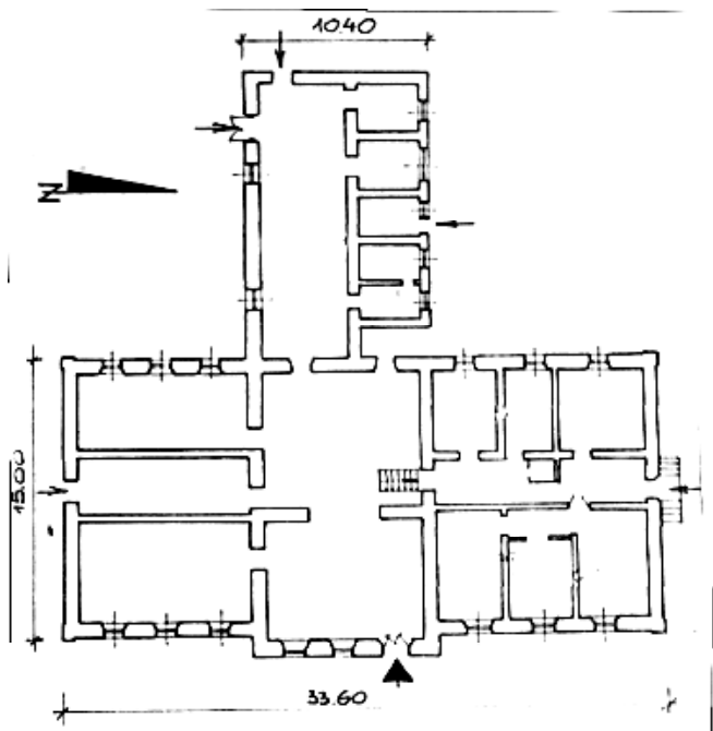
Ryc. 171. Jabłonna. Rzut parteru gorzelni, Inwentaryzacja. Stan w 2003 roku. Opr. autor za W. Boruch
