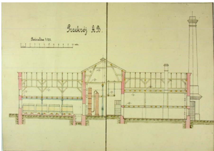
Ryc. 38. Projekt gorzelnii w Różance, przekrój podłużny. (APL UWL w. kom.- bud. sygn. 358).
