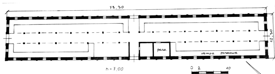
Ryc. 227. Podłódów, obora, rzut parteru, inwentaryzacja. Stan z 2003 roku. Opr. autor.
