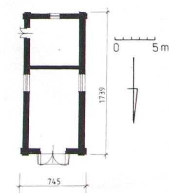
Ryc. 271. Wierzchowska, drewnutnia, rzut przyziemia, inwentaryzacja. Stan w 2003 roku. Opr. autor.
