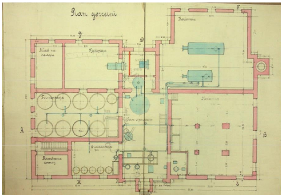
Ryc. 37. Projekt gorzelnii w Różance, rzut parteru. (APL UWL w. kom.-bud. sygn. 358).
