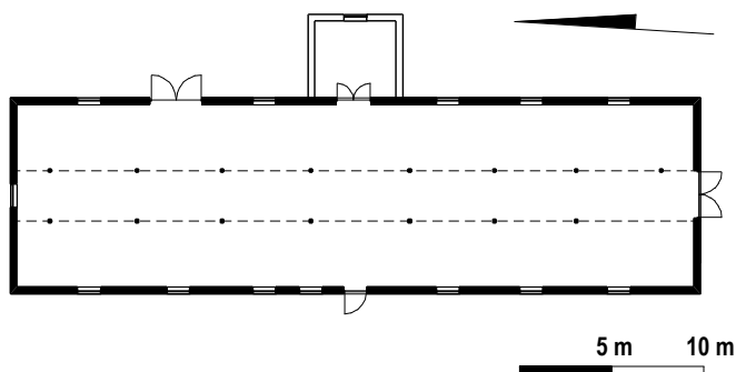
Ryc. 208. Pilaszkowice. Rzut parteru obory. Inwentaryzacja. Stan na 2003 roku. Opr. autor.
