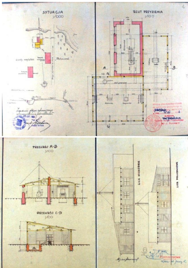
Ryc. 25. Plan sytuacyjny i rzut przyziemia, przekroje i widok elewacji tartaku w miejscowości Potoczek z 1936 r. (APL, UWL w. kom.-bud. Sygn. 356).
