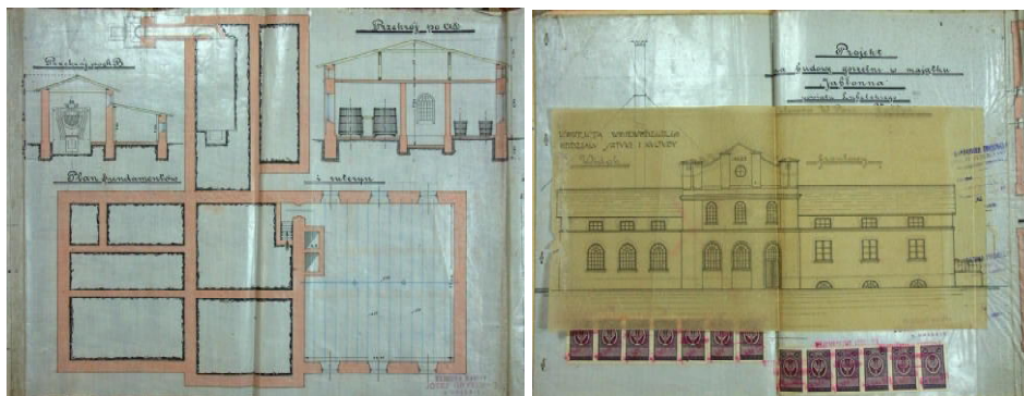
Ryc. 164. Jabłonna, projekt gorzelni, rzut piwnic i elewacja frontowa, (APL, UWL w. kom. – bud. Sygn. 353).
