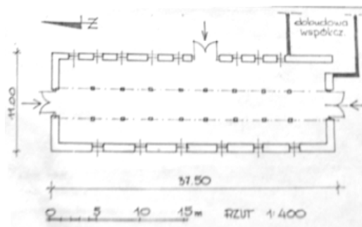
Ryc. 157. Jabłonna. Rzut przyziemia stajni. Inwentaryzacja. Opr. autor, za W. Boruch.
