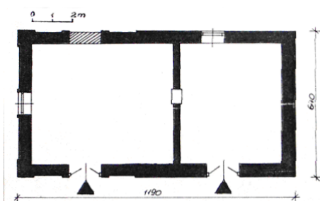
Ryc. 222. Podlodów, stolarsnia. Inwentaryzacja, rzut parteru. Stan w 2005 roku. Opr. autor.
