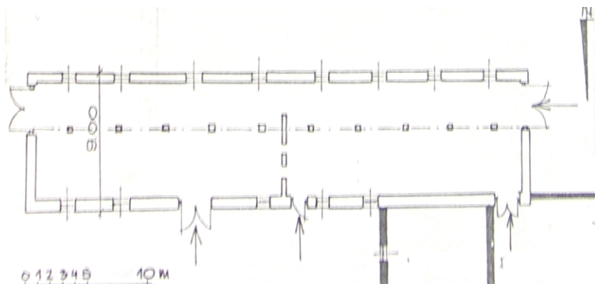
Ryc. 153. Jabłonna. Rzut przyziemia. Inwentaryzacja. Opr. autor, za W. Boruch.
