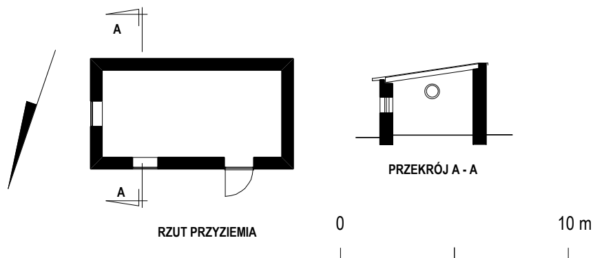
Ryc. 100. Brzeżice, stelmarnia, inwentaryzacja, rzut przyziemia i przekrój A-A. Stan w 2003 roku. Opr. autor.
