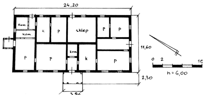
Ryc. 226. Podlodów, oficyna, rzut parteru, inwentaryzacja. Stan w 2003 roku. Opr. autor.
