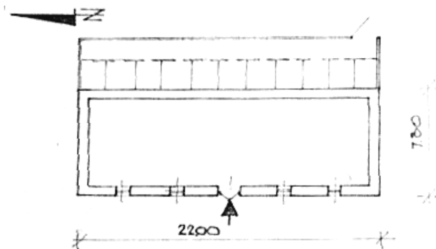
Ryc. 138. Jabłonna. Rzut przyziemia budynku gospodarczego. Inwentaryzacja. Stan w 1988 roku. Opr. autor, za W. Boruch.
