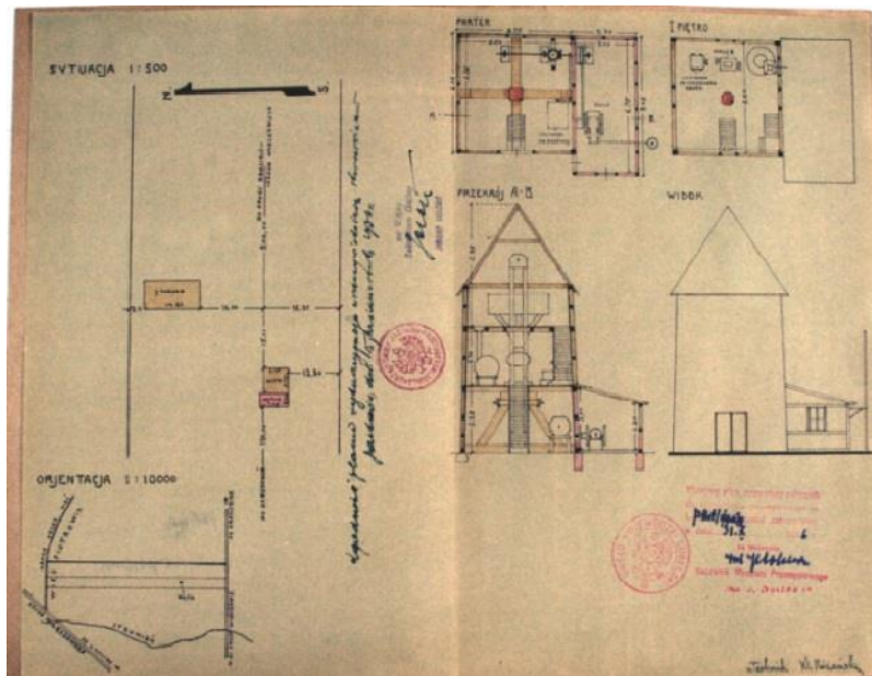
Ryc. 47. Plan sytuacyjny wiatraka w Wierzchowiskach i projekt dobudowania kotłowni parowej. (APL, UWL w. kom.-bud. sygn. 452).
