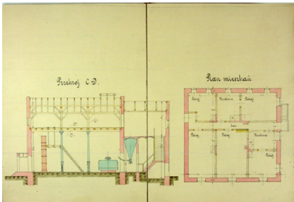
Ryc. 39. Projekt gorzelni w Różance, przekrój poprzeczny i rzut II piętra. (APL UWL w. kom.-bud. sygn. 358).
