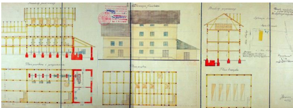
Ryc. 50. Projekt młyna parowego w folwarku Kłutwy (APL, UWL w. kom.-bud. sygn. 482).
