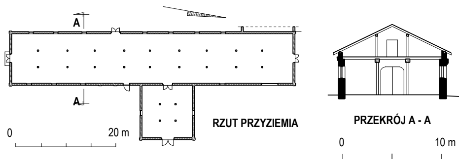
Ryc. 92. Brzezice, obora, inwentaryzacja, rzut przyziemia i przekrój. Stan w 2003 roku. Opr. autor.
