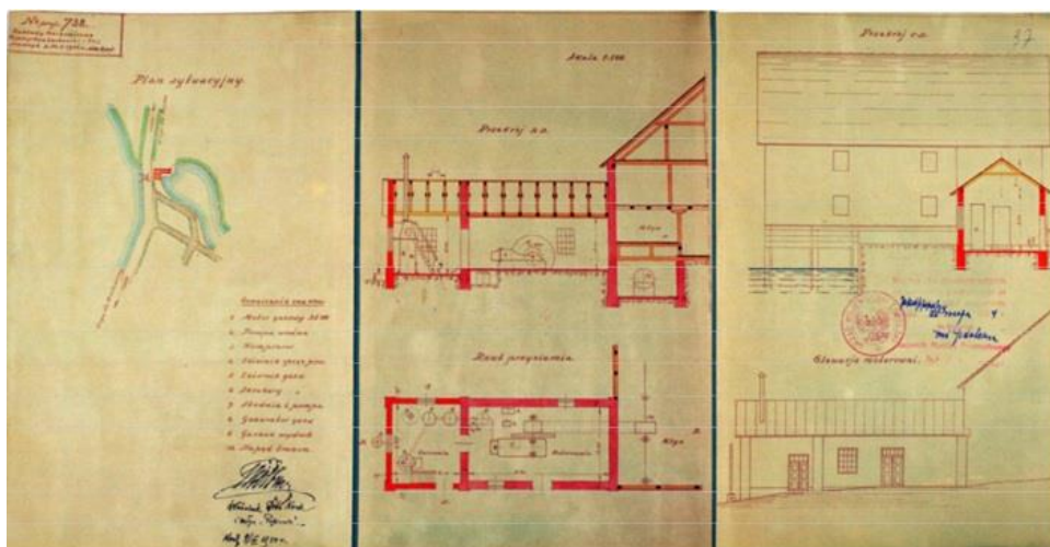
Ryc. 54. Projekt wstawienia kotła parowego do młyna wodnego w dobrach Kockich (APL, UWL w. kom.-bud. sygn. 459).
