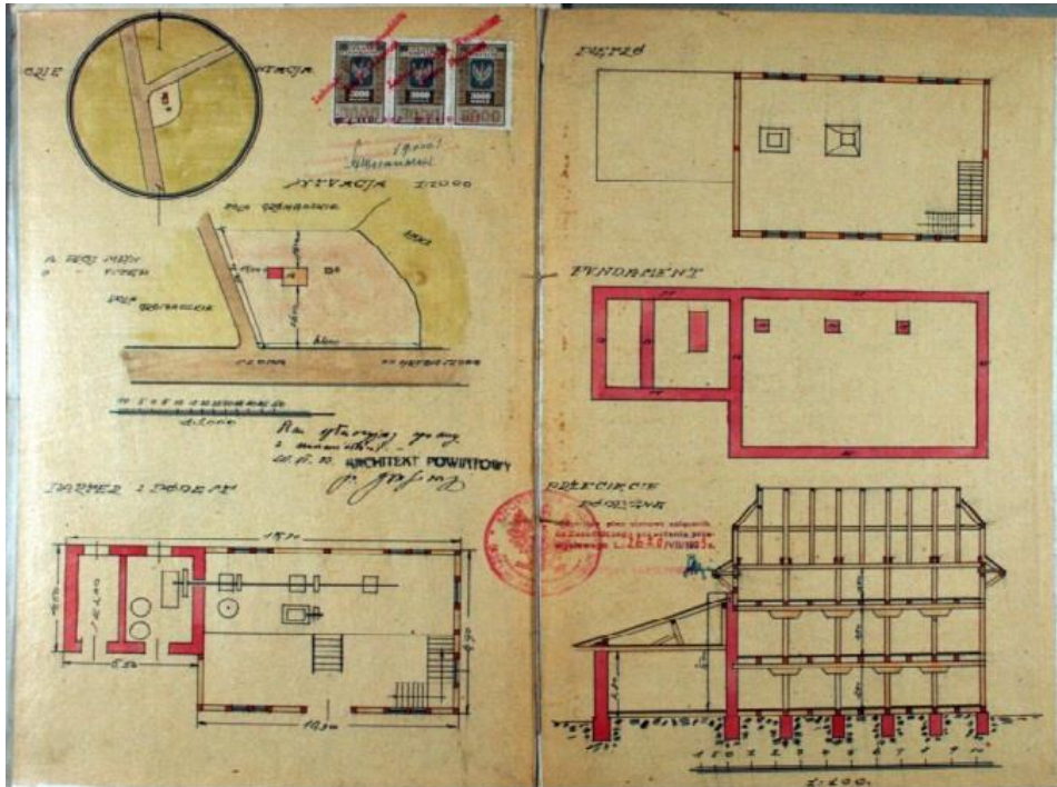
Ryc. 49. Projekt młyna parowego w Mirczu (APL, UWL w. kom.-bud. sygn. 410).
