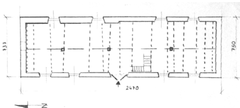
Ryc. 141. Jabłonna. Rzut przyziemia. Inwentaryzacja. Stan w 1988 roku. Opr. autor za W. Boruch.
