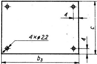
Kształt P 3
