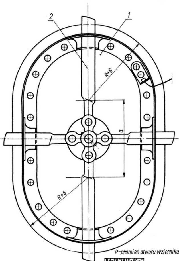
Rys. 1. Wziernik owalny
