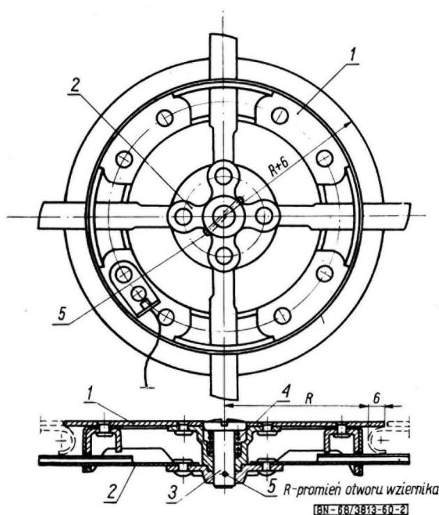
Rys. 2. Wziernik okrągły
